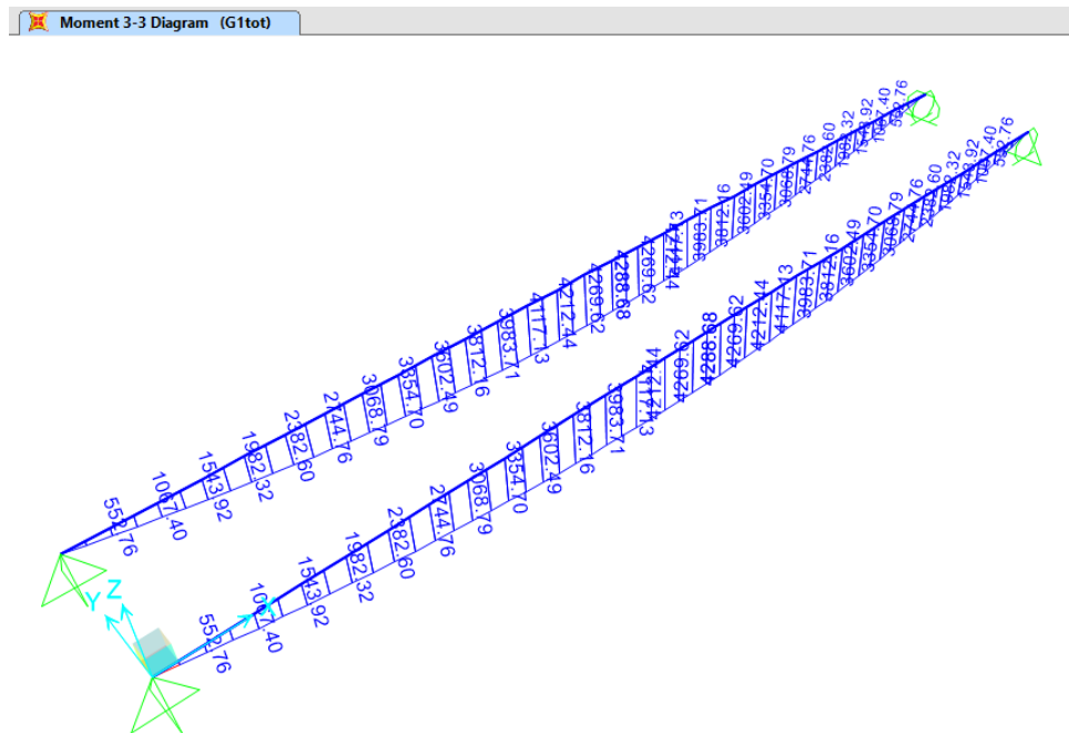
Figura 3: sollecitazione flettente per i carichi dovuti al peso proprio strutturali
