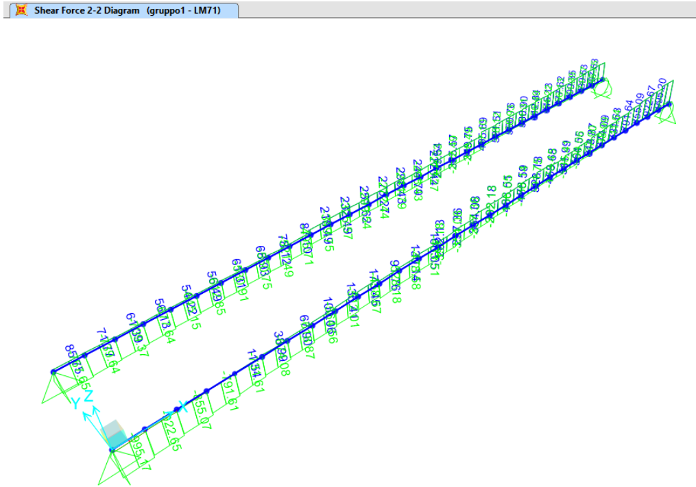
Figura 11: sollecitazione tagliante per i carichi dovuti al treno di carico LM71 - gruppo1
