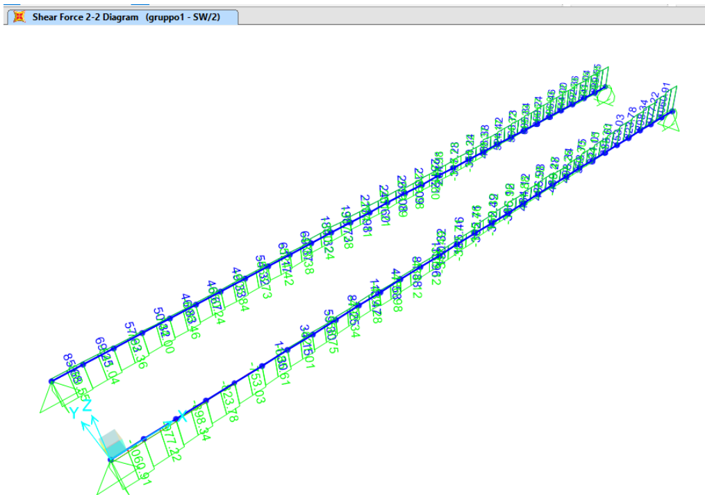
Figura 12: sollecitazione tagliante per i carichi dovuti al treno di carico SW/2 - gruppo1
