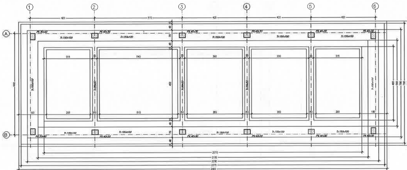
Figura 1 – Carpenteria Fondazione
