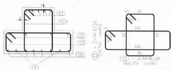
SEZIONE A-A
