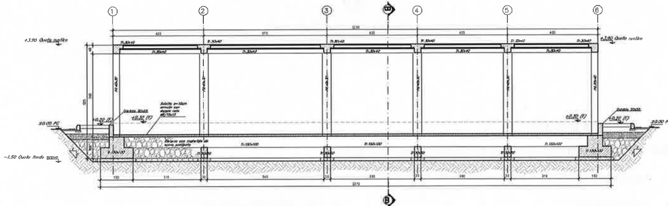
Figura 2 – Sezione Longitudinale
