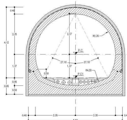
Figura - Sezione tipo di intradosso uscita di emergenza pedonale zona d'innesto
