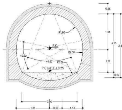
Figura - Sezione tipo di intradosso uscita di emergenza pedonale sezione corrente
