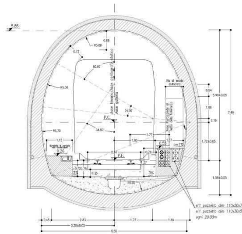
Figura - Sezione di intradosso gallerie di linea e gallerie artificiali policentriche (sezione corrente)
