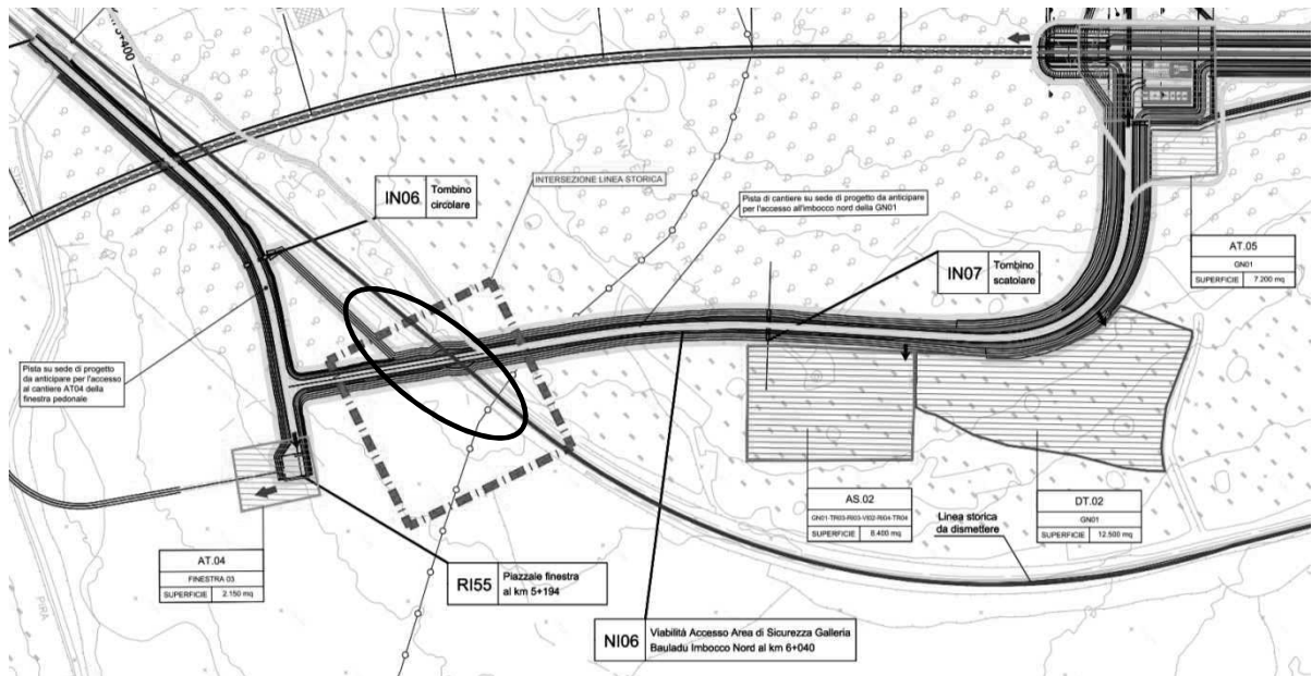
Interferenza NI06 con la LS da ultimarsi nel periodo di interruzione prolungata
