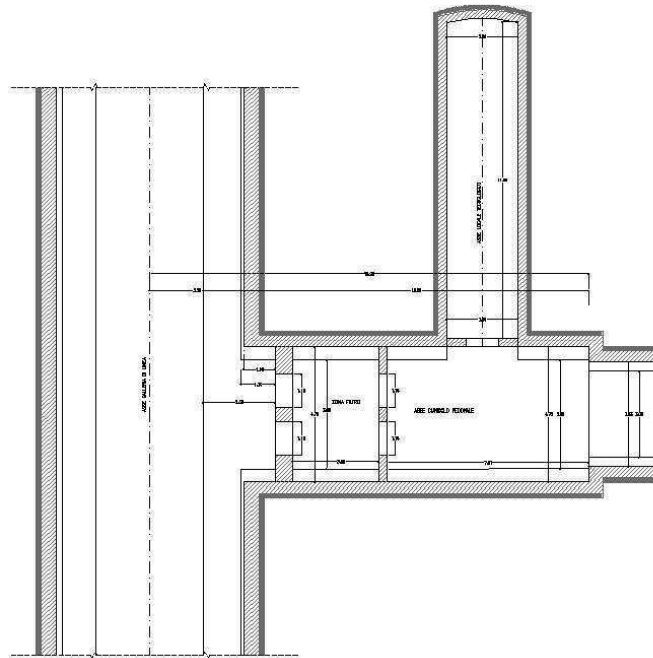
Figura - Innesto galleria di linea – cunicolo pedonale
