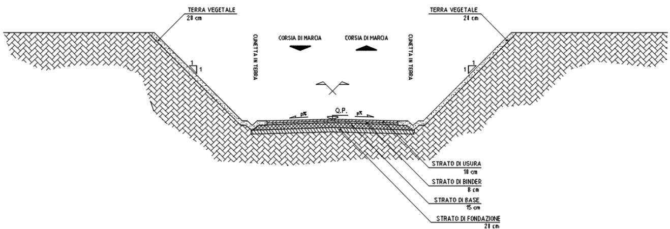
Sezione tipo in trincea
