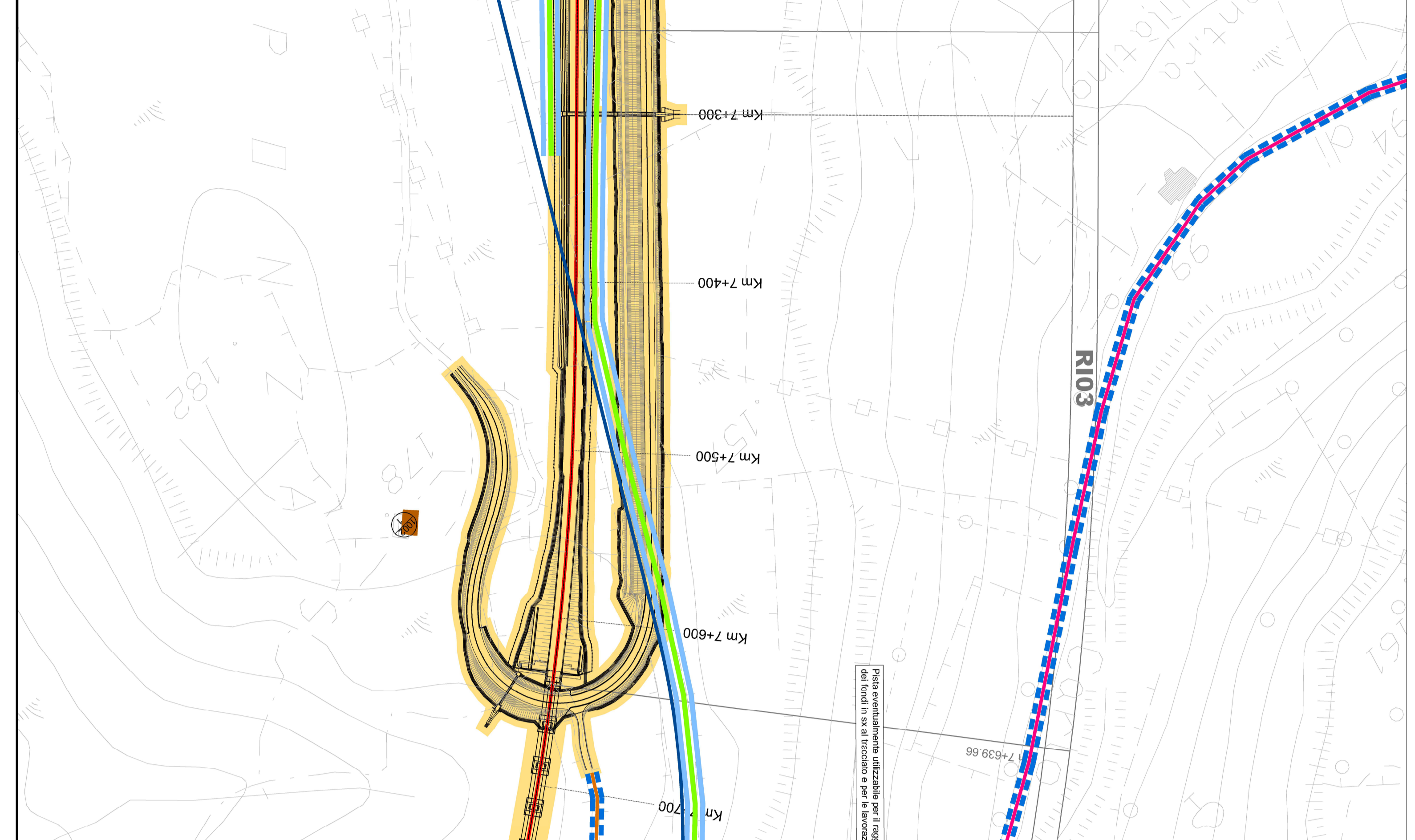
PLANIMETRIA STAZIONE DI PAULLATINO PER DEPOSITO TOLTO D'OPERA - Scala 1:2000
