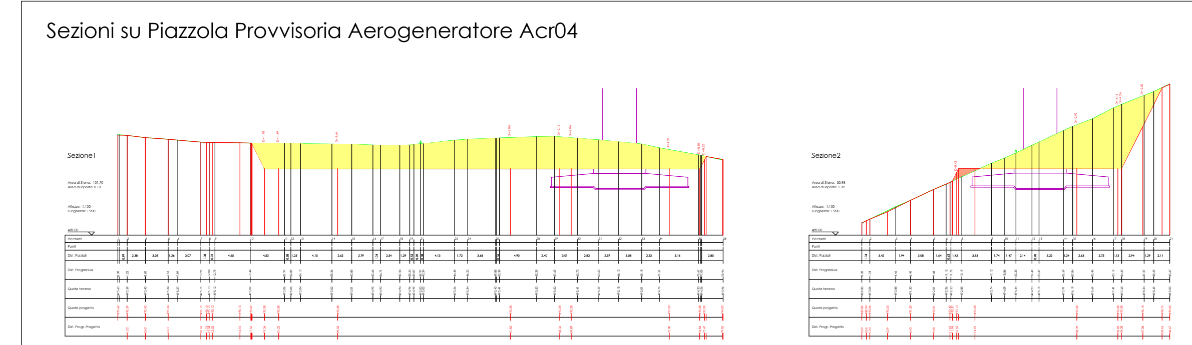
Sezioni su Piazzola Provvisoria Aerogeneratore Acr04
