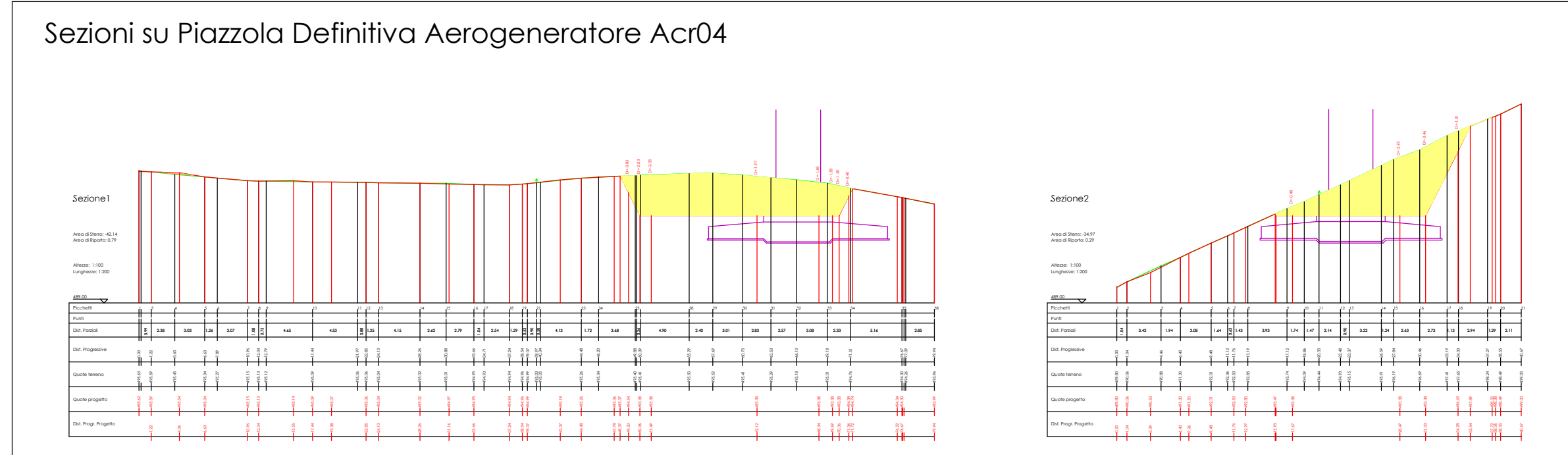
Sezioni su Piazzola Definitiva Aerogeneratore Acr04
