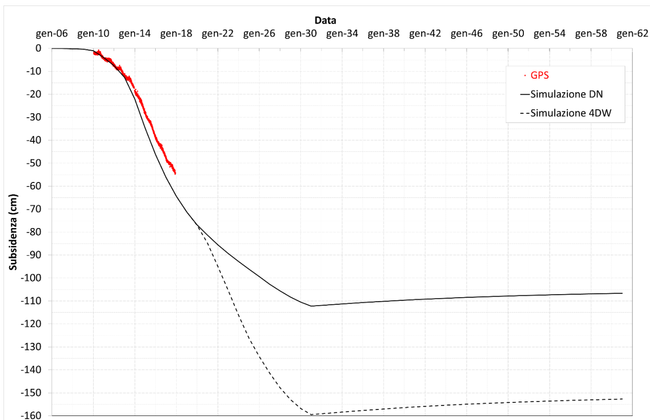
Figura 11 – Confronto tra spostamento verticale misurato e simulato alla piattaforma Annamaria A.
