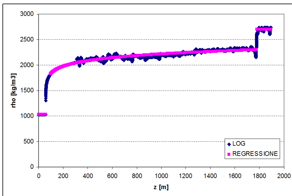
Figura 5 - Profilo del log di densità per il pozzo Annamaria 1.
