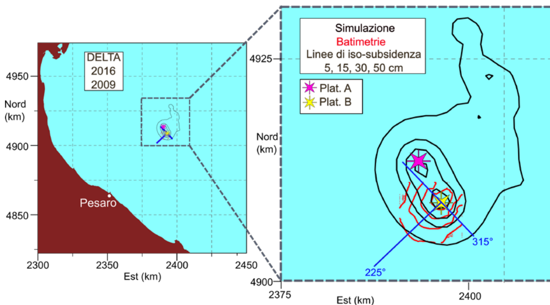
Figura 15 – Subsidenza sviluppata dal 2009 al 2016. Confronto tra misure batimetriche e stime del modello Abaqus. Sono riportate anche le tracce delle sezioni utilizzate per i confronti della Figura 16 e della Figura 17.
