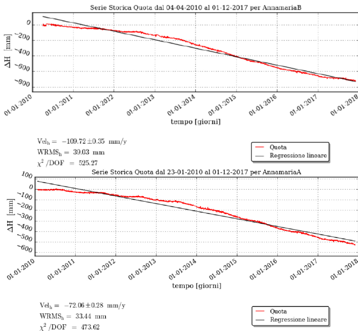
Figura 3 – Serie storiche di spostamenti verticali registrati dalle stazioni CGPS, aggiornate al giorno 01/12/2017, (in alto piattaforma B e in basso piattaforma A).
