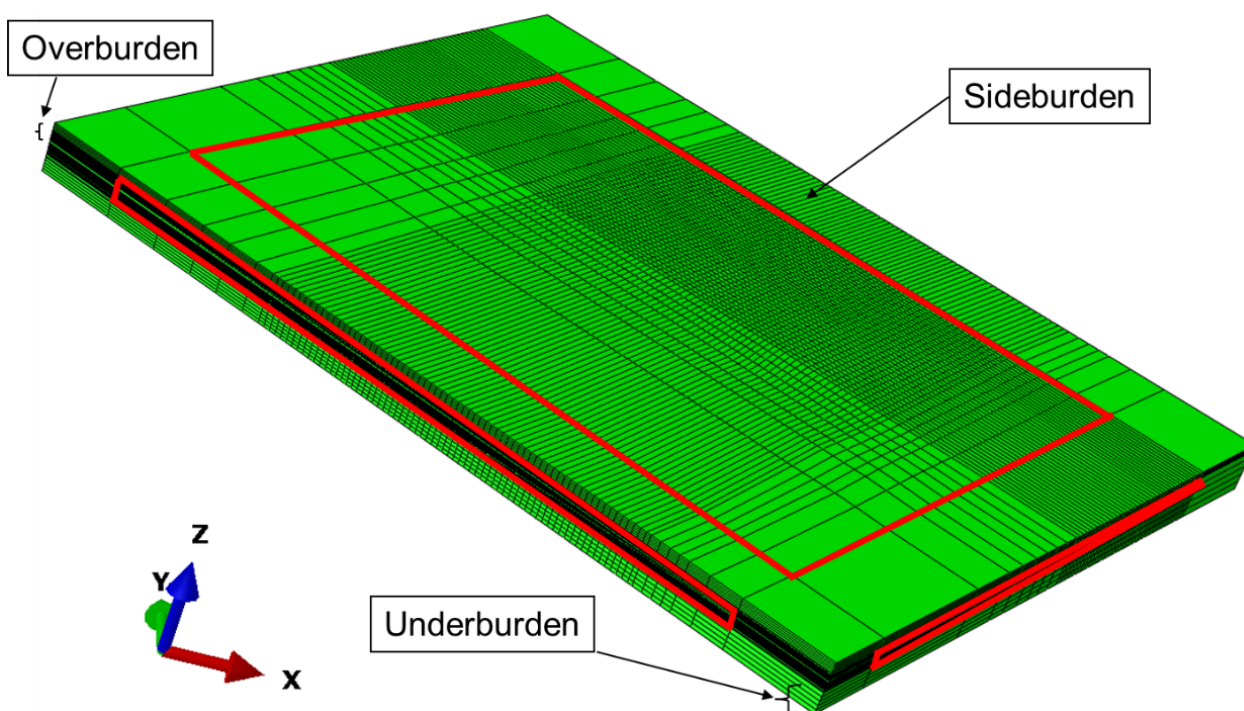
Figura 4 – Confronto tra l'estensione del modello geomeccanico e del modello fluido-dinamico (riquadri rossi).
