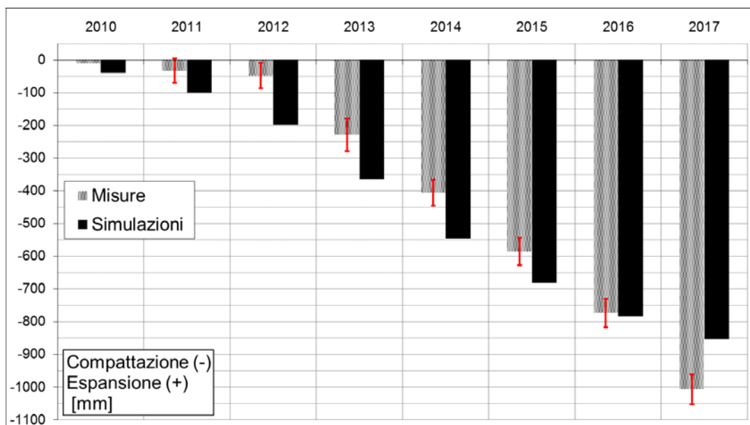
Figura 13 – Confronto tra le deformazioni verticali misurate e le corrispondenti stime del modello geomeccanico, rispetto al primo sondaggio del 2010, con riferimento all'insieme di tutti gli spacing monitorati, fatta eccezione per gli spacing numero 2, 96, 97, 98 e 99.
