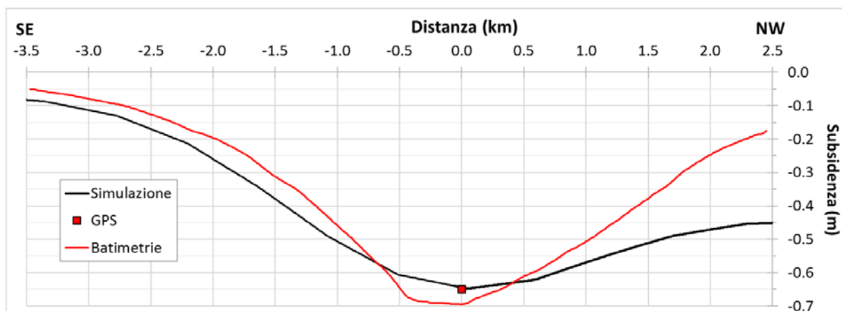
Figura 17 - Subsidenza sviluppata dal 2009 al 2016 lungo la sezione parallela alla linea mediana e avente azimut 315°. Confronto tra misure batimetriche, valori stimati dal modello Abaqus e GPS.
