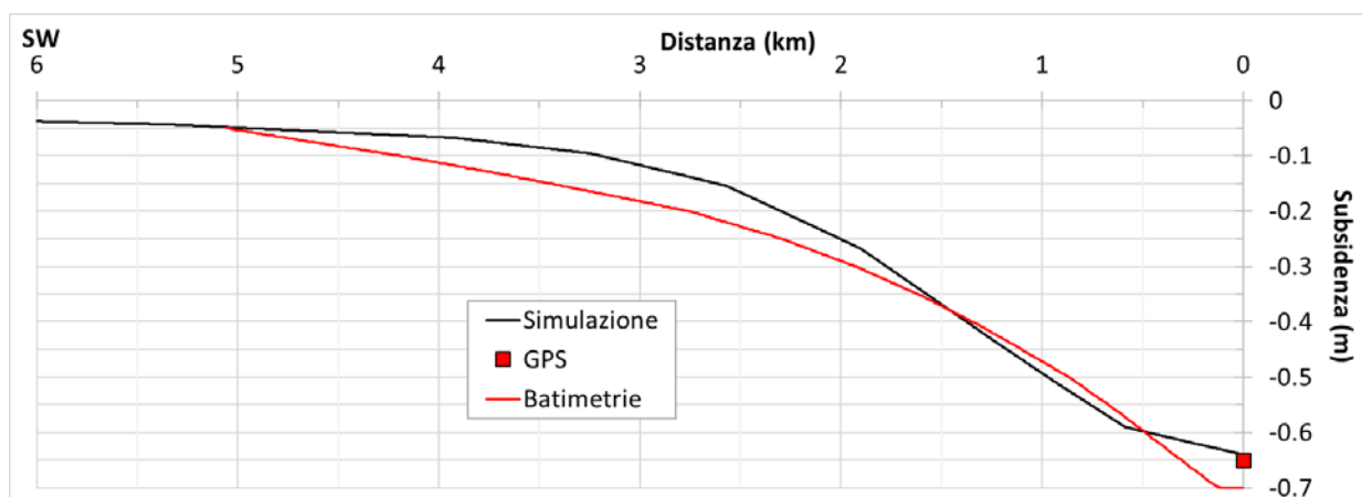
Figura 16 – Subsidenza sviluppata dal 2009 al 2016 lungo la sezione perpendicolare alla linea mediana e avente azimut 225°. Confronto tra valori stimati dal modello Abaqus, misure batimetriche e GPS.
