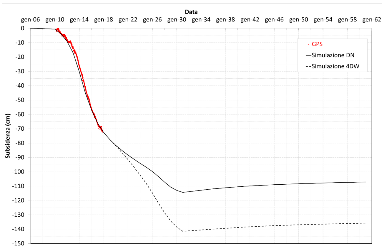
Figura 9 – Confronto tra spostamento verticale misurato e simulato alla piattaforma Annamaria B.
