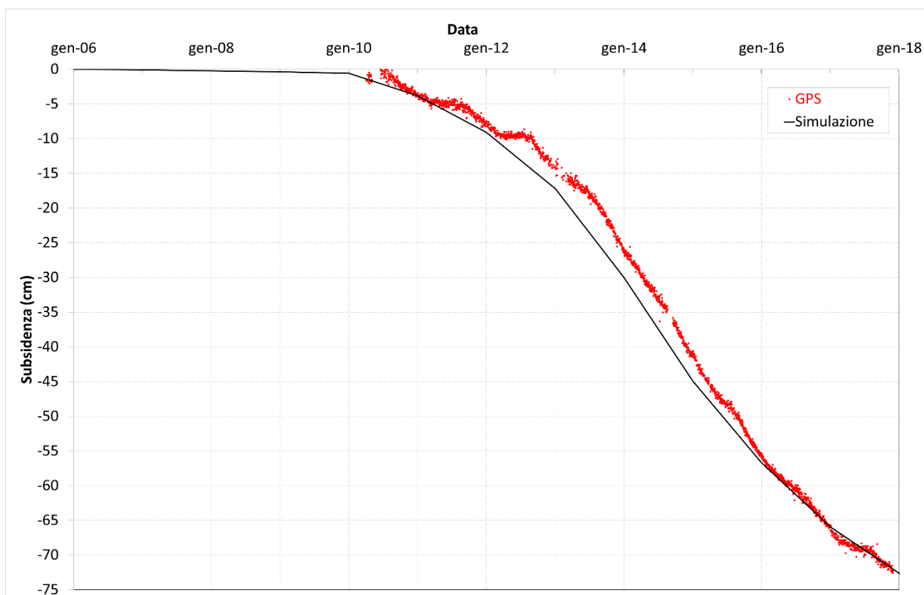
Figura 10 – Ingrandimento della Figura 9.
