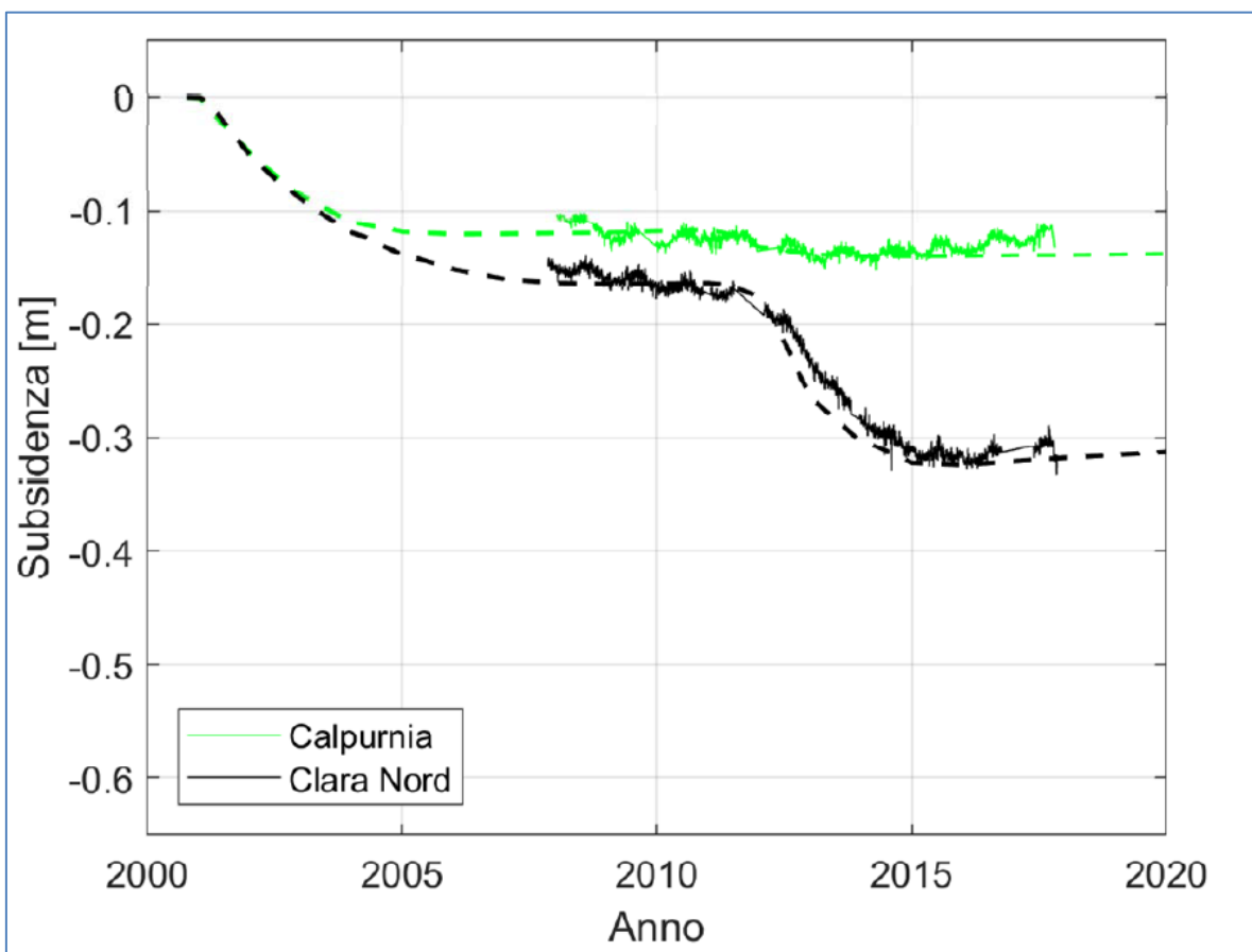
Figura 14 – Andamento della subsidenza misurata (CGPS in p.ma) comparata con la simulazione per i campi di Clara Nord e Calpurnia
