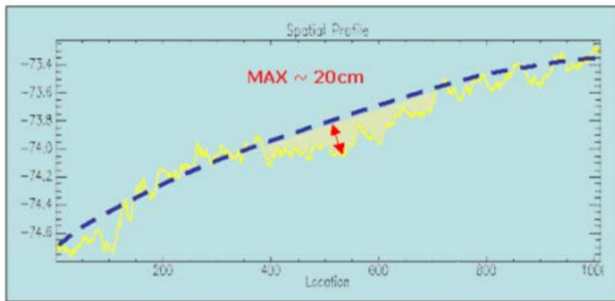
Figura 9 – Campo di Clara Nord: profilo batimetrico interpolato e differenza con la batimetria misurata
