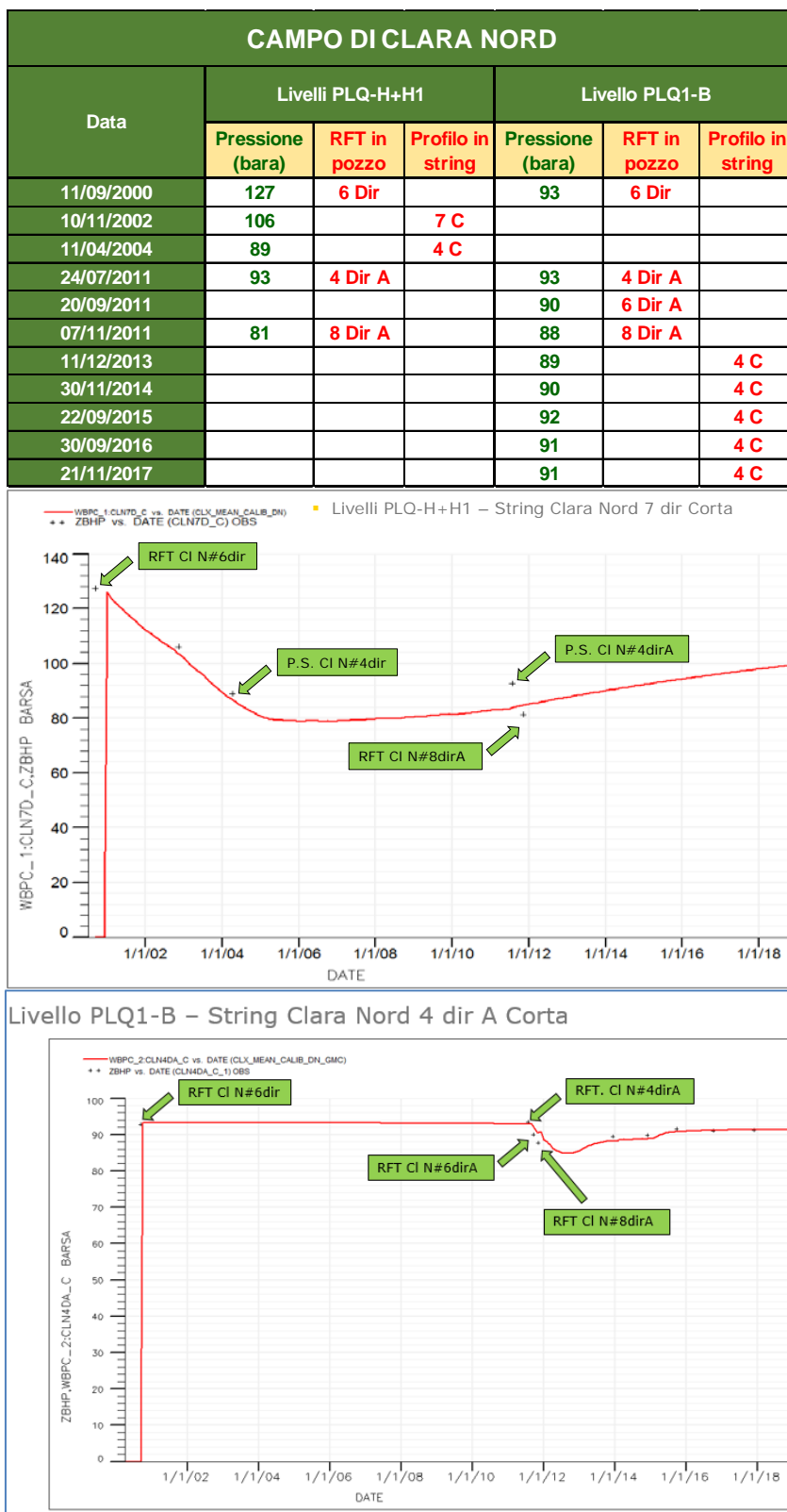
Figura 5 – Campo di Clara Nord: confronto tra dati di pressione da profili statici e modello Eclipse (livelli PLQ-HH1 e PLQ1-B)
