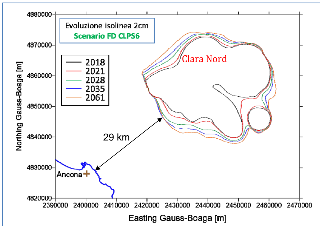
Figura 6 – Evoluzione nel tempo della linea dei -2 cm per lo scenario CLPS6
