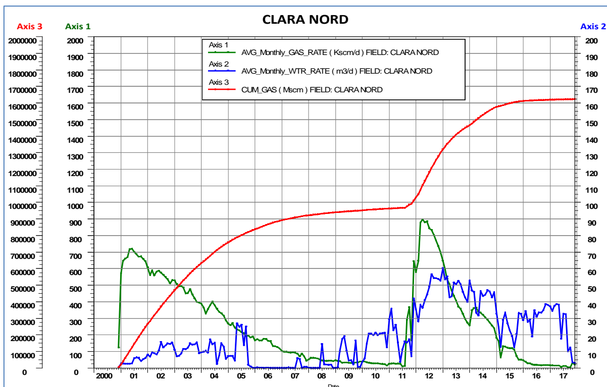
Figura 4 – Campo di Clara Nord: grafico di produzione storica
