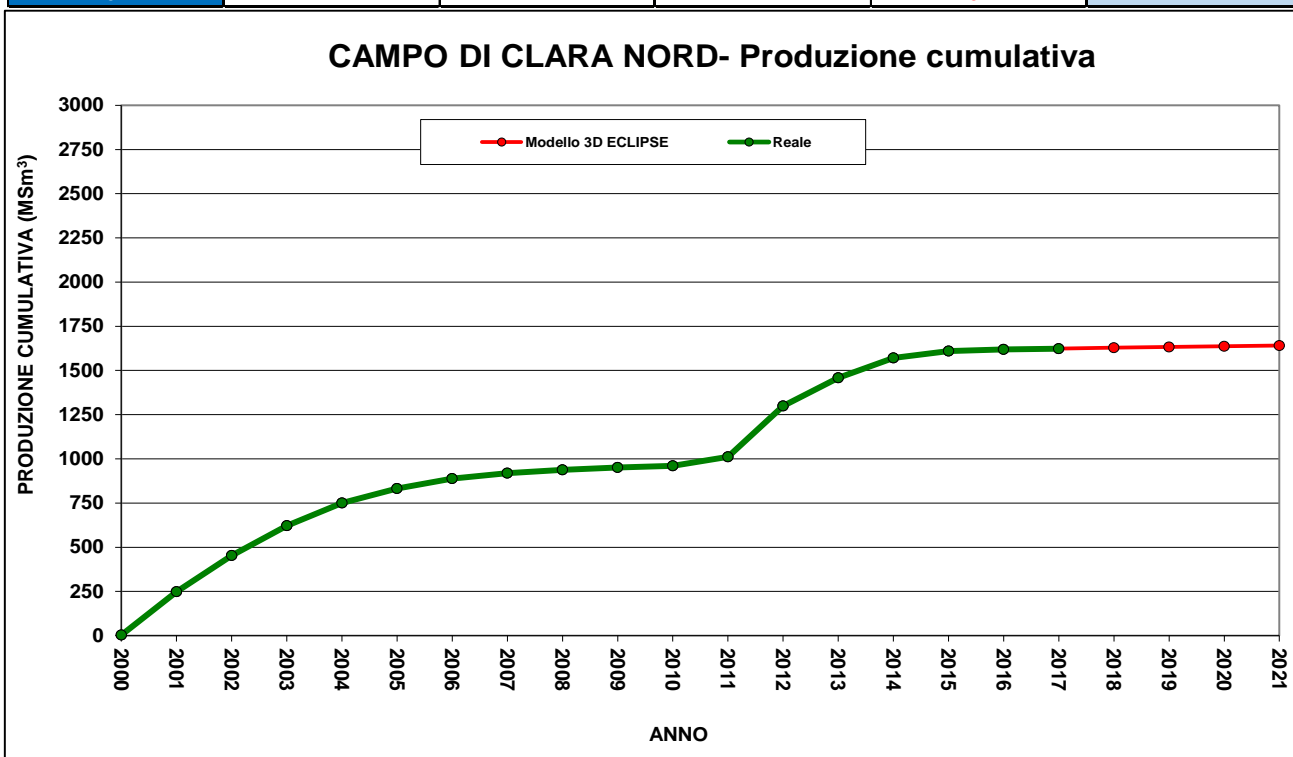
Figura 3a – Campo di Clara Nord: tabelle e grafici di produzione vs. modello Eclipse (dicembre 2017)
