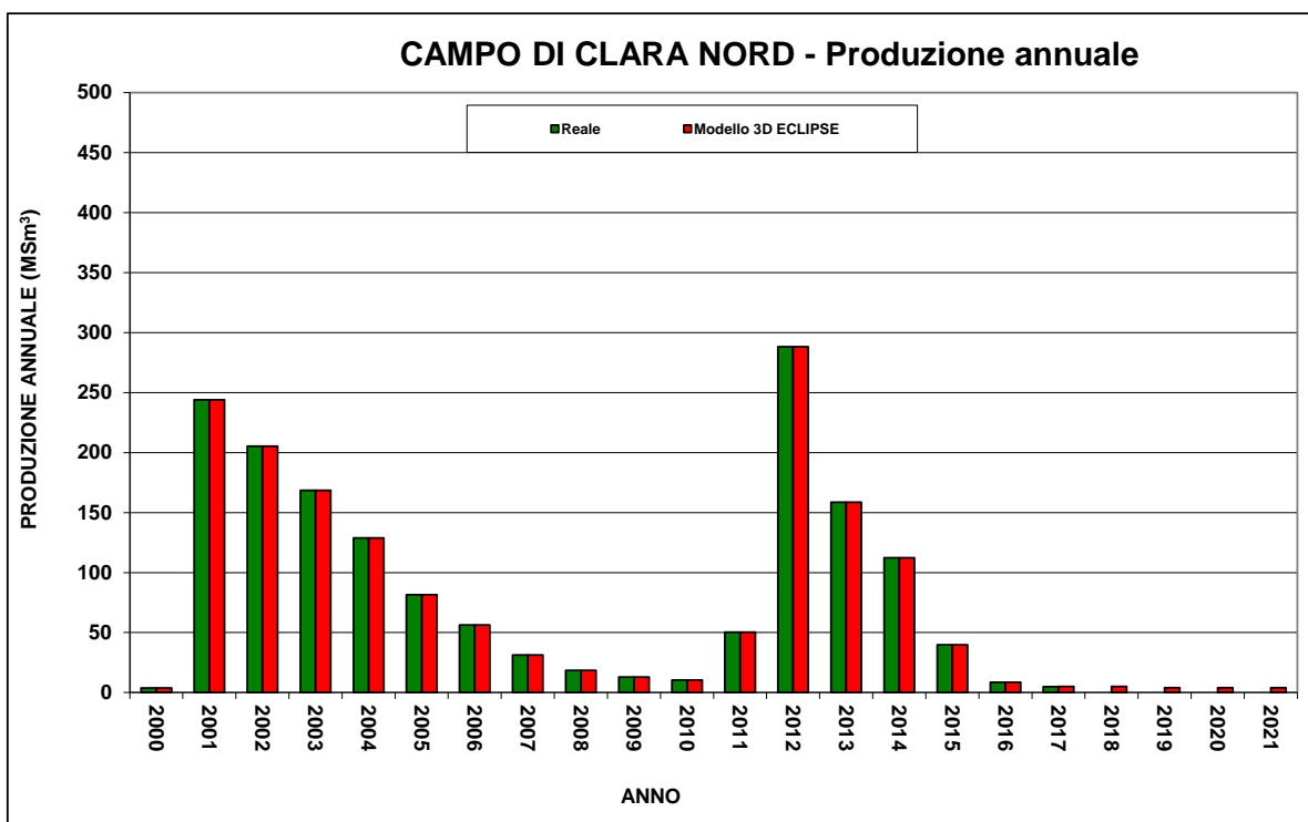
Figura 3b – Campo di Clara Nord: tabelle e grafici di produzione vs. modello Eclipse (dicembre 2017)
