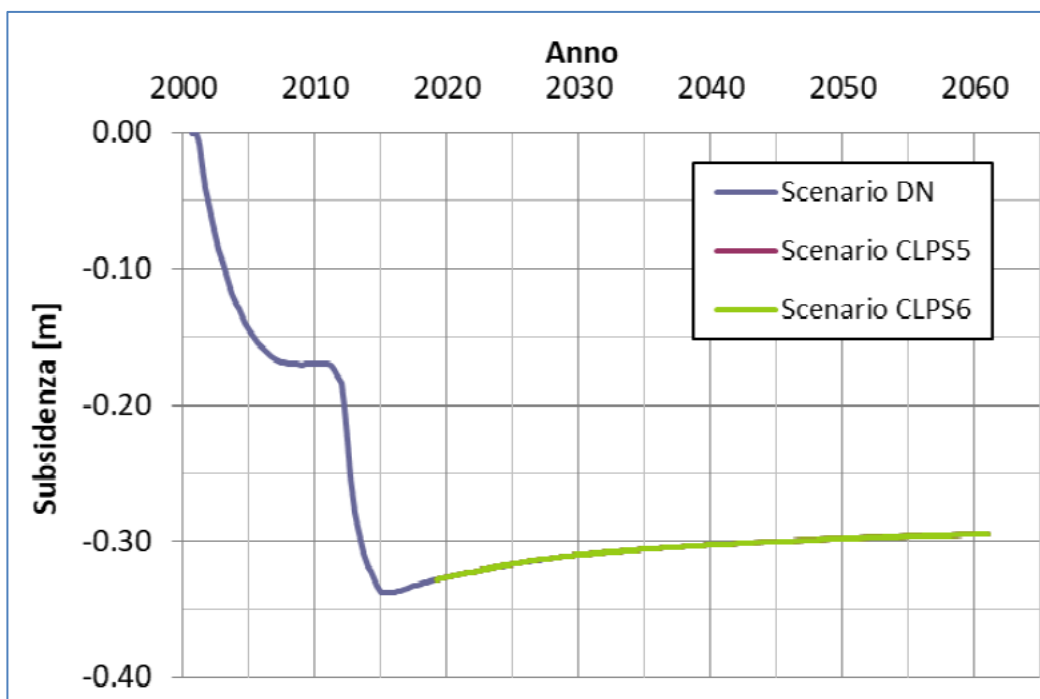
Figura 7 – Evoluzione temporale della subsidenza prevista nel punto di massimo di Clara Nord
