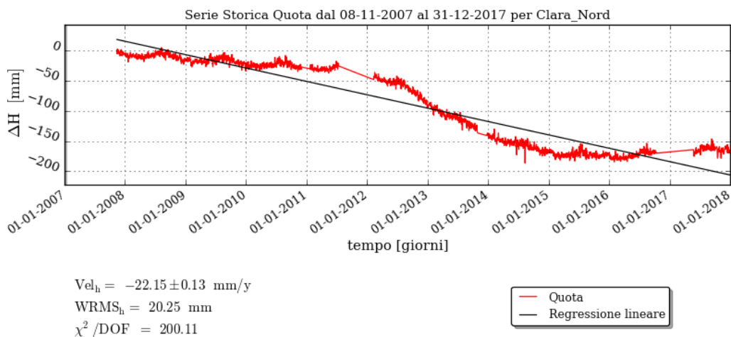
Figura 11 – Campo di Clara Nord: serie storica di misure CGPS
