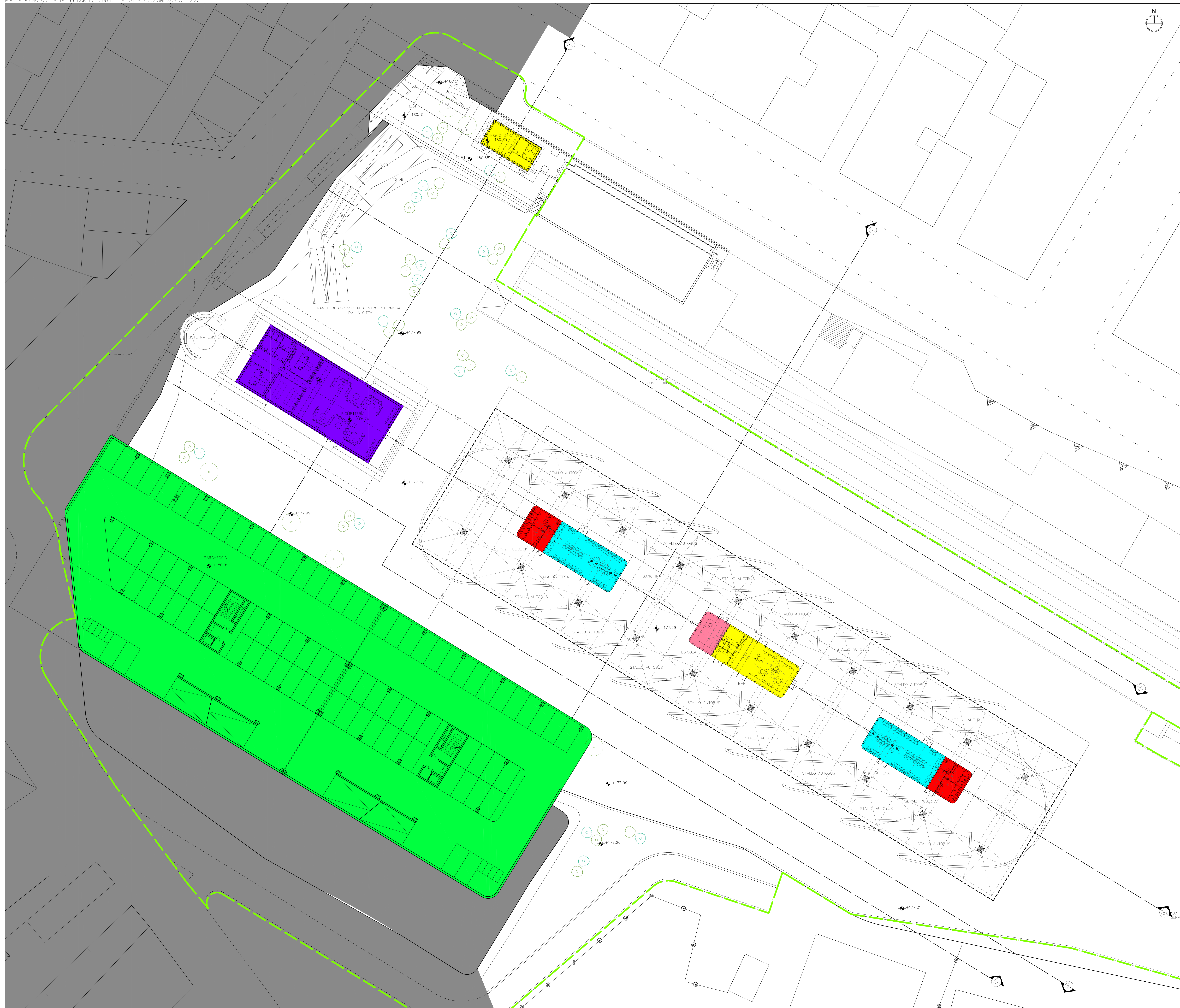
STRALCIO PIANO PARCHEGGIO A QUOTA 177.99 SCALA 1:200
