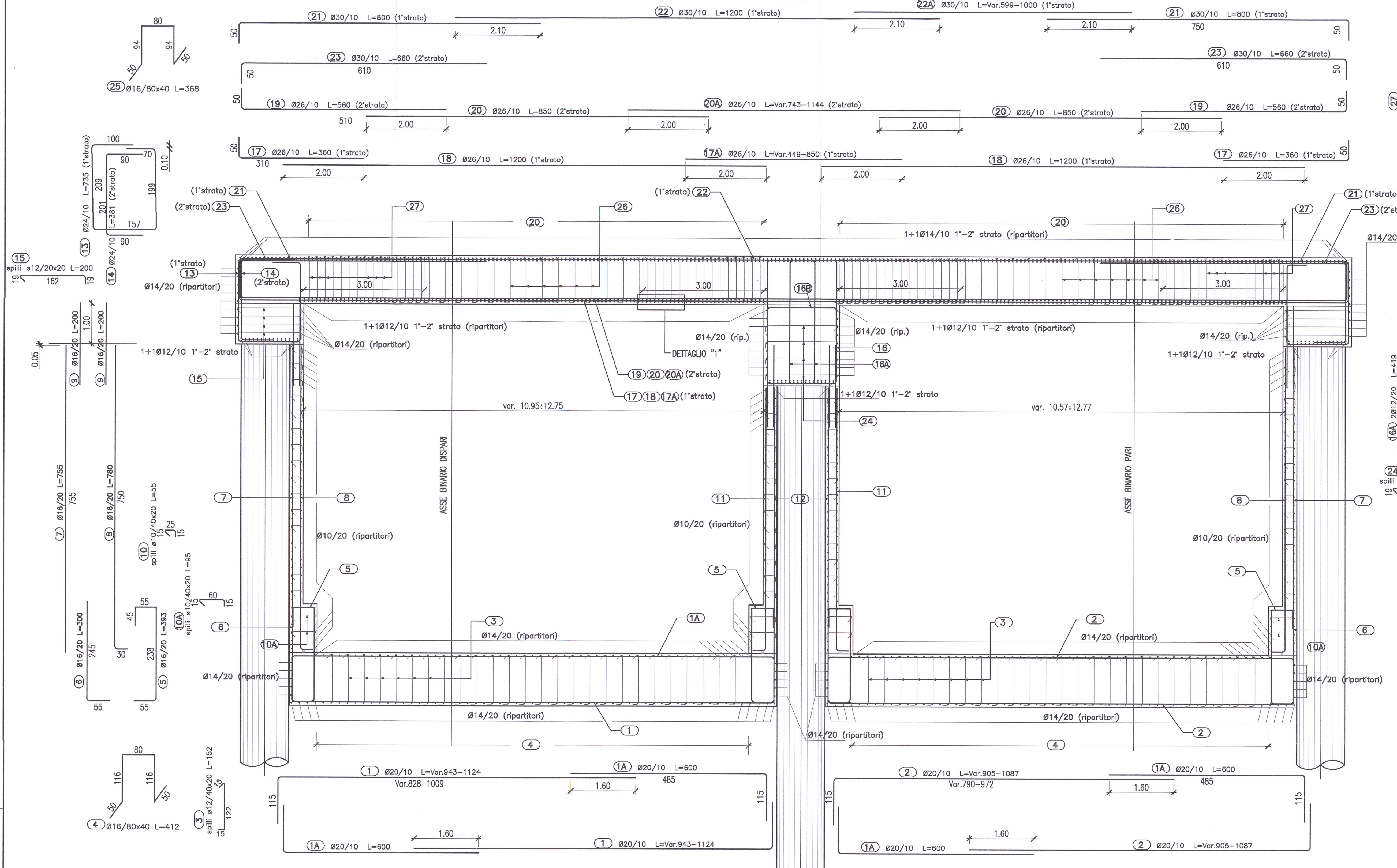
SEZIONE TIPO M3 CONCI dal 32 al 39 SCALA 1:50
