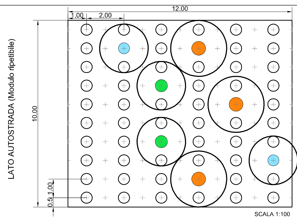
PLANIMETRIA DEL MODULO DI IMPIANTO (10x12) m = 120 mq
