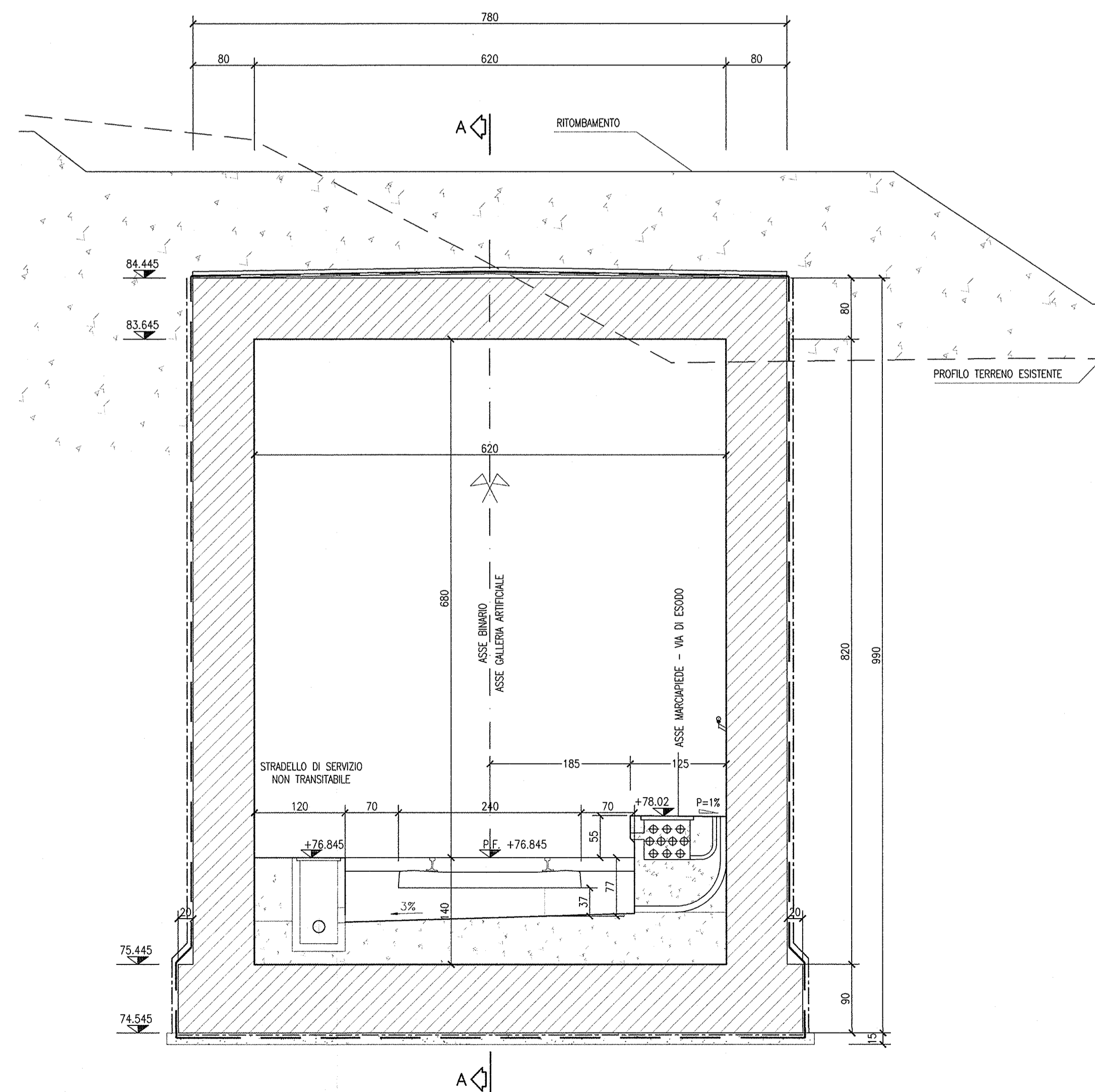
SEZIONE TRASVERSALE B-B SCALA 1:50
