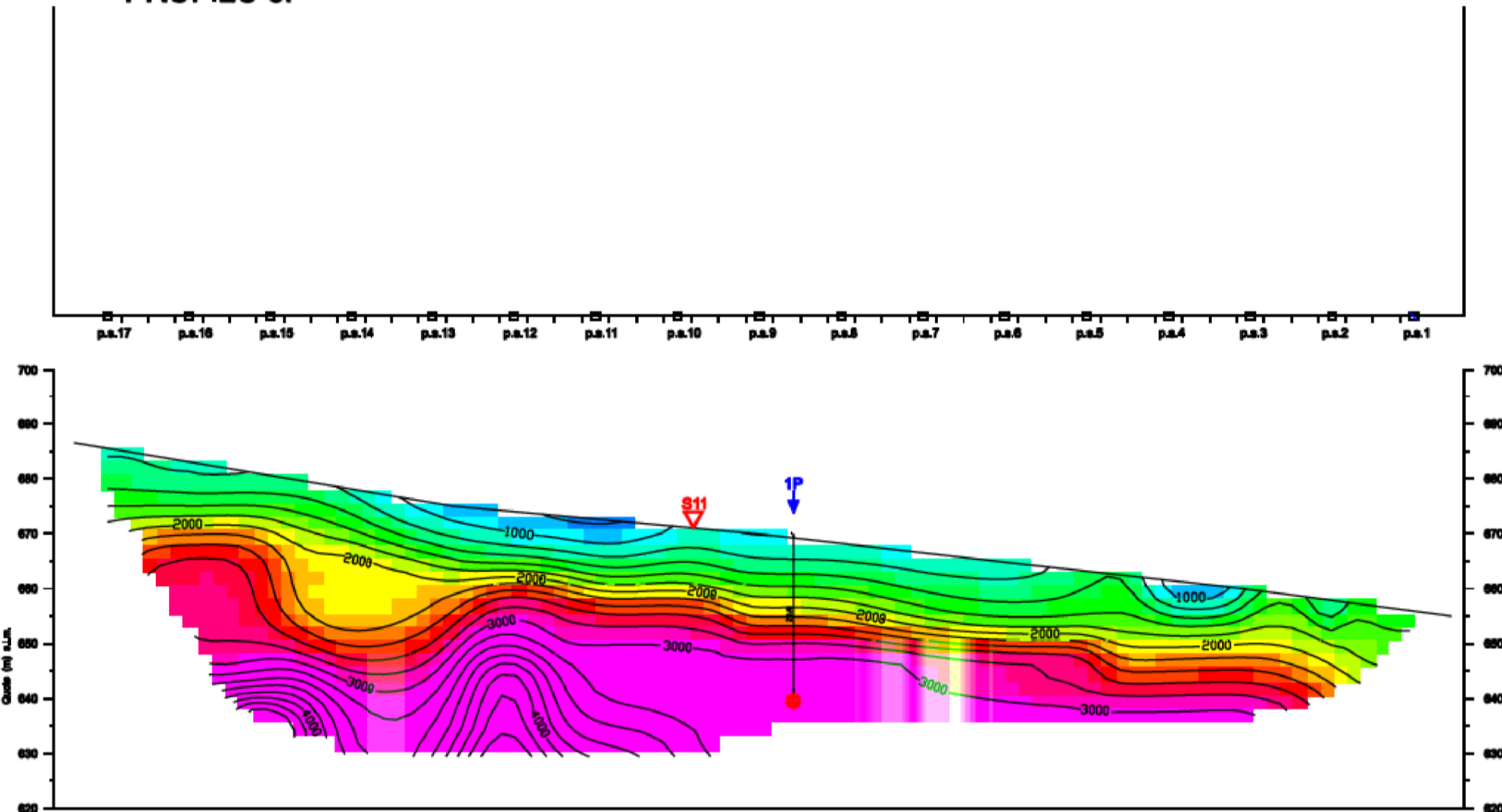
PROFILO 3P
