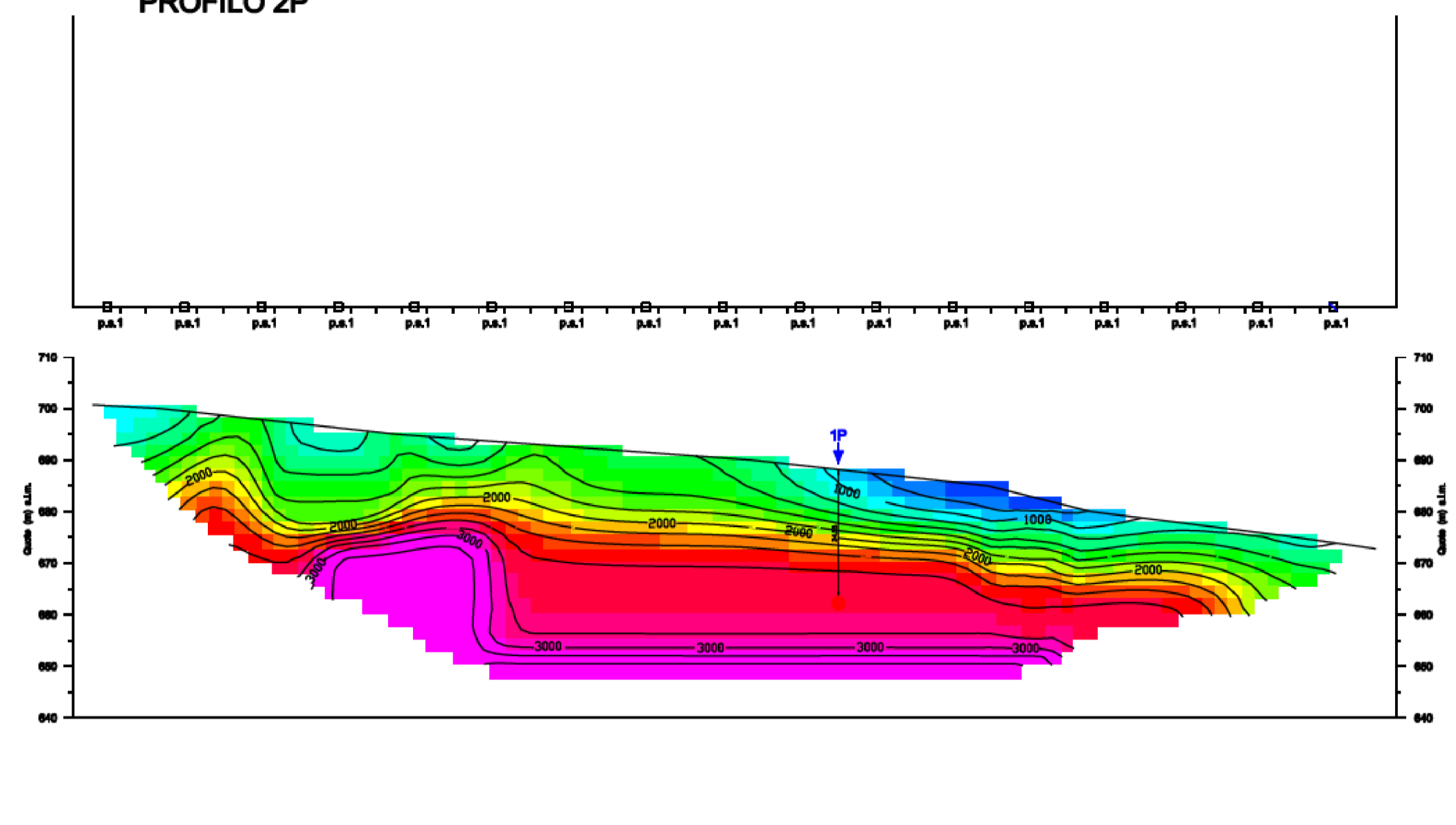
PROFILO 2P
