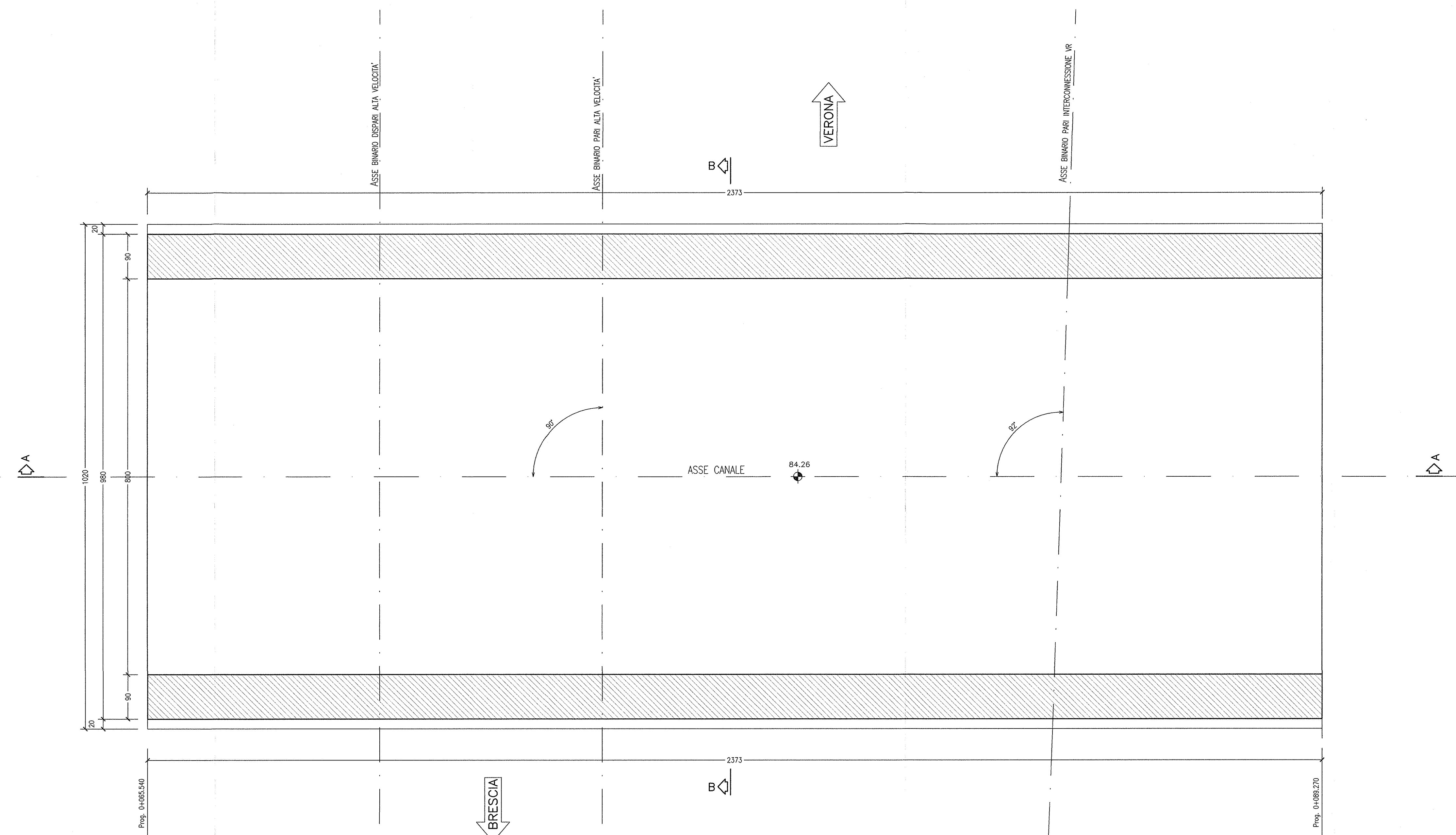
PIANTA FONDAZIONI scala 1:50
