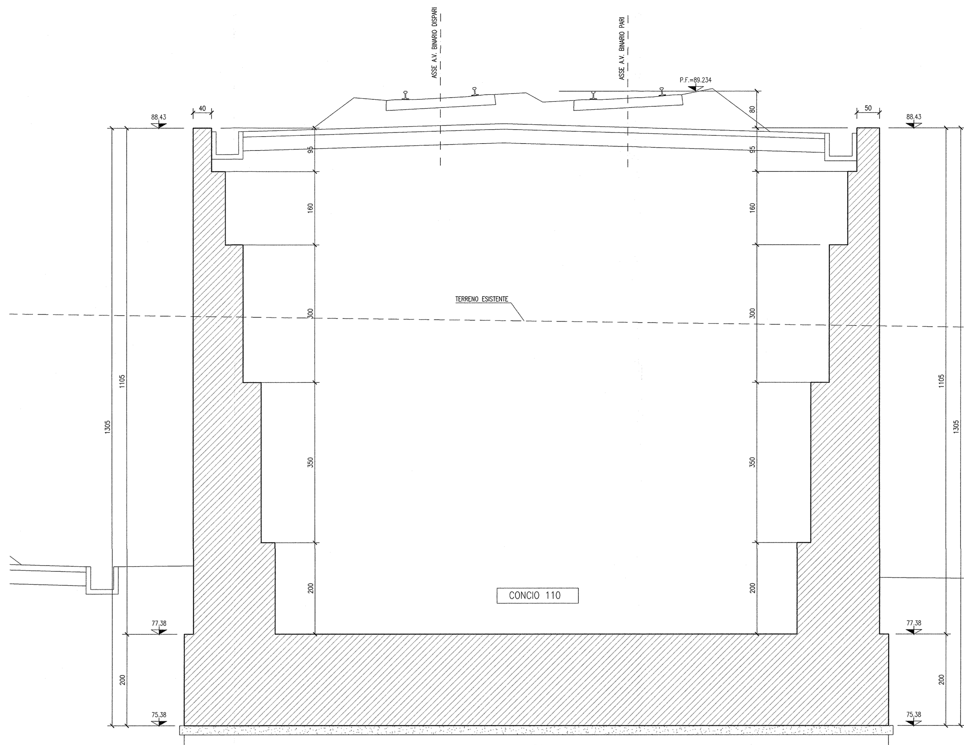
SEZIONE 44-44 SCALA 1:50
