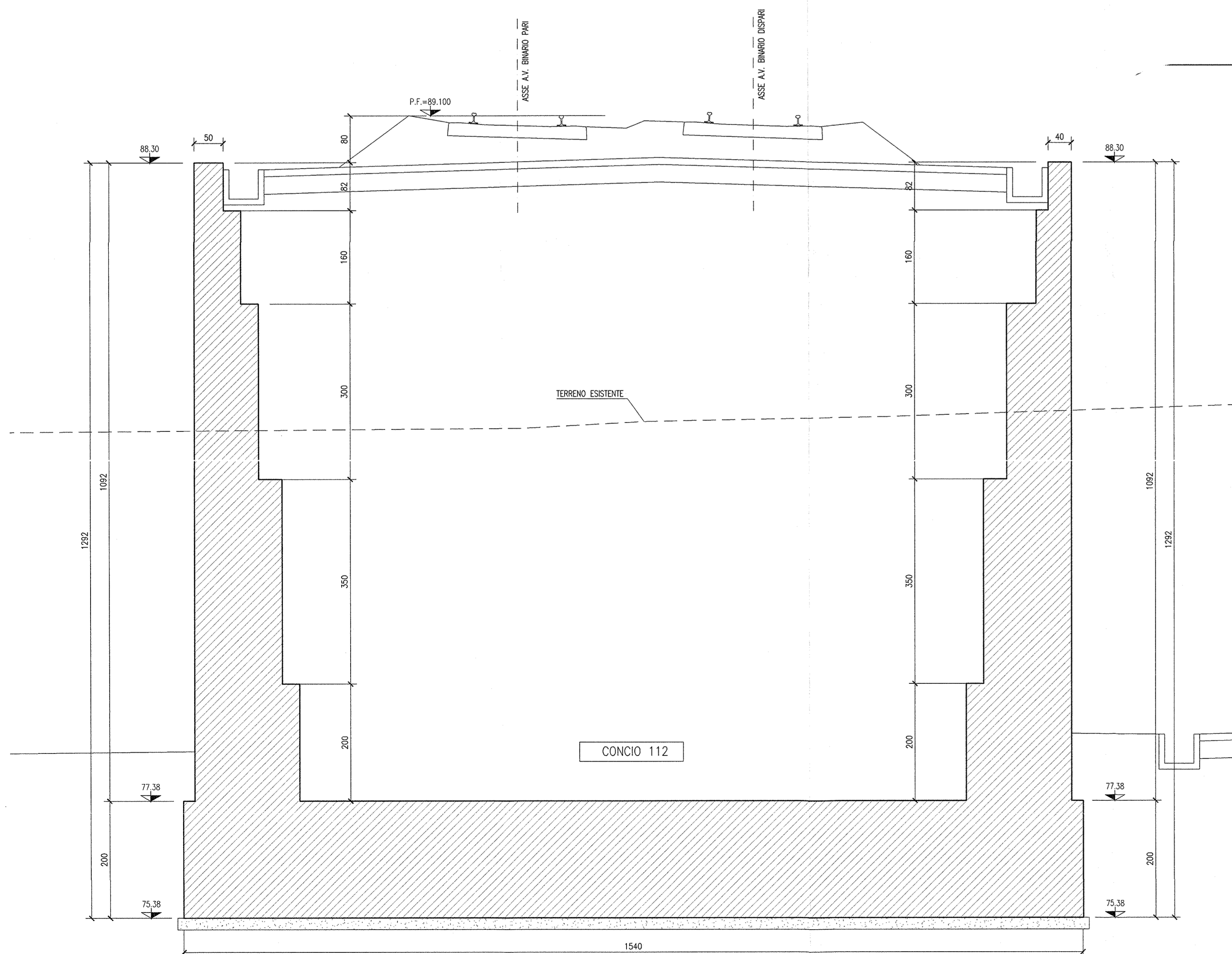
SEZIONE 45-45 SCALA 1:50
