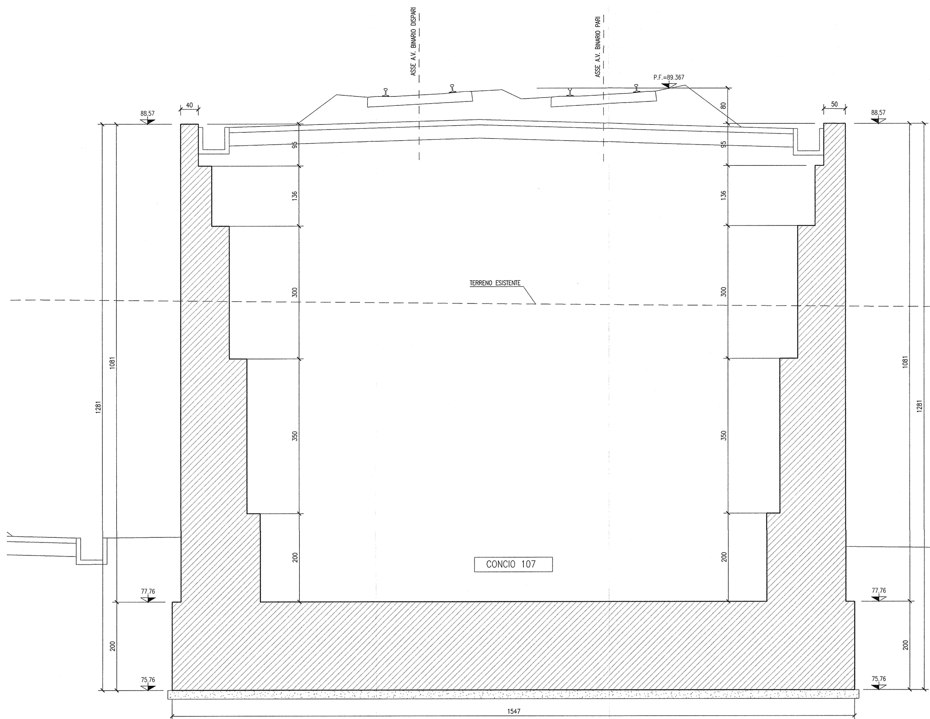
SEZIONE 43-43 SCALA 1:50
