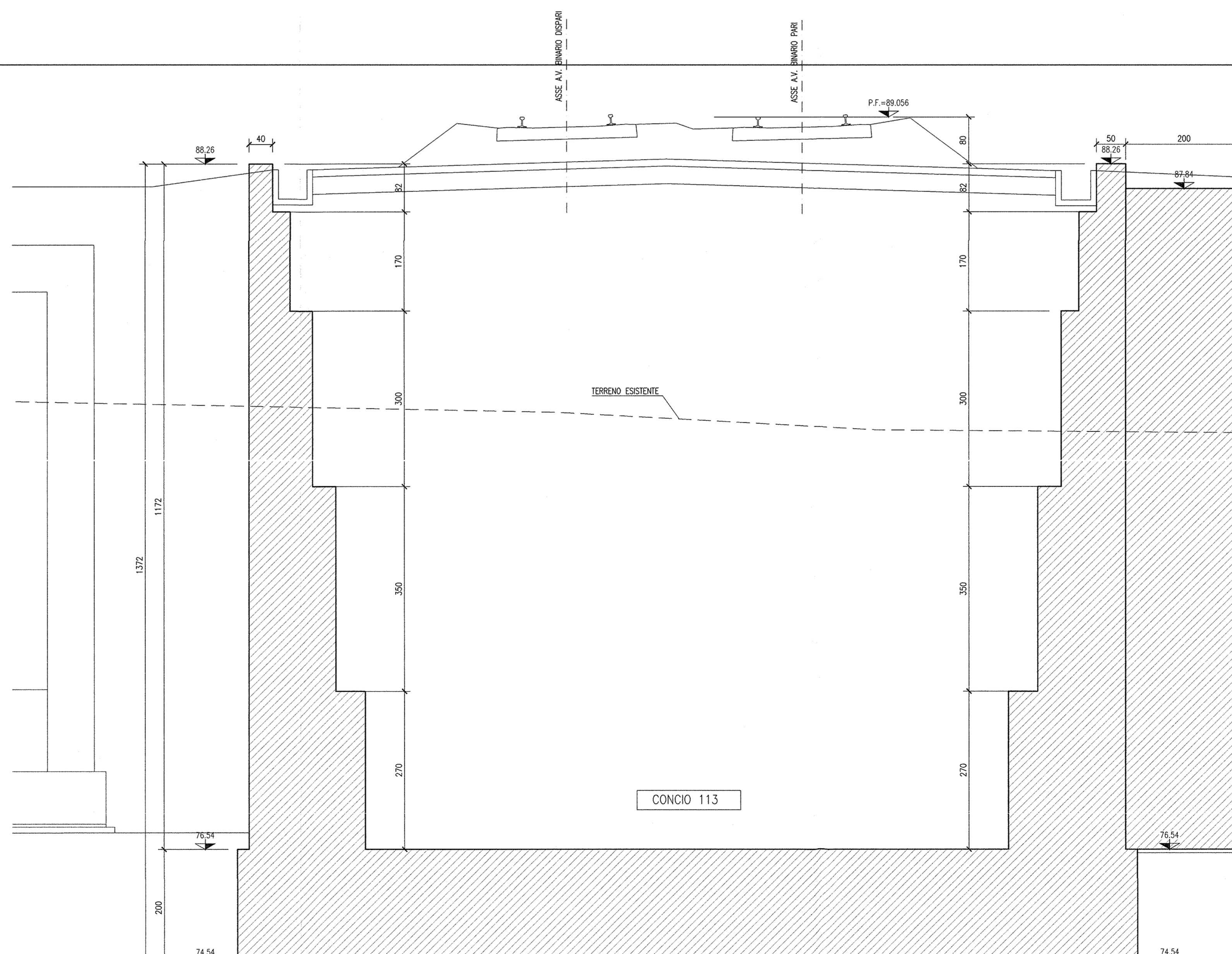
SEZIONE 46-46 SCALA 1:50
