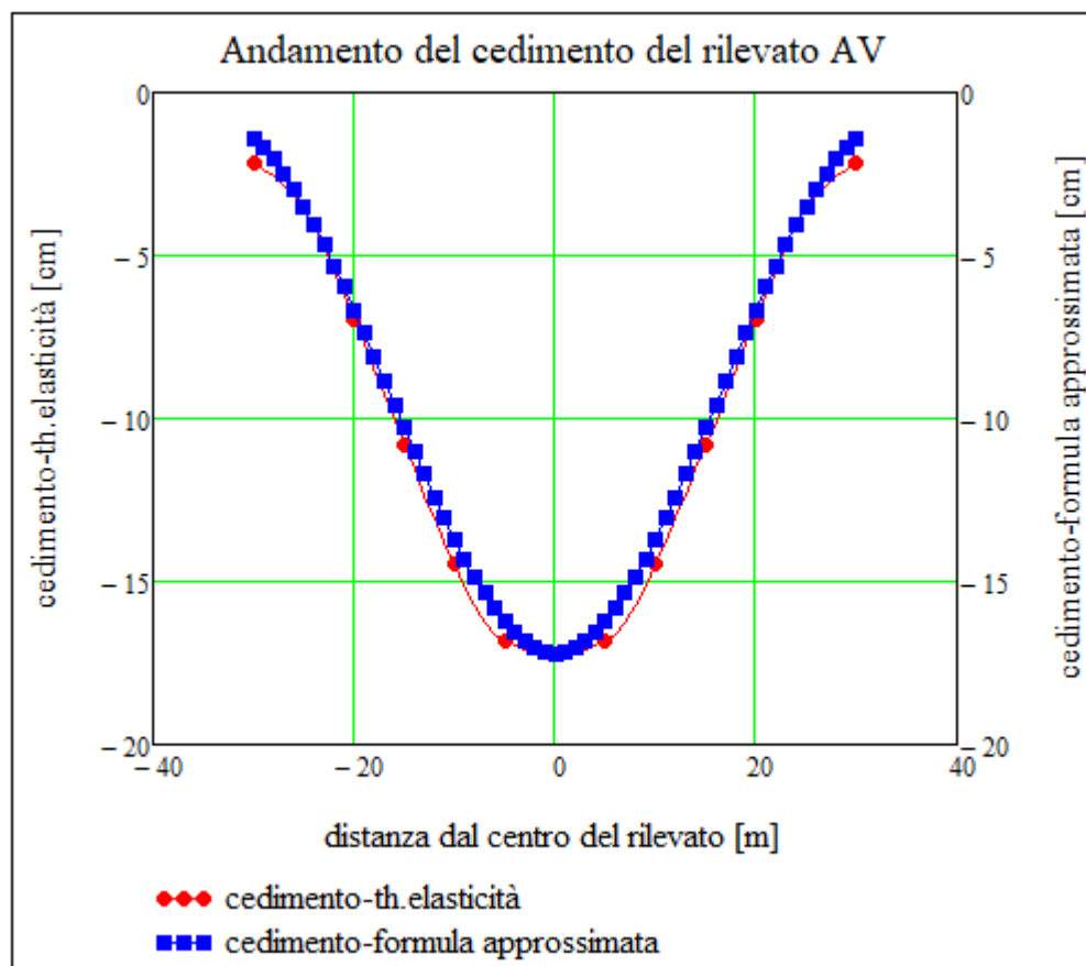
Figura 15-6: Andamento del cedimento del rilevato AV, confronto tra la soluzione elastica e quella approssimata.
