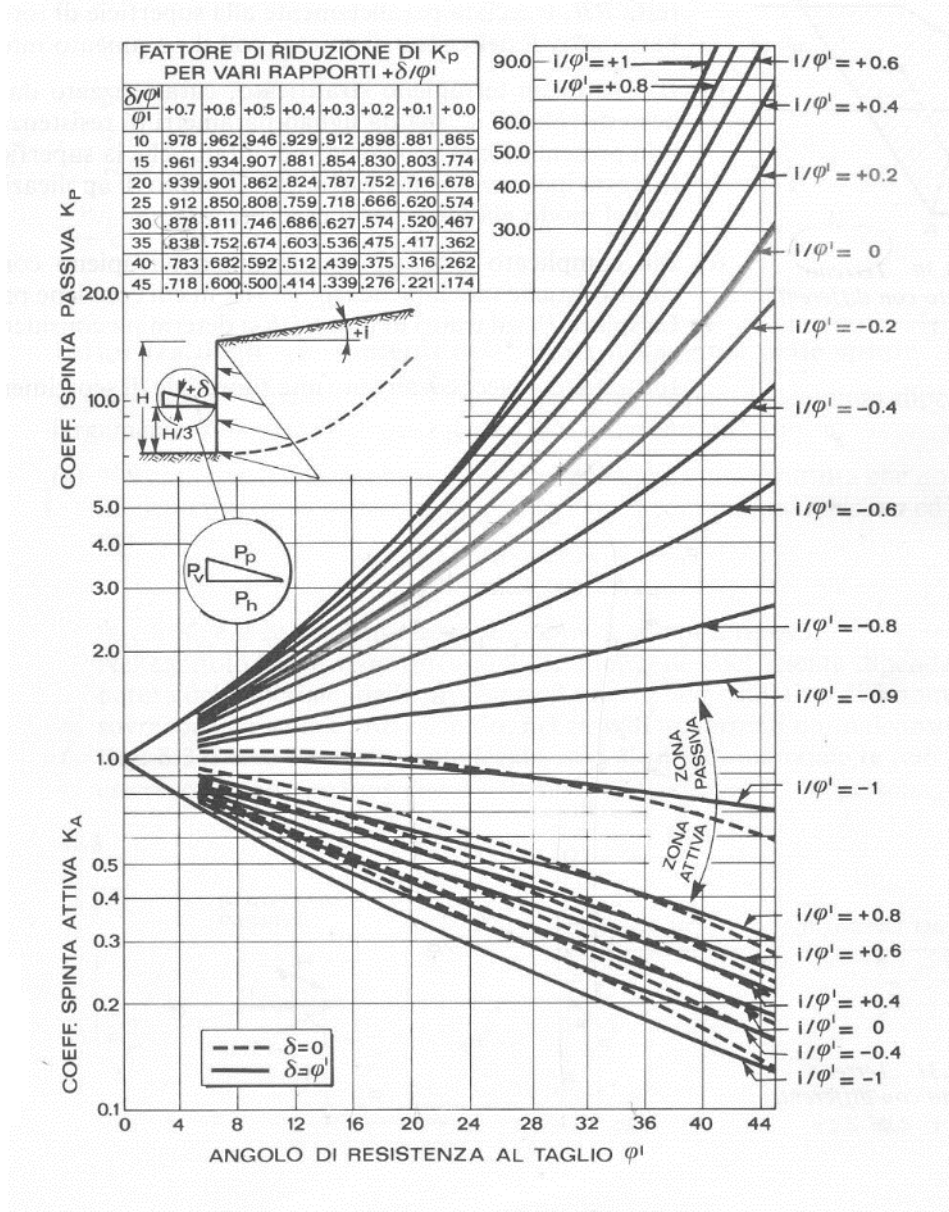
Figura 15-8: abaco per il calcolo di K_A e K_P (condizioni statiche)
