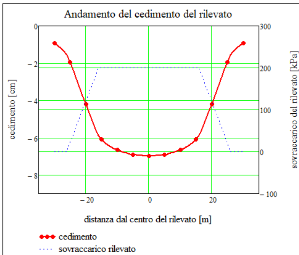
Figura 12-2: Cedimenti Rilevato RI61 (TEORIA DELL'ELASTICITÀ).
