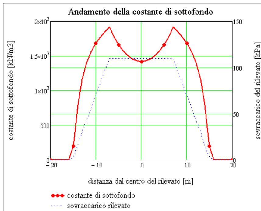
Figura 15-4: Andamento della costante di sottofondo kw.
