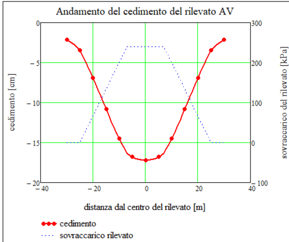
Figura 15-5: Andamento del cedimento del rilevato AV.
