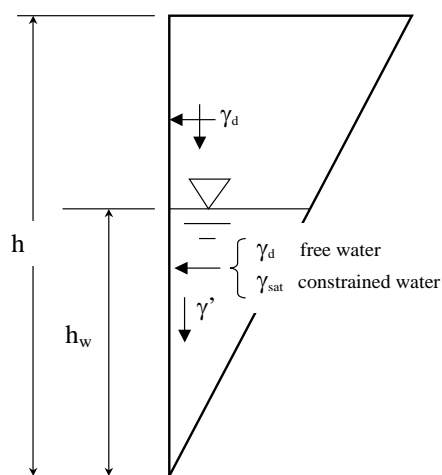
Figura 15-9: terrapieno parzialmente immerso.
