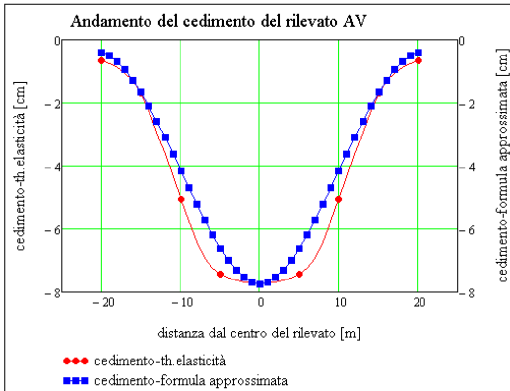
Figura 15-3: Andamento del cedimento del rilevato AV, confronto tra la soluzione elastica e quella approssimata.
