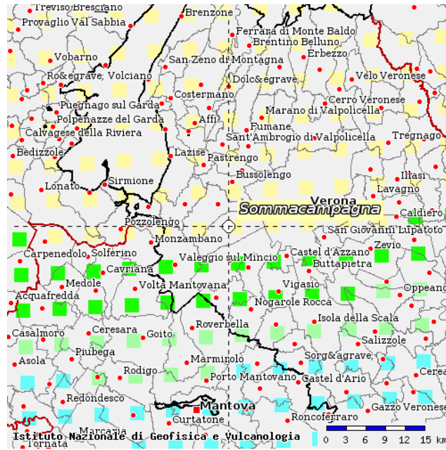
Figura 11-1: estratto mappa sismica INGV (Comune di Sommacampagna)
