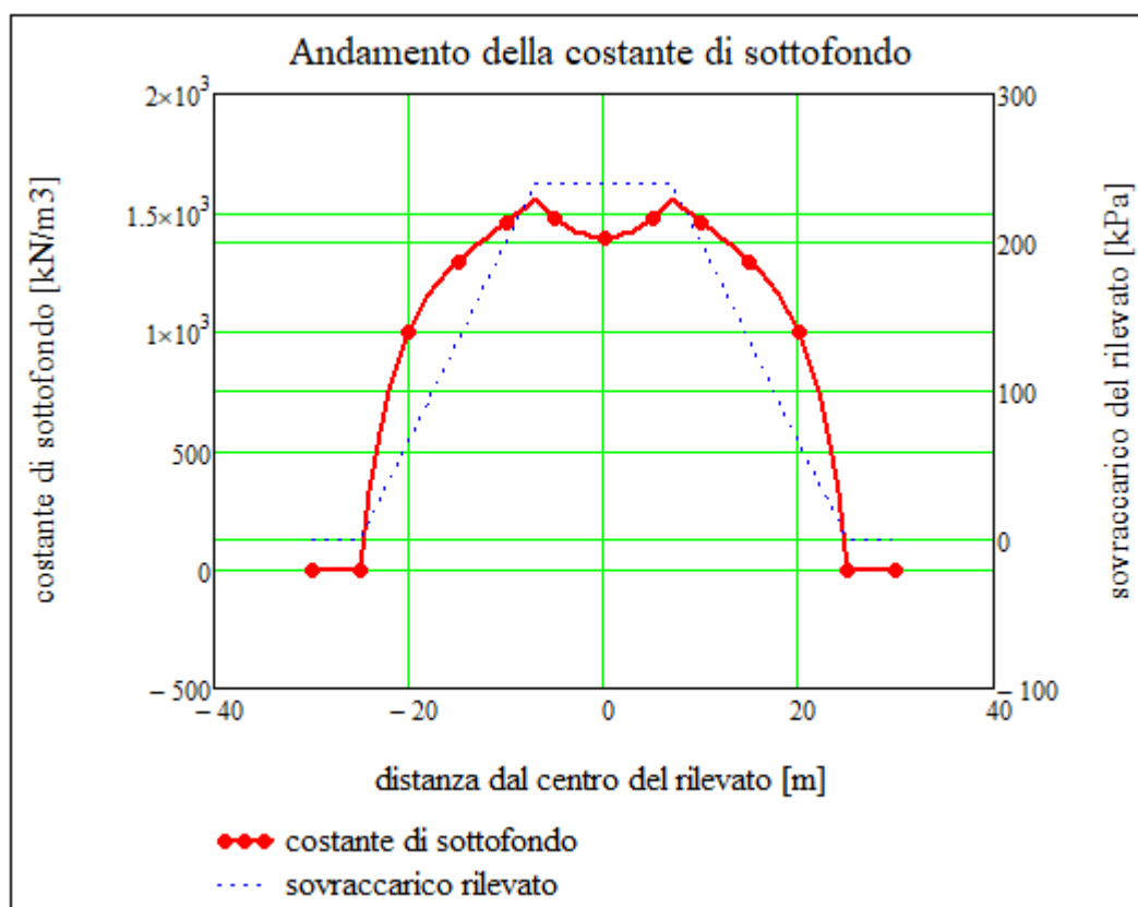
Figura 15-7: Andamento della costante di sottofondo kw.
