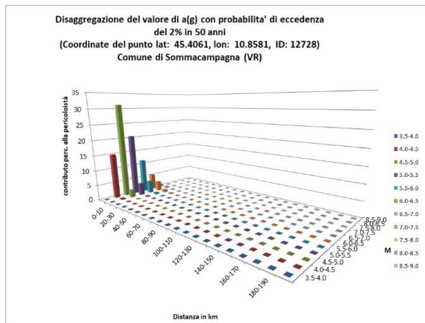
Figura 11-3: Contributi specifici magnitudo-distanza alla pericolosità sismica (Comune di Sommacampagna)
