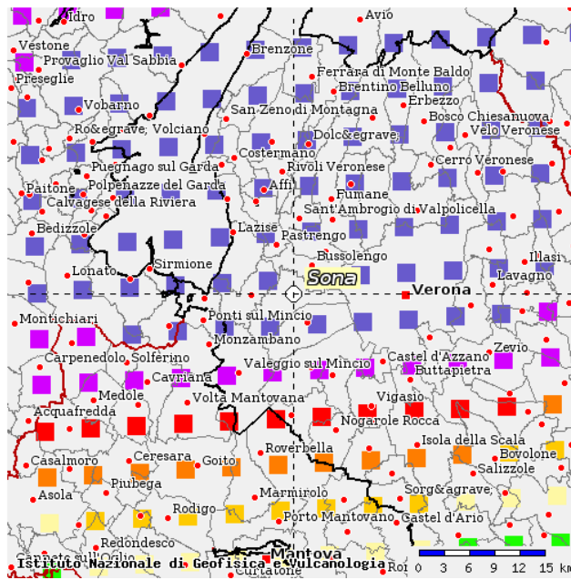
Figura 11-2: estratto mappa sismica INGV (Comune di Sona)
