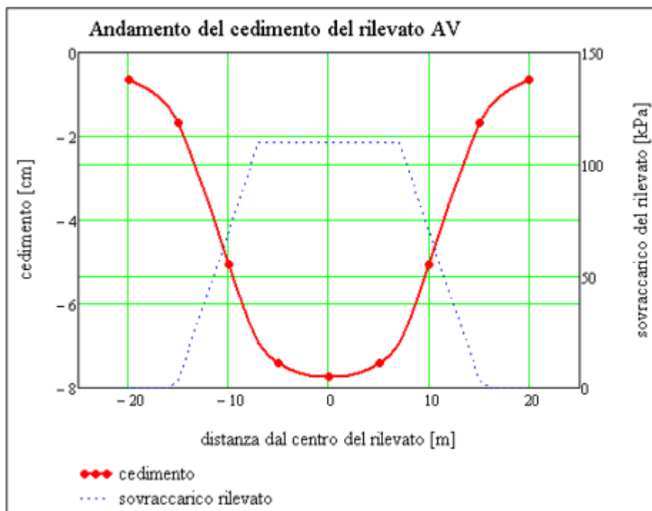
Figura 15-2: Andamento del cedimento del rilevato AV
