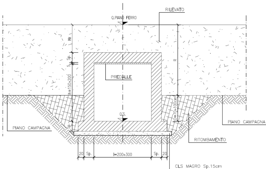
Figura 15-1: Sezione di riferimento dei tombini sottostanti il rilevato ferroviario.
