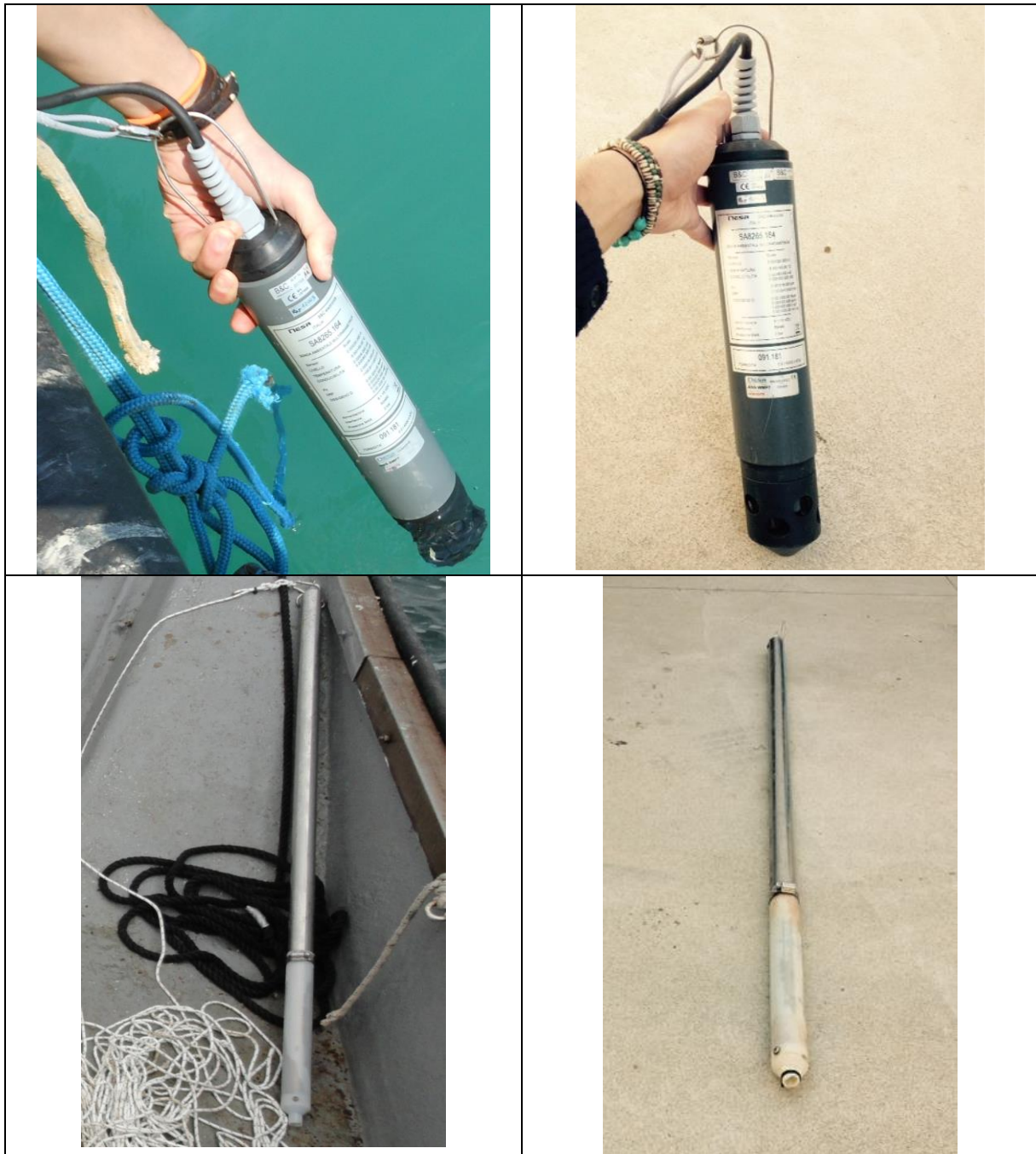
Foto 5: Sonda multiparametrica NESA e Bomb sampler utilizzato per il campionamento delle acque
