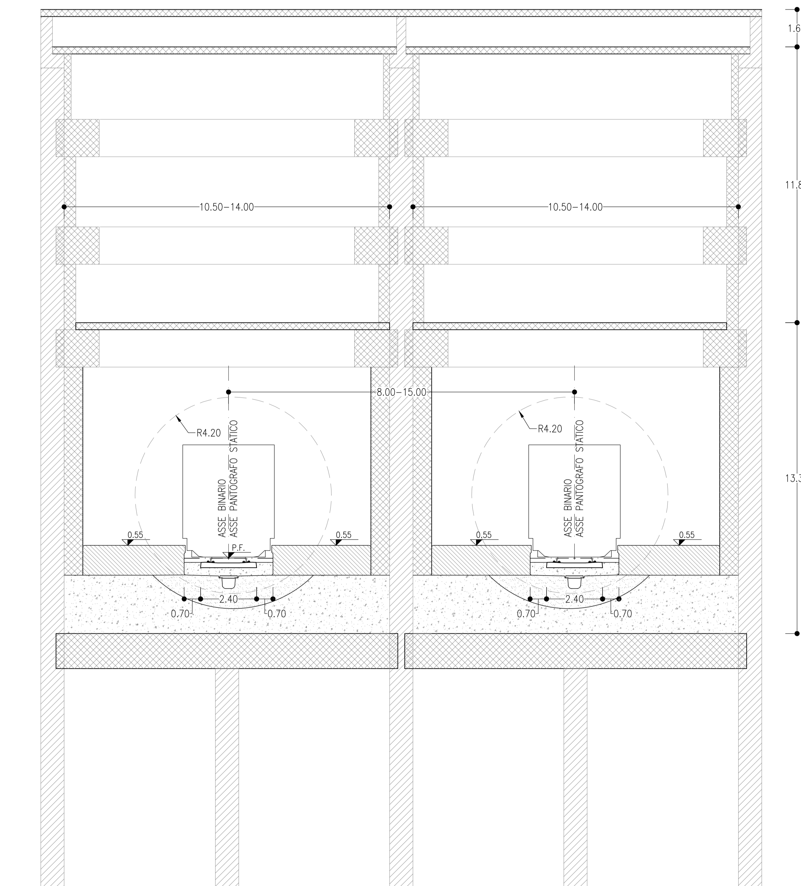
POZZO DI LANCIO SCALA 1:100 SEZIONE TRASVERSALE
