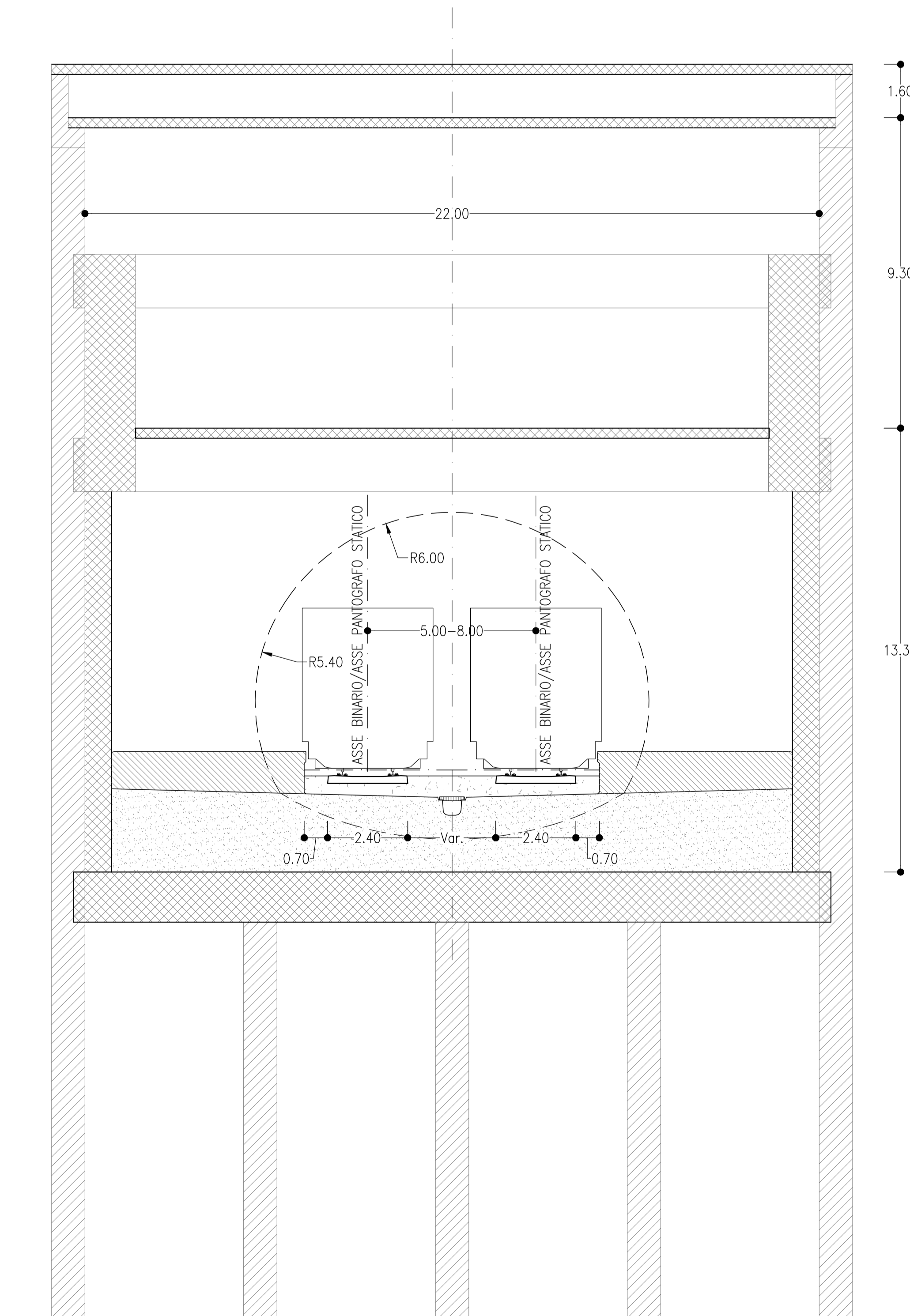
TRATTO INTERASSE BINARI 5-8 SCALA 1:100 SEZIONE TRASVERSALE
