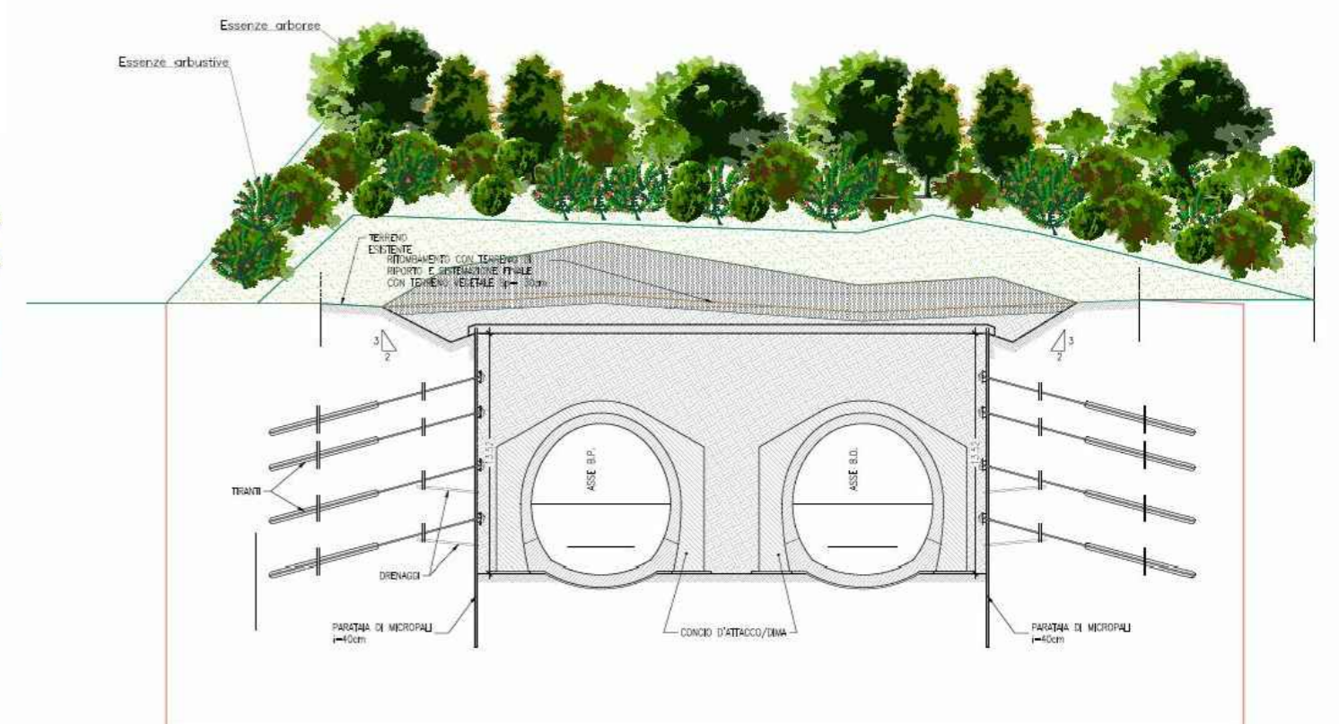
SEZIONE TIPO
