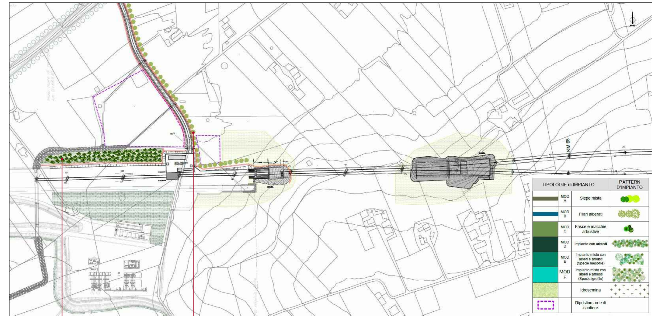
Planimetria di ubicazione delle mitigazioni
