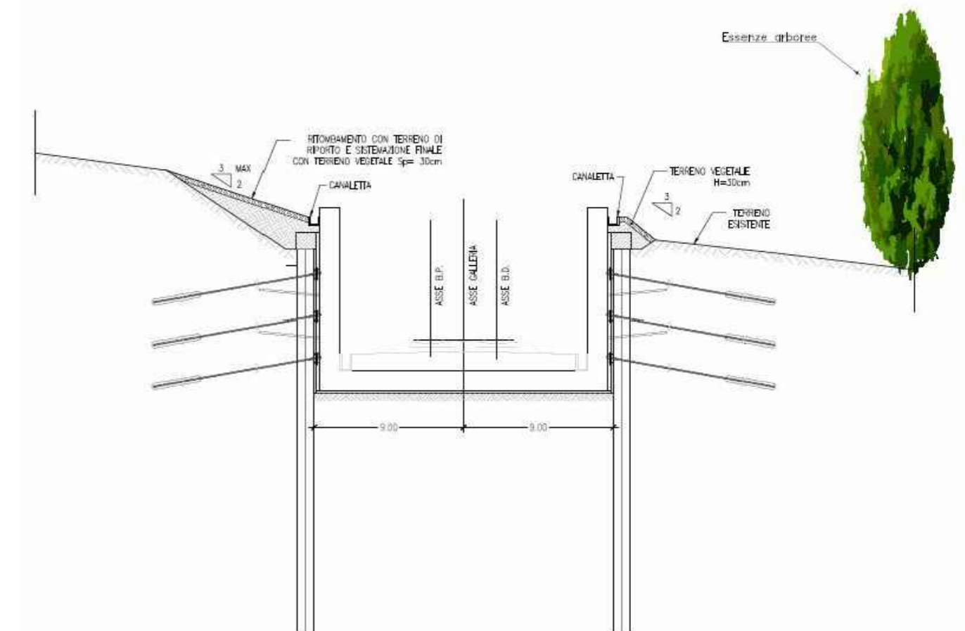
SEZIONE TIPO
