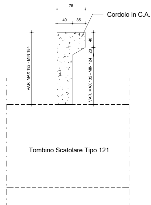
S4005 - TRATTO "B"
