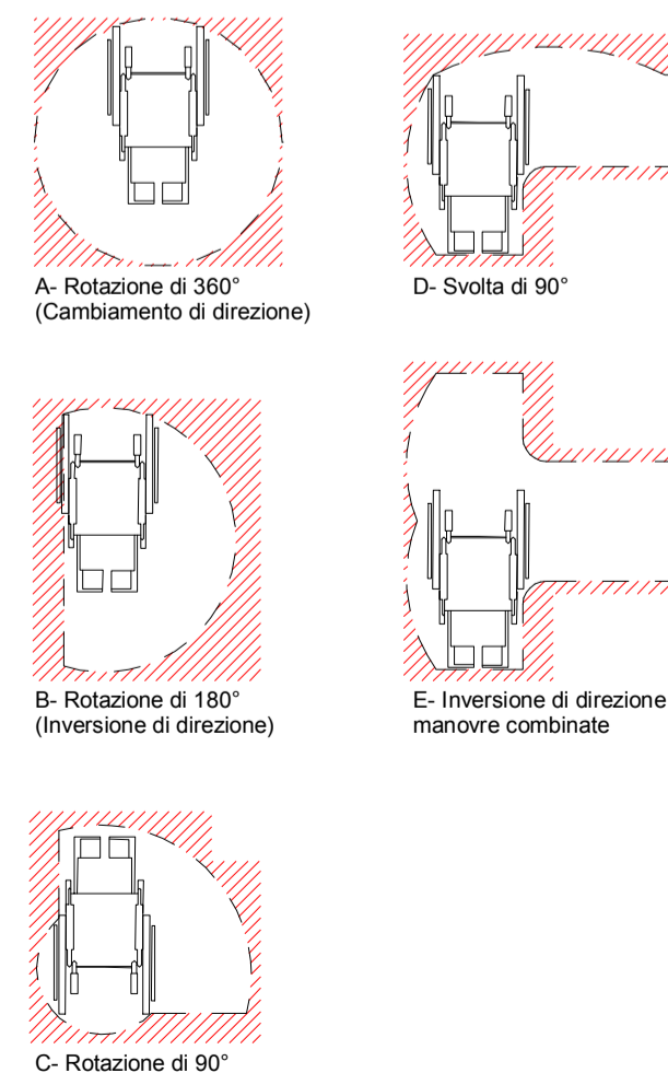
Schema spazi di manovra sedia a rotelle 1 : 50
