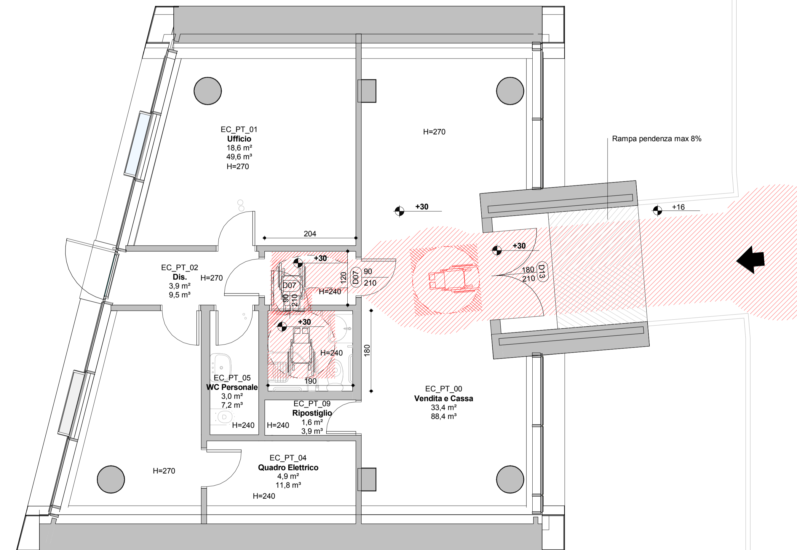
A-L0 - Pianta quotata 1 : 50
