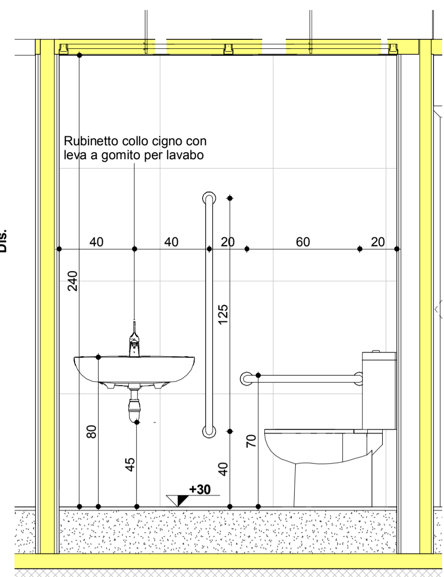
A-B - Dettaglio A 1 : 20
