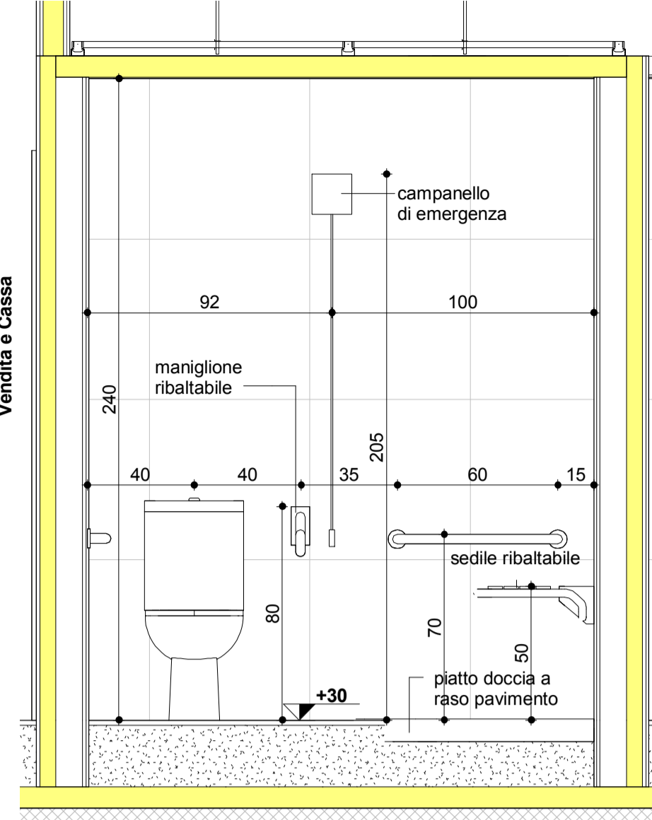
A-C - Dettaglio A 1 : 20
