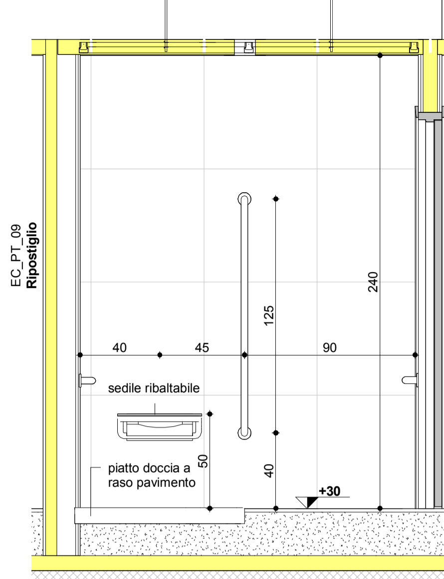
A-D - Dettaglio A 1 : 20
