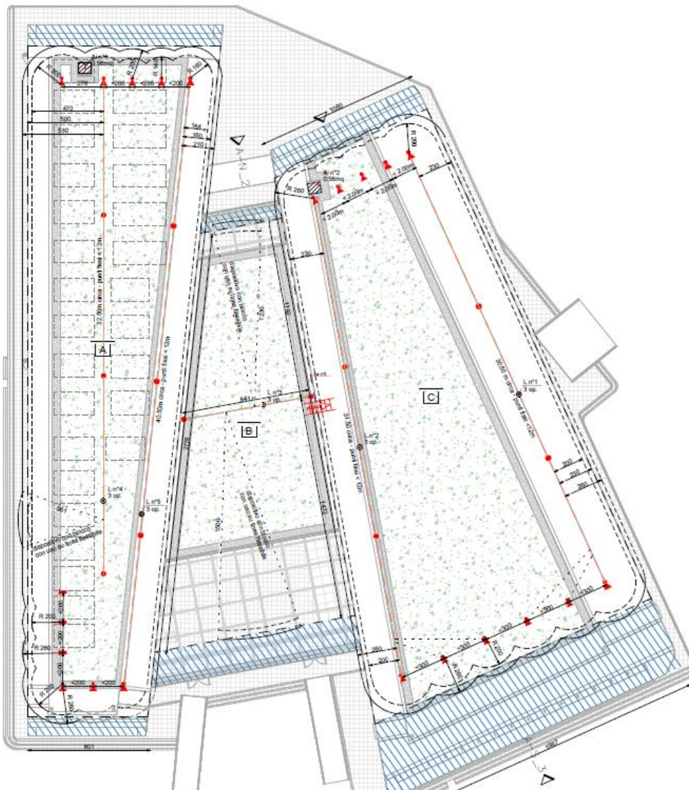
Figura 1 ó Misure di sicurezza coperture ATC
