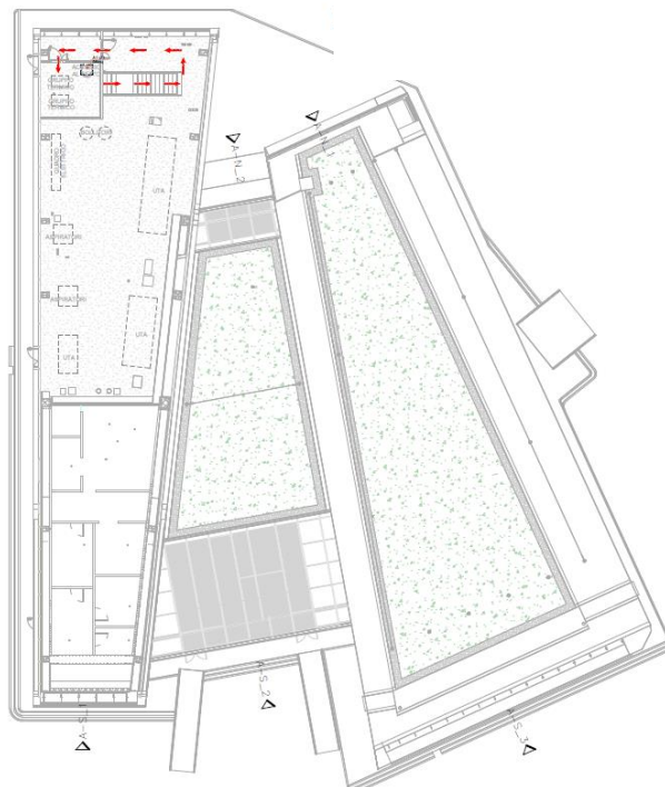
Figura 3 ó Percorsi di accesso alle coperture ó Livello 1
