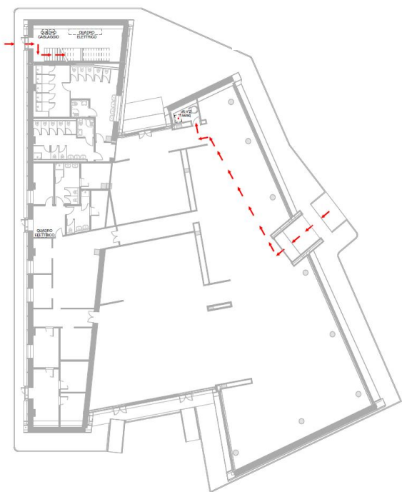
Figura 2 ó Percorsi di accesso alle coperture ó Livello 0
