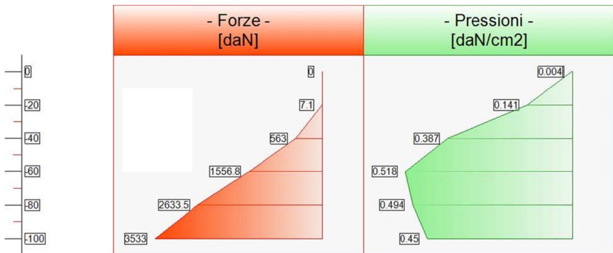
Forze (totali) e Pressioni lungo il fusto, per il Caso 11 ( GEO_ECCEZIONALE [ SLU_GEO ] - SLU_Geo_Eccezionale (appr.1;comb.2) )
