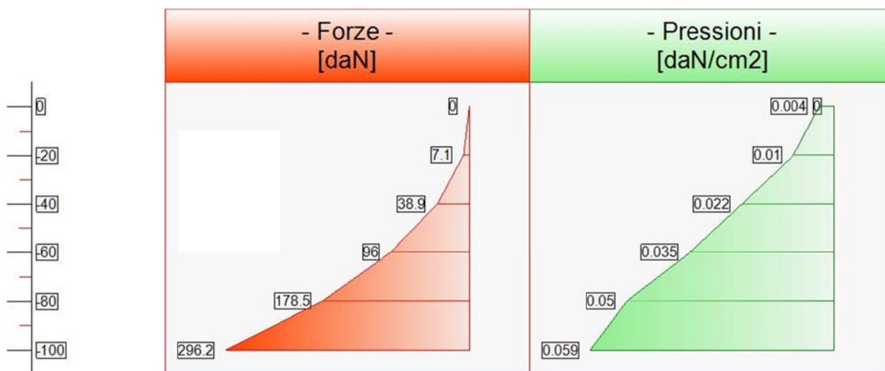
Forze (totali) e Pressioni lungo il fusto, per il Caso 2 ( GEO [ SLU_GEO ] - SLU_Geo (appr.1;comb.2) )
