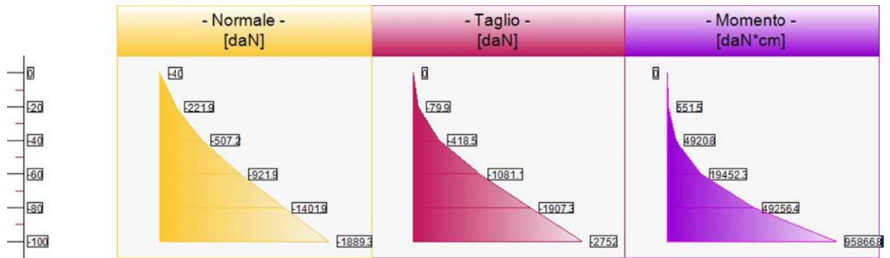
Sollecitazioni lungo il fusto, per il Caso 10 ( STR_ECCEZIONALE [ SLU ] - SLU_Str_Eccezionale (appr.1;comb.1) )
