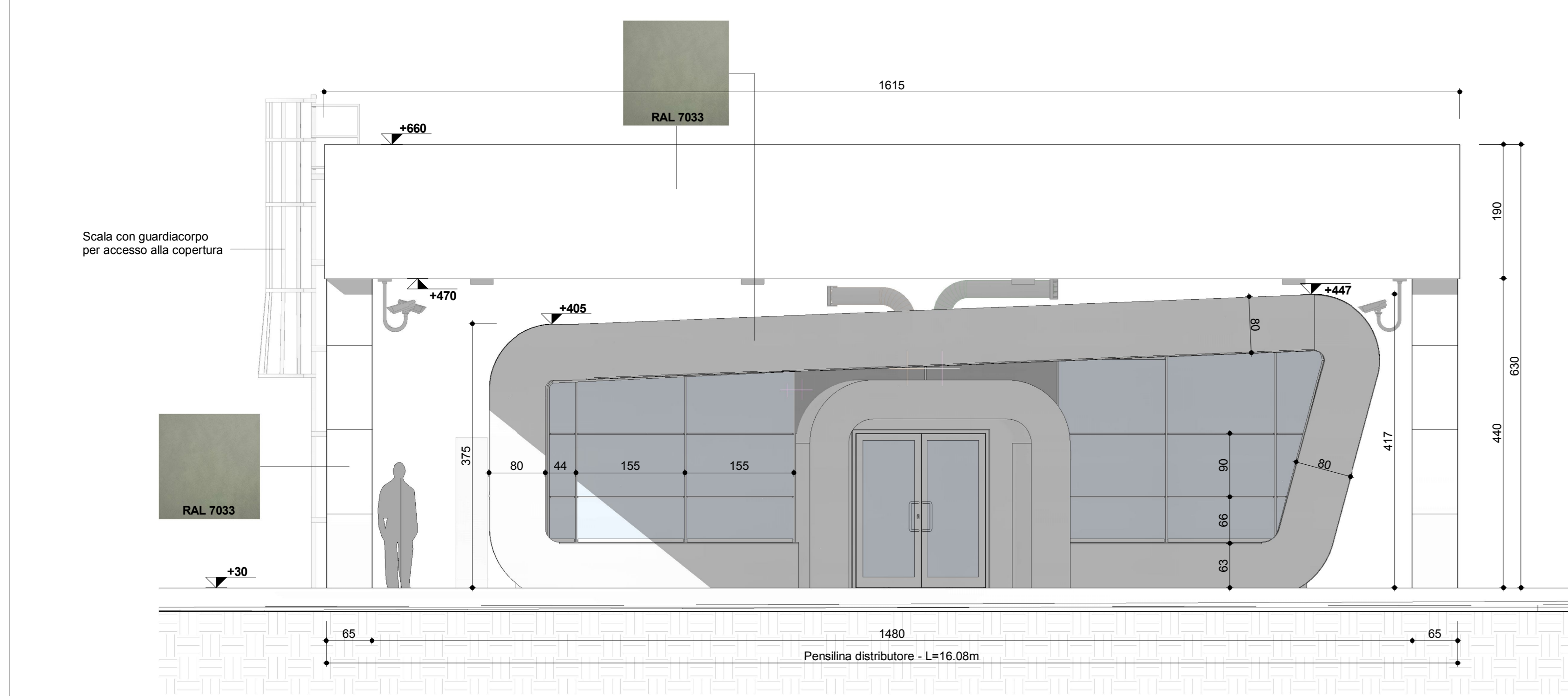
A_E - Prospetto Est 1 : 50
