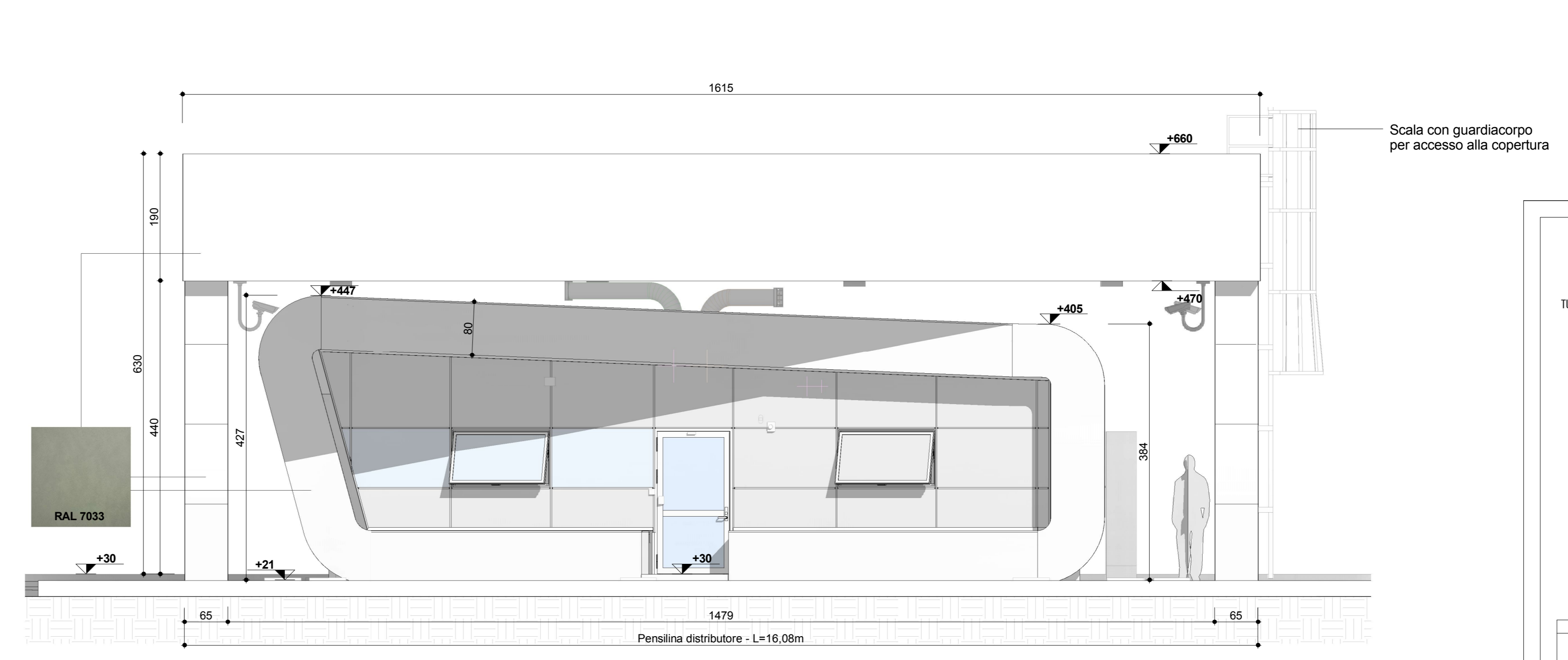
A_W - Prospetto Ovest 1 : 50
