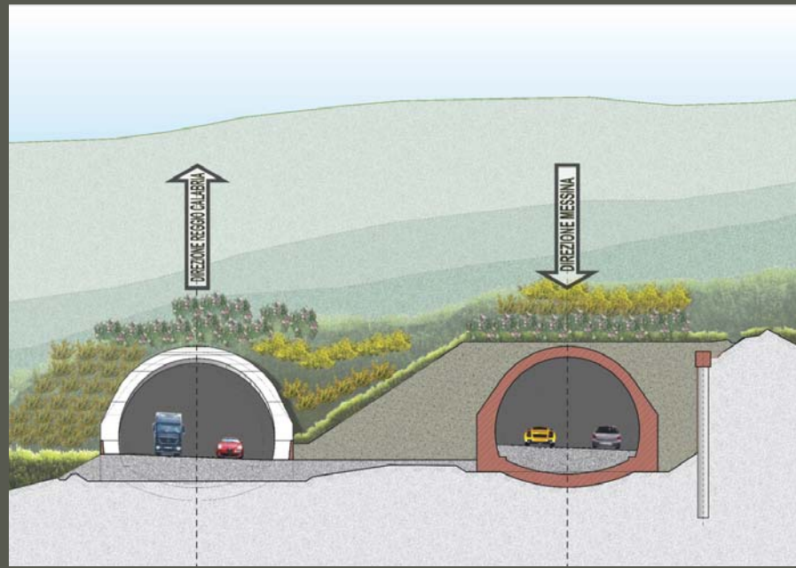
Prospetto di progetto
