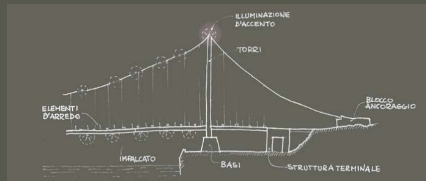
Fig. 4 - I principali elementi componenti dell'opera
