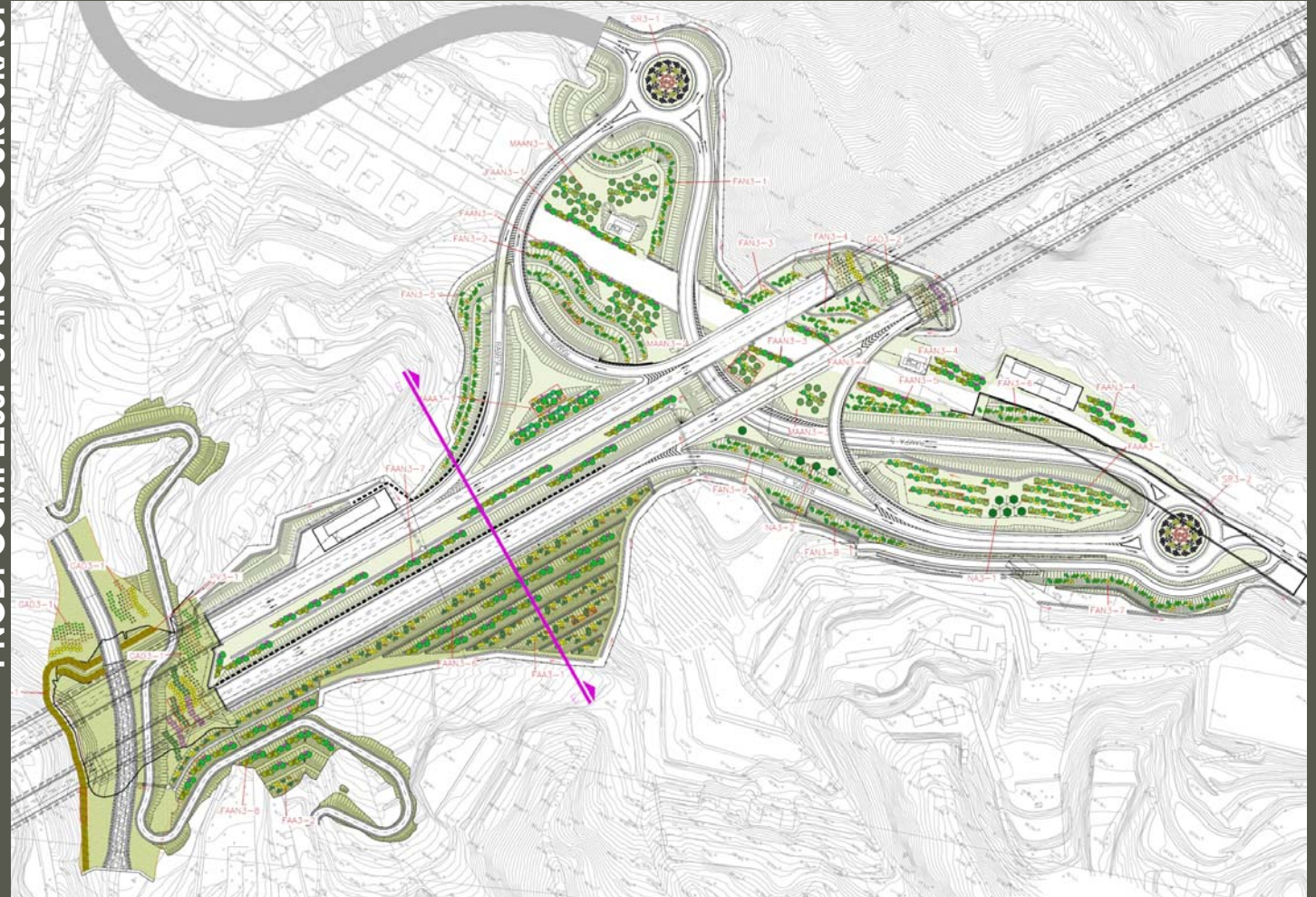
Planimetria di progetto
