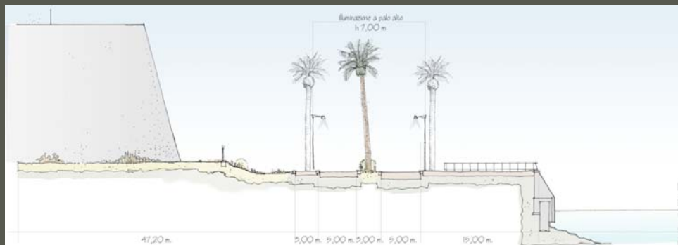
Sezione trasversale sul Lungomare di Cannitello
