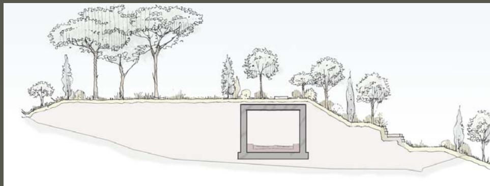
Sezione trasversale sulla Galleria Artificiale
