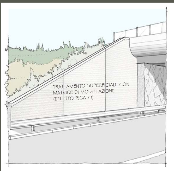
MURO DEL VIADOTTO
