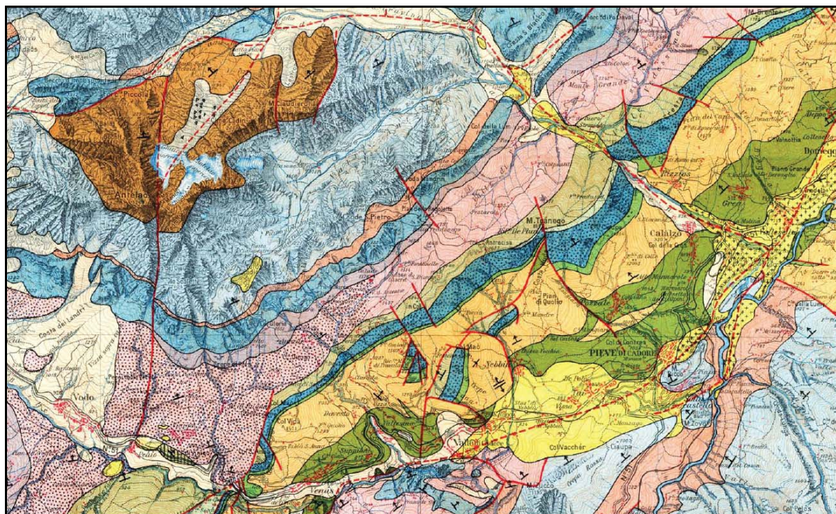
Figura 34 – Stralci della carta geologica-strutturale del Cadore (fonte Gordon, 1934)
