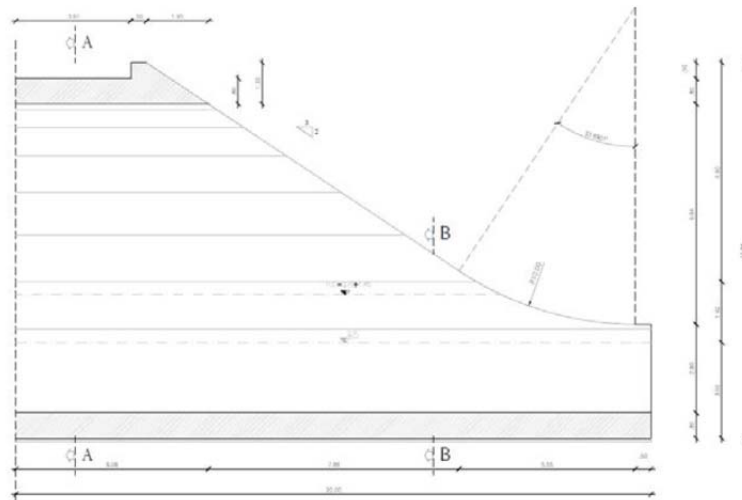
Figura 7 Imbocco Est e Ovest a becco di flauto
