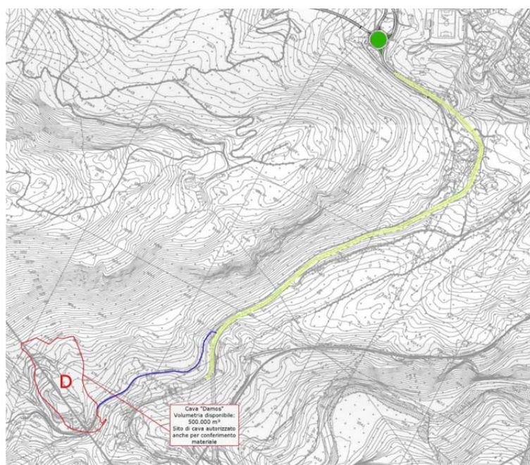
Figura 8 Corografia con ubicazione del deposito permanente (Cava "Damos")
