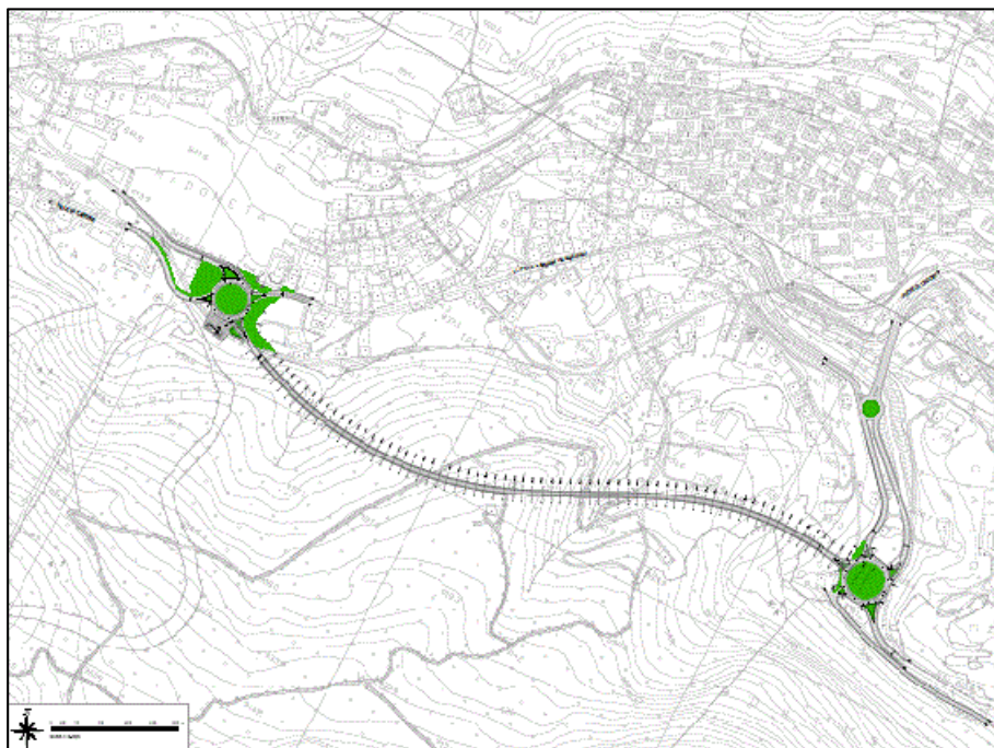
Figura 19 Planimetria del tracciato della variante in progetto (Alternativa 1)
