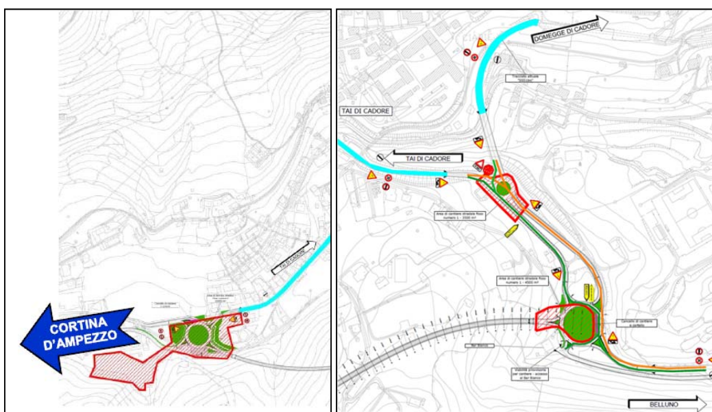
Figura 15 Stato di cantiere dell'area in esame: aree di cantiere in direzione Ovest (sx) ed Est (dx)
