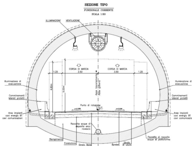
Figura 6 Sezione corrente della galleria tipo C2 Anas
