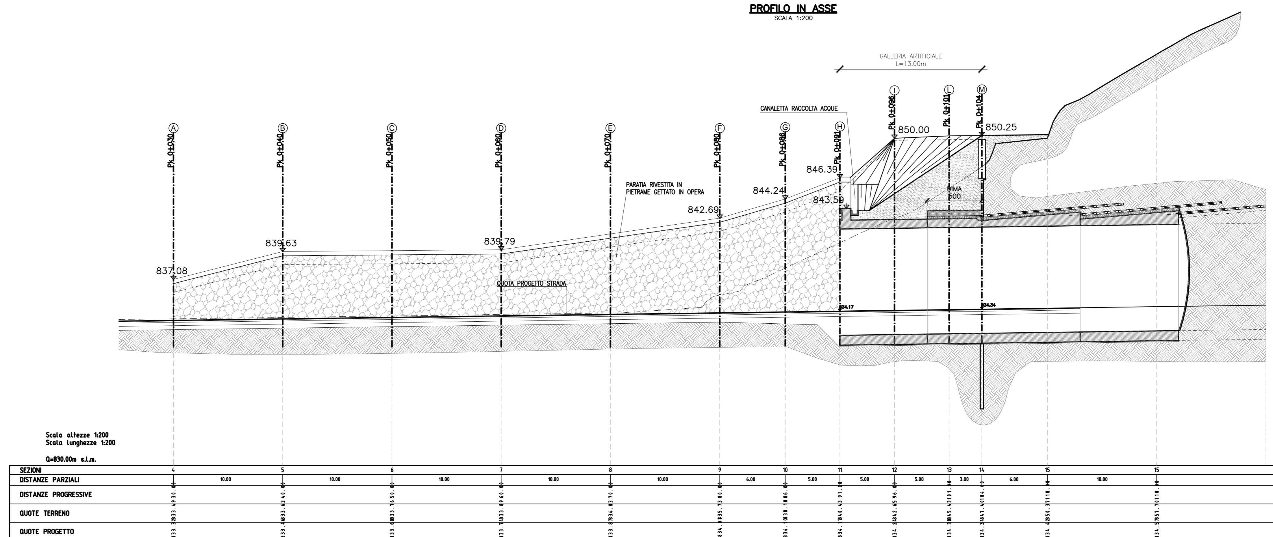
PROFilo IN ASSE SCALA 1:200
