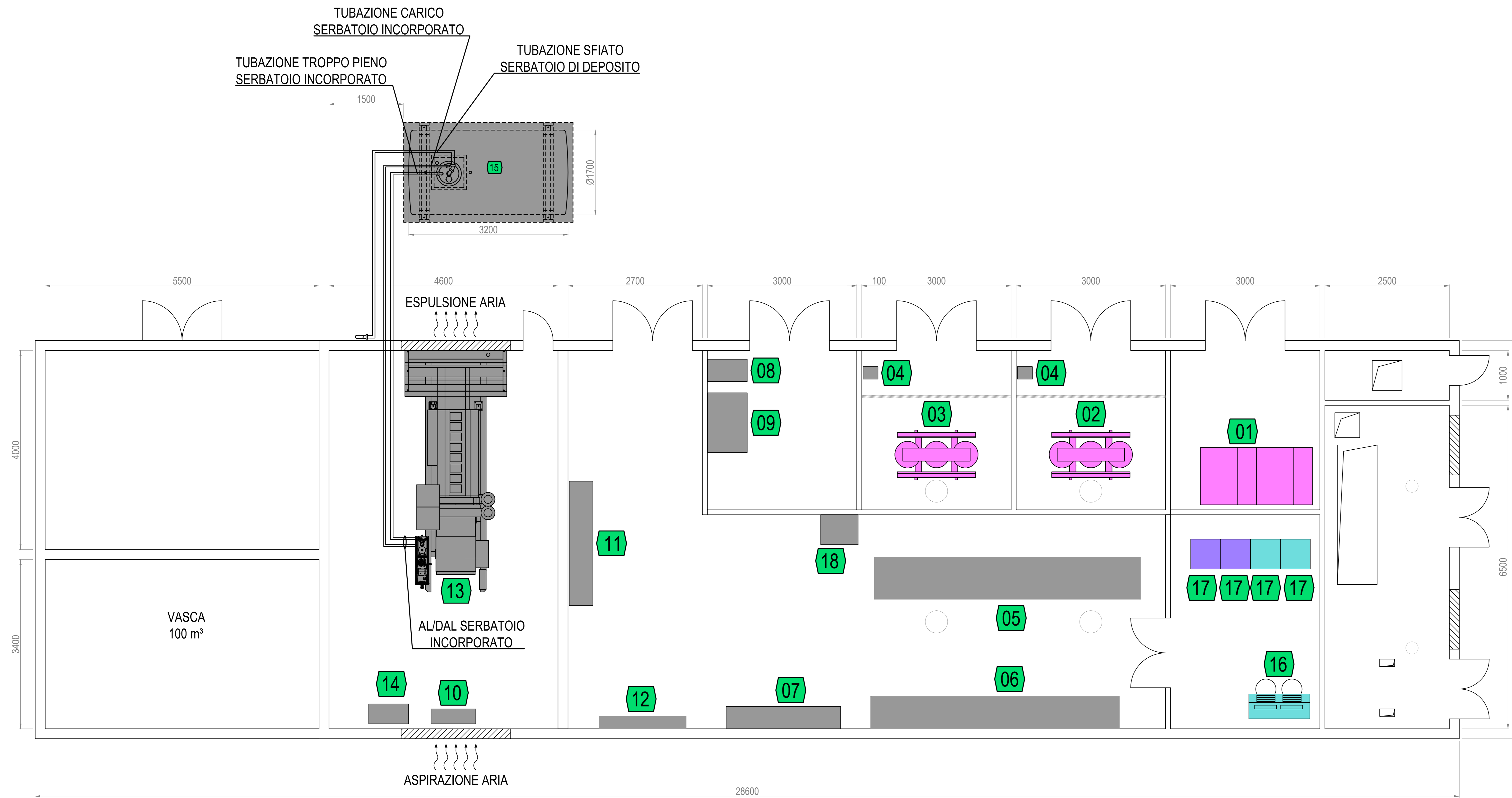
PLANIMETRIA D'INQUADRAMENTO Scala 1:500
