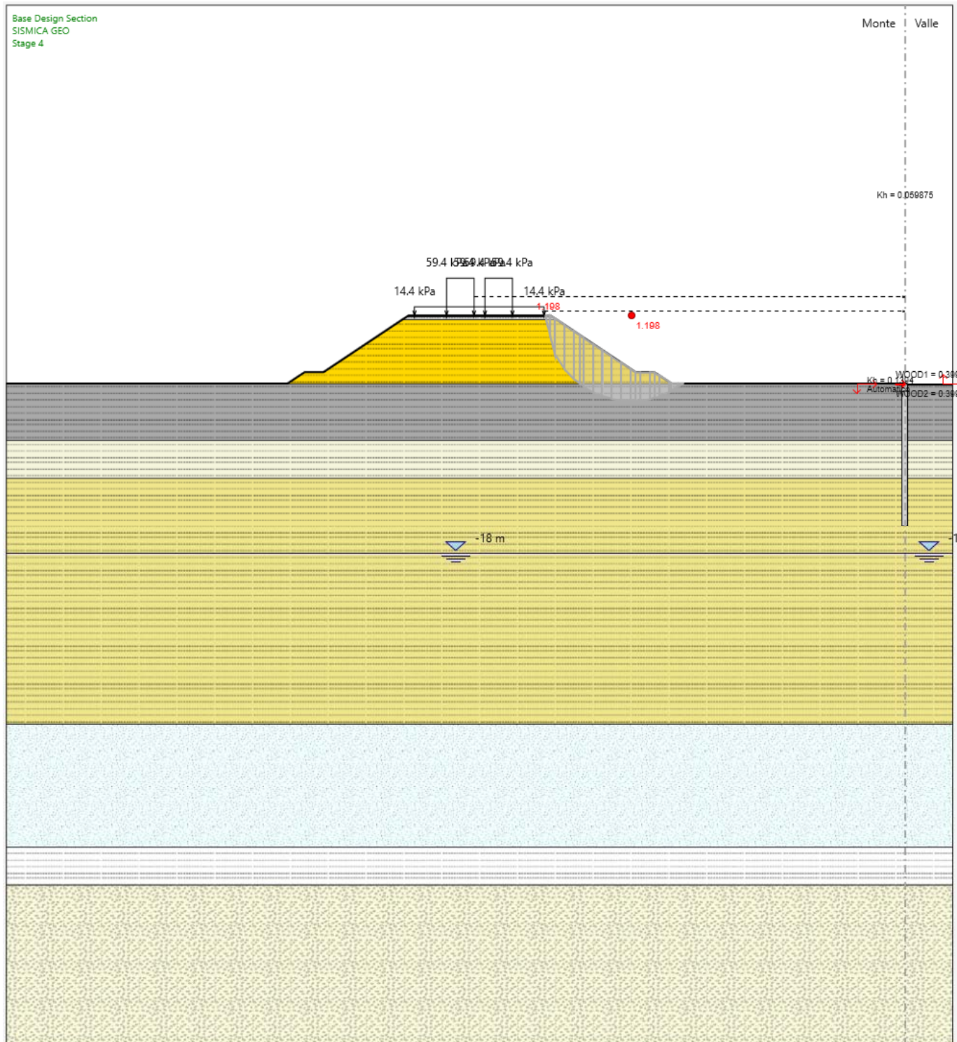
Fig. 2: Rilevato H (distanza PF e PC) = 8.0 m (da pk 7+402 a pk 7+724) - Analisi di stabilità globale in campo sismico
