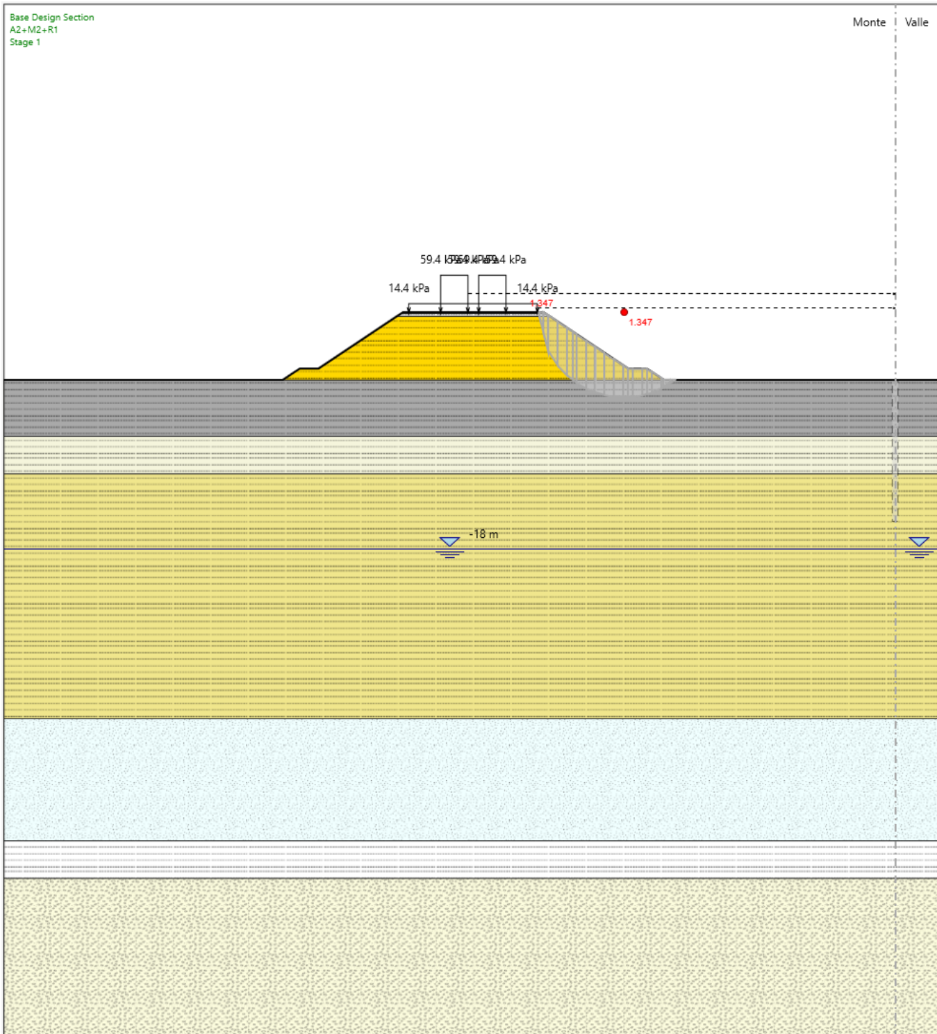
Fig. 1: Rilevato H (distanza PF e PC) = 8.0 m (da pk 7+402 a pk 7+724) - Analisi di stabilità globale in campo statico DA1C2
