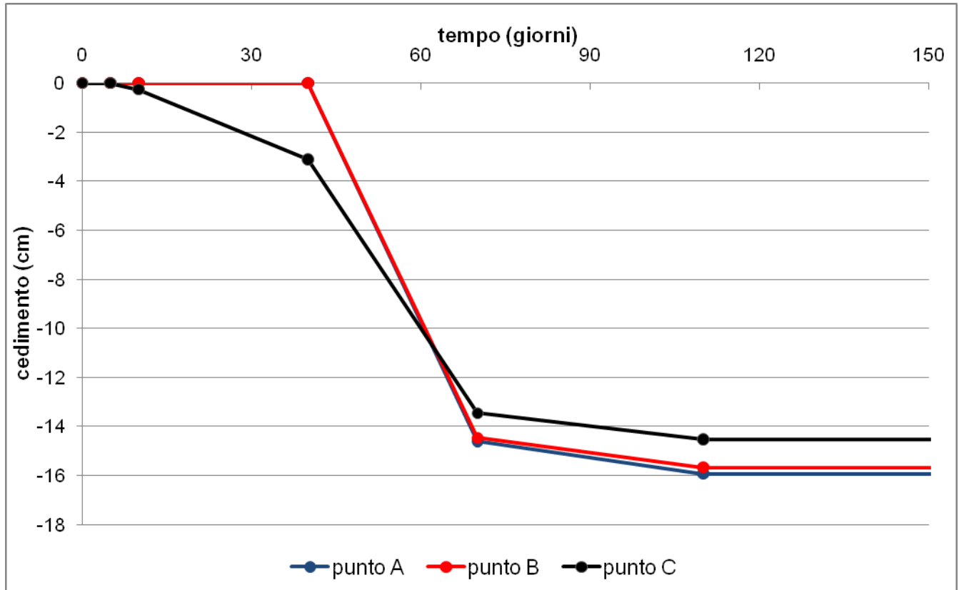
Figura 4 – Rilevato H (distanza PF – PC) = 8.0 m (da pk 7+402 a pk 7+724) – Analisi SLE – Curve cedimento – tempo.
