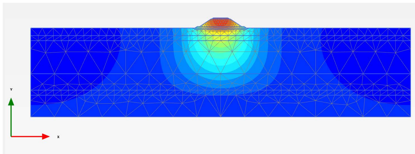
Figura 2 – Rilevato H (distanza PF – PC) = 8.0 m (da pk 7+402 a pk 7+724) – Analisi SLE – Campo dei cedimenti a 1 anno.
