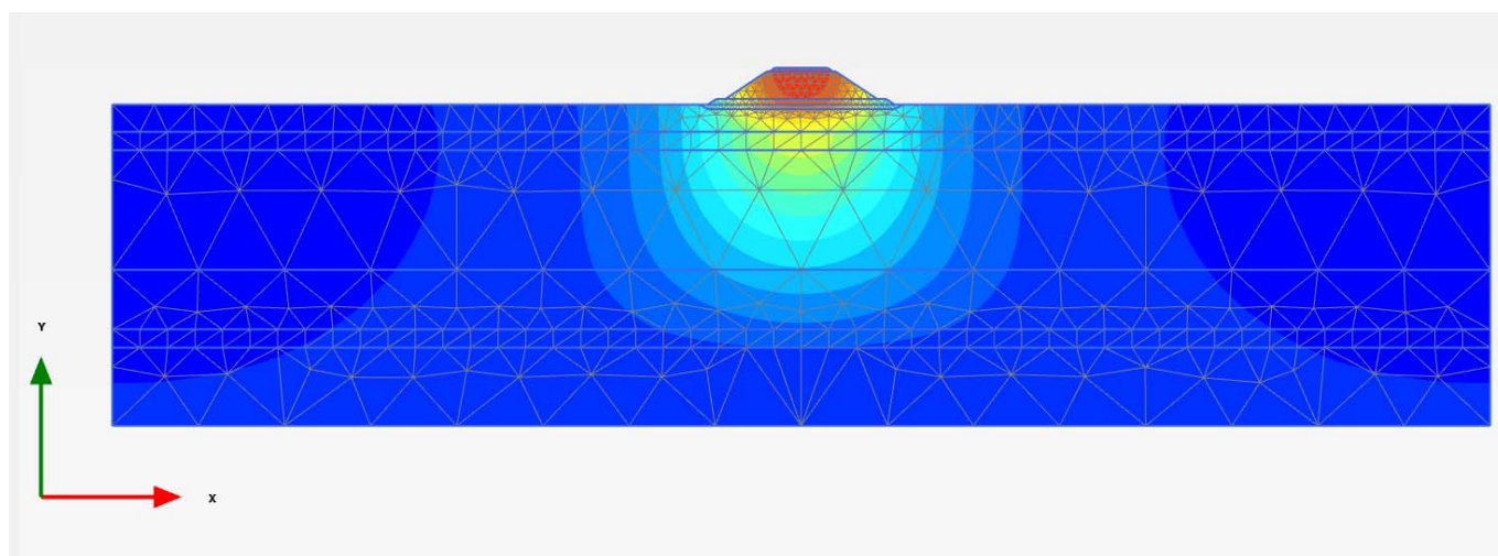
Figura 3 – Rilevato H (distanza PF – PC) = 8.0 m (da pk 7+402 a pk 7+724) – Analisi SLE – Campo dei cedimenti a 100 anni.
