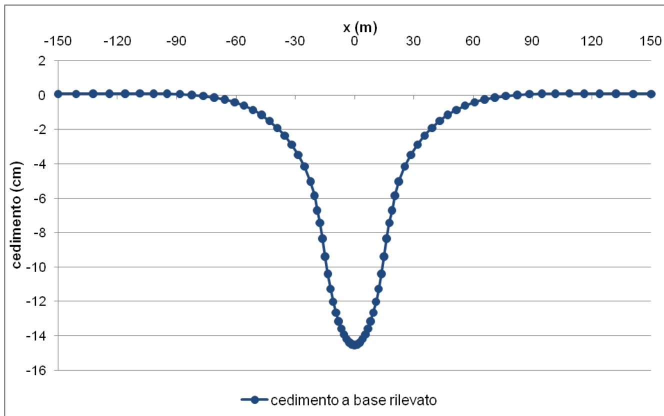
Figura 5 – Rilevato H (distanza PF – PC) = 8.0 m (da pk 7+402 a pk 7+724) – Analisi SLE – Cedimenti indotti sul rilevato esistente.
