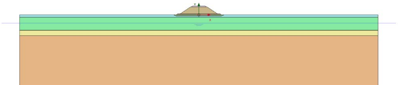
Figura 1 – Rilevato H (distanza PF – PC) = 7.6 m (da pk 13+609 a pk 14+415) – Analisi SLE – Modello Plaxis 2D.
