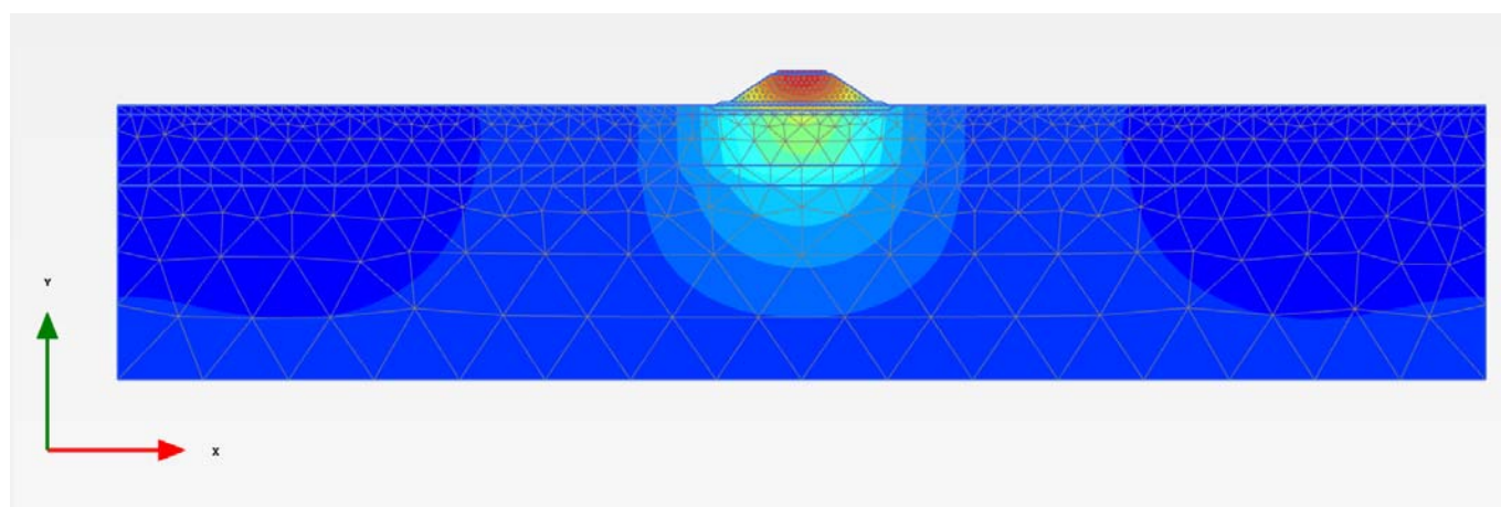
Figura 3 – Rilevato H (distanza PF – PC) = 7.6 m (da pk 13+609 a pk 14+415) – Analisi SLE – Campo dei cedimenti a 100 anni.
