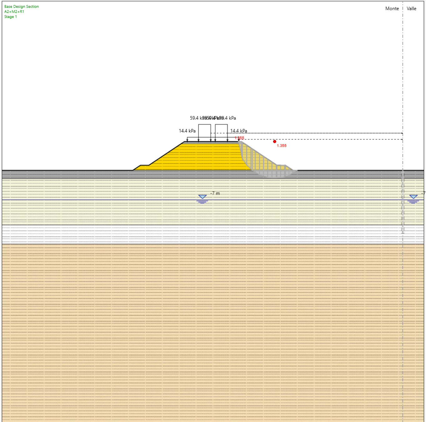
Fig. 1: Rilevato H (distanza PF e PC) = 7.6 m (da pk 13+609 a pk 14+415) - Analisi di stabilità globale in campo statico DA1C2
