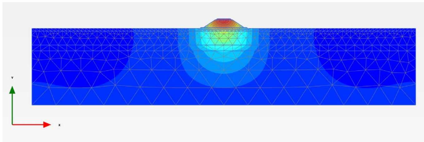
Figura 2 – Rilevato H (distanza PF – PC) = 7.6 m (da pk 13+609 a pk 14+415) – Analisi SLE – Campo dei cedimenti a 1 anno.
