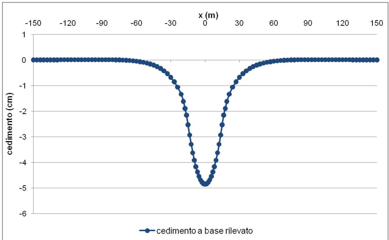
Figura 5 – Rilevato H (distanza PF – PC) = 7.6 m (da pk 13+609 a pk 14+415) – Analisi SLE – Cedimenti indotti sul rilevato esistente.
