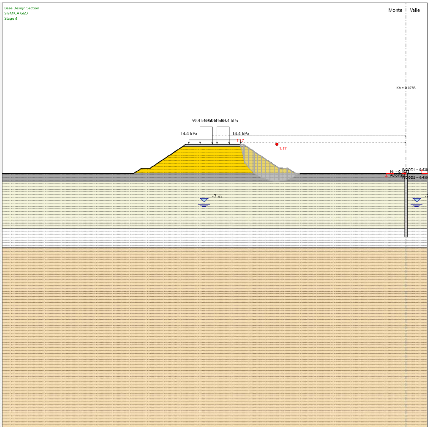
Fig. 2: Rilevato H (distanza PF e PC) = 7.6m (da pk 13+609 a pk 14+415) - Analisi di stabilità globale in campo sismico
