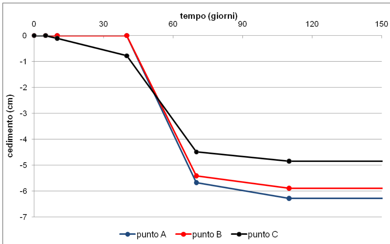
Figura 4 – Rilevato H (distanza PF – PC) = 7.6 m (da pk 13+609 a pk 14+415) – Analisi SLE – Curve cedimento – tempo.
