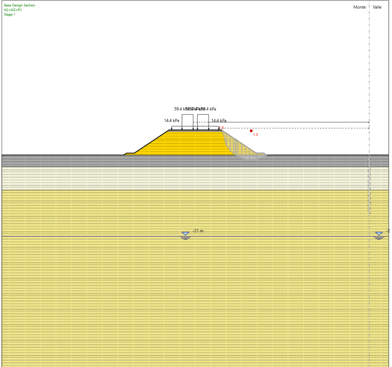
Fig. 1: Rilevato H (distanza PF e PC) = 7.3 m (da pk 2+201 a pk 2+518) - Analisi di stabilità globale in campo statico DA1C2
