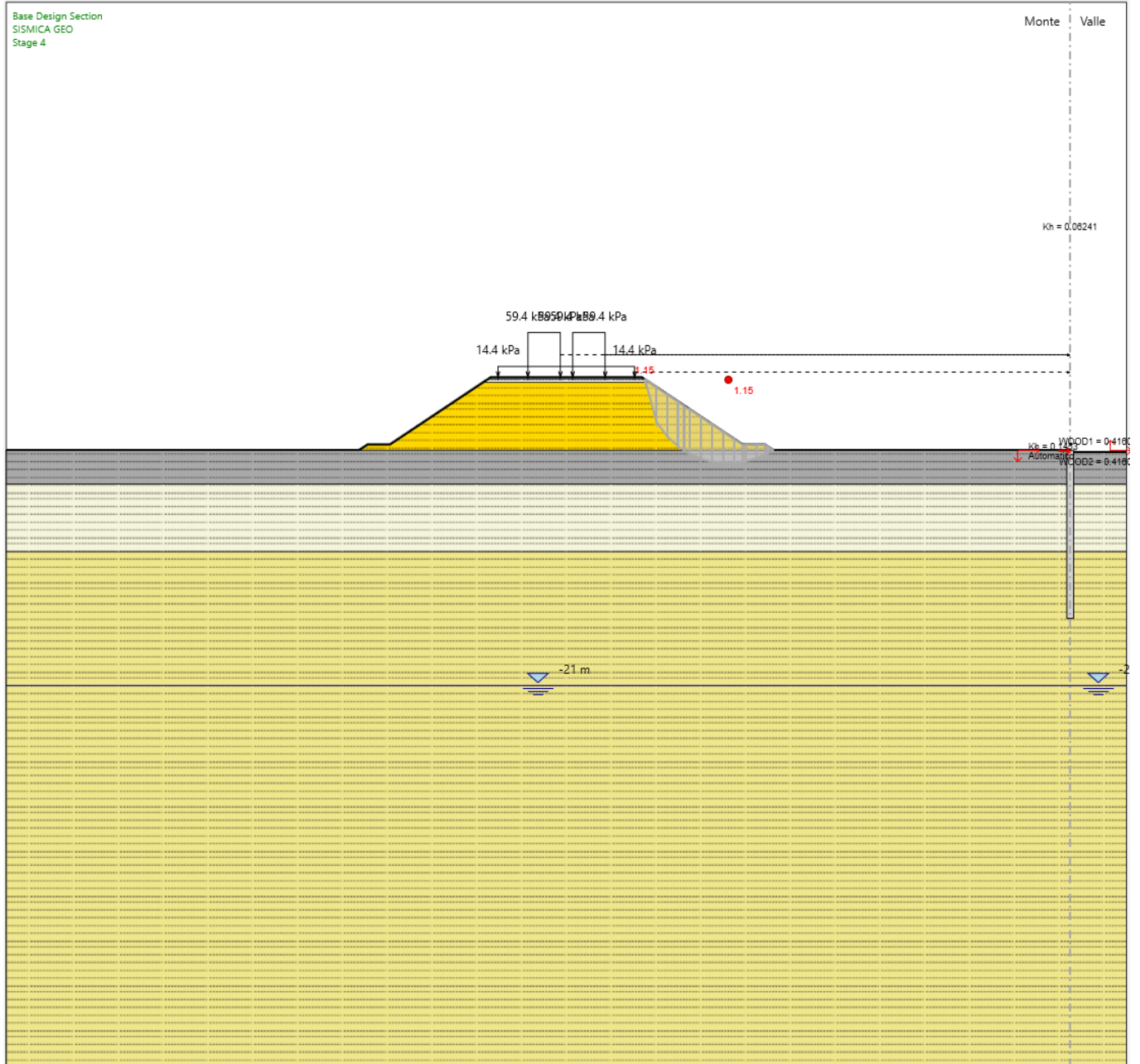
Fig. 2: Rilevato H (distanza PF e PC) = 7.3 m (da pk 2+201 a pk 2+518) - Analisi di stabilità globale in campo sismico
