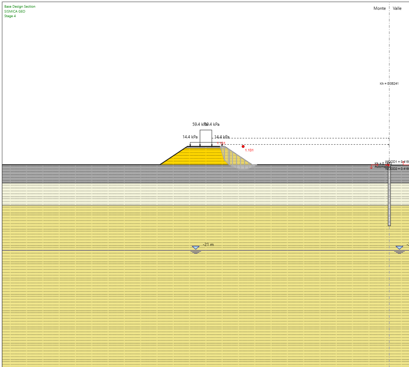
Fig. 2: Rilevato H (distanza PF e PC) = 5.3 m (pk 1+375 BD circa) - Analisi di stabilità globale in campo sismico
