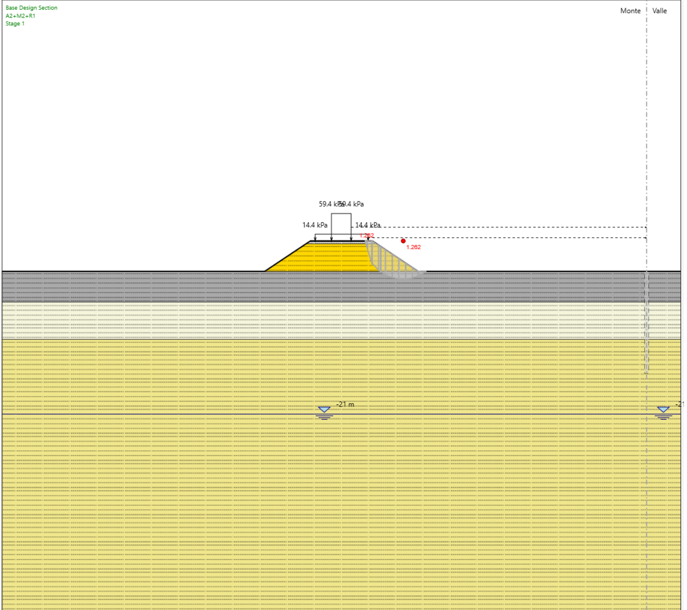
Fig. 1: Rilevato H (distanza PF e PC) = 5.3 m (pk 1+375 BD circa) - Analisi di stabilità globale in campo statico DA1C2
