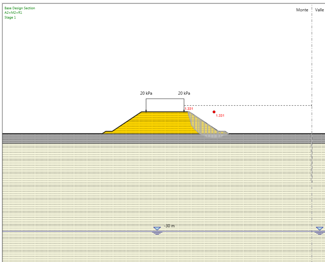
Fig. 1: Rilevato H = 6.7 m (pk 2+225 BD) - Analisi di stabilità globale in campo statico DA1C2.
