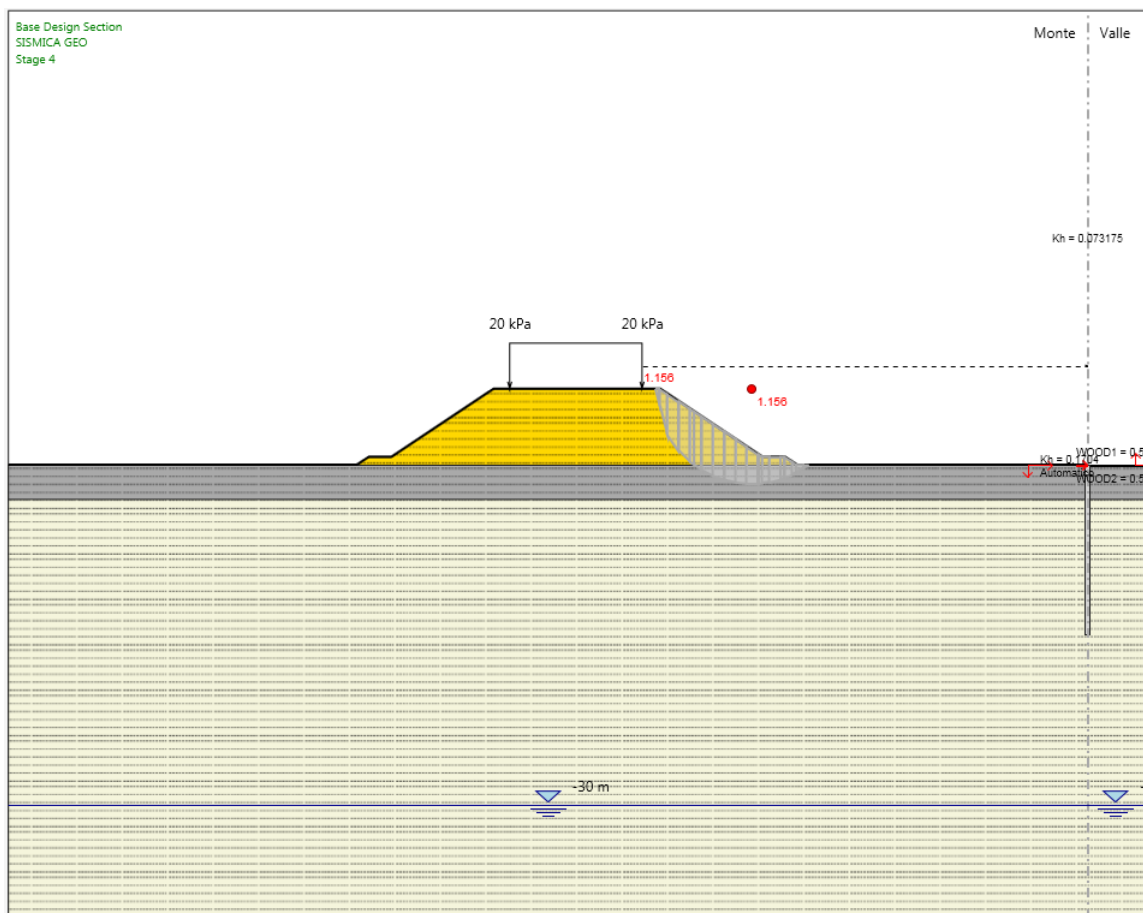
Fig. 2: Rilevato H = 6.7 m (pk 2+225 BD) - Analisi di stabilità globale in campo sismico.
