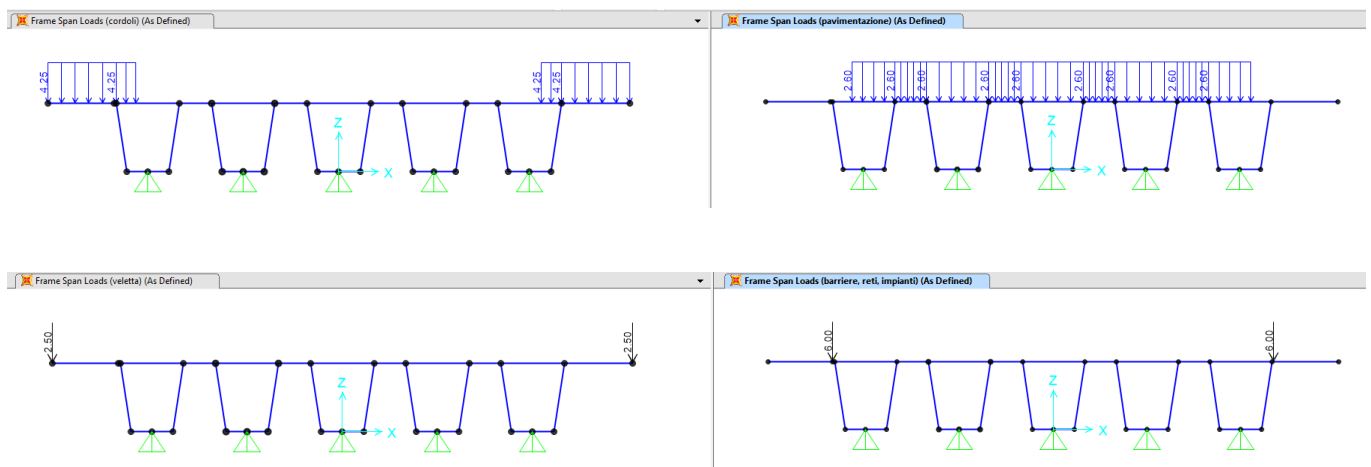
Figura 23 – Applicazione dei carichi permanenti non strutturali (G2) sul modello agli E.F.
