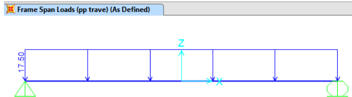
Figura 3 – modello di calcolo f.e.m. fase 0 – carico distribuito dovuto al peso proprio della trave
