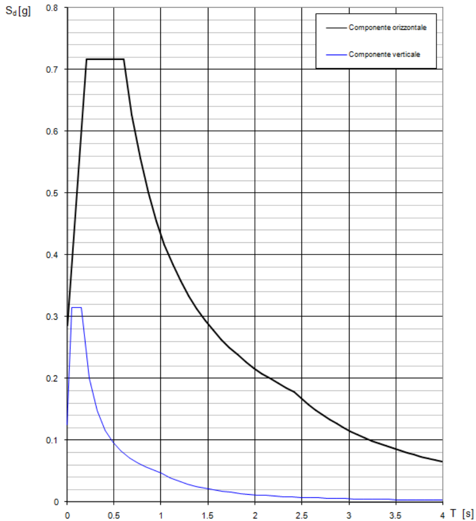
Figura 18 – Spettro di progetto allo SLV – componente orizzontale e verticale
