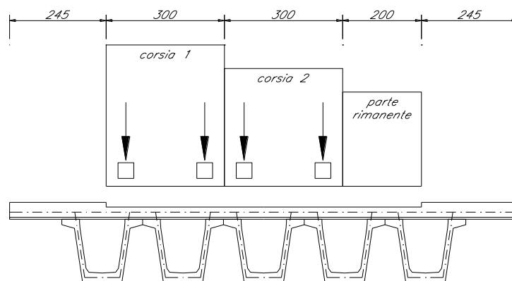
Figura 24 – Schema 1 - Disposizione 1
