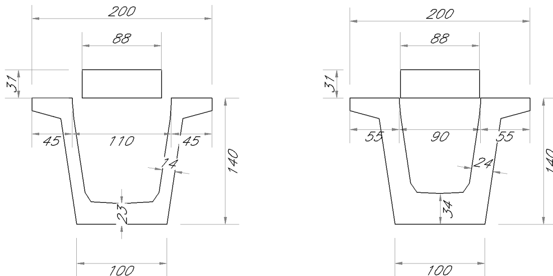
Figura 9 – Sezioni in Fase 3 (cassoncino con soletta omogeneizzata a l.t.): sezione corrente e sezione di transizione - sezione di testata
