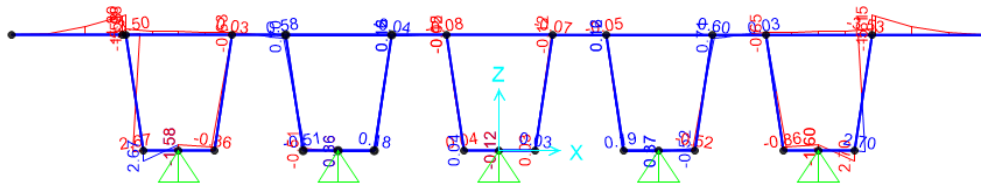
Moment 3-3 Diagram (vento)
