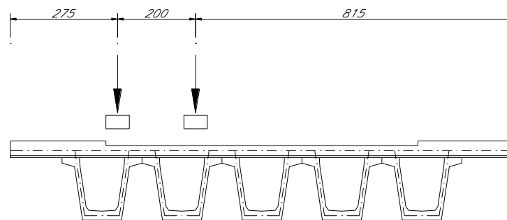
Figura 28 – Schema 2 - Disposizione 1
