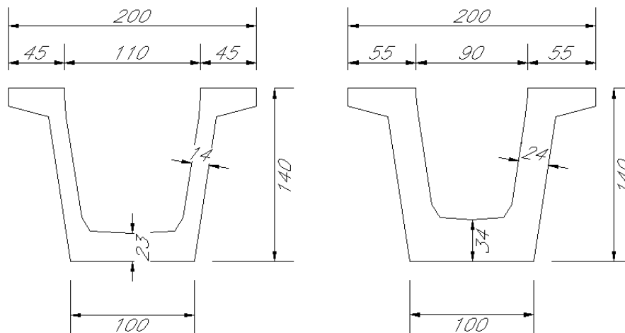
Figura 7 – Sezioni in Fase 1 (cassoncino): sezione corrente e sezione di transizione - sezione di testata
