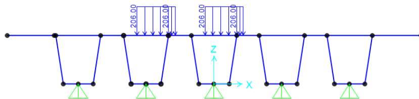
Figura 31 – Assegnazione carichi su modello agli E.F. - Schema 2 - Disposizione 2 (Q2-2)
