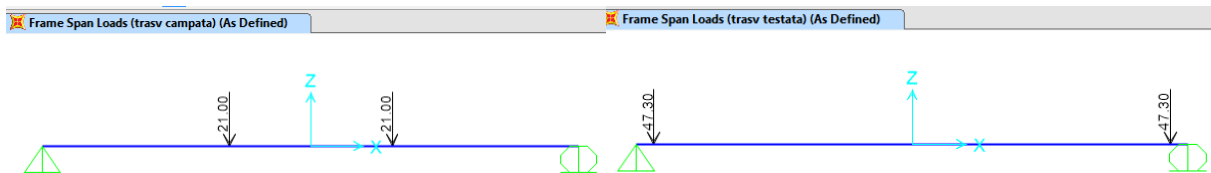
Figura 4 – modello di calcolo f.e.m. fase 0 – carichi concentrati dovuti al peso dei trasversi
