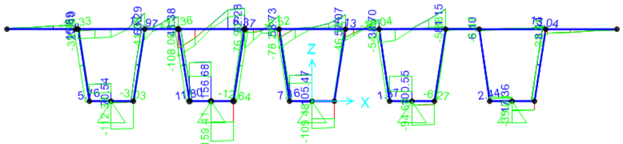
Figura 38 – Taglio - Combinazione di involucro SLE-Frequente e SLE-Rara
