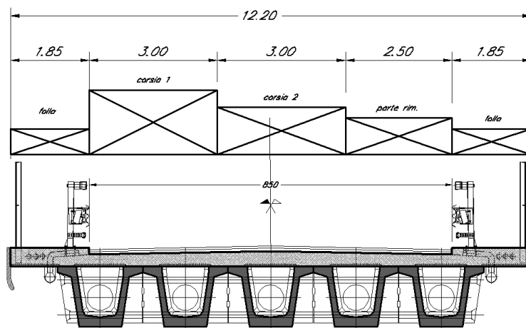
Figura 14 – Disposizione corsie convenzionali
