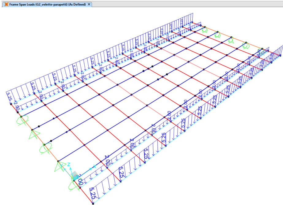
Figura 11 – Applicazione al modello agli EF dei carichi permanenti non strutturali G2_velette, parapetti, impianti
