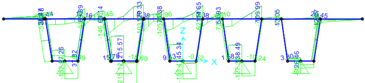
Figura 36 – Taglio - Combinazione di involucro SLU-STR e SLU-ECC
