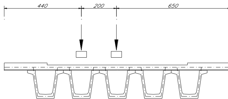
Figura 30 – Schema 2 - Disposizione 2
