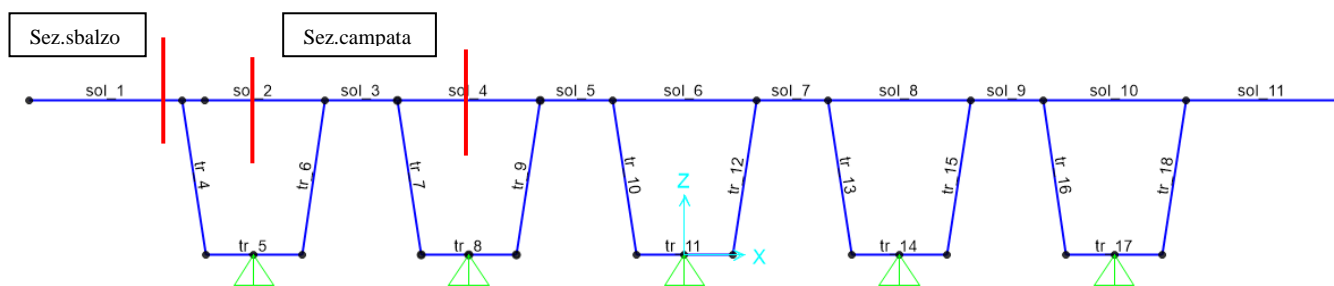
Figura 39 – Sezioni di verifica (“sbalzo” e “campata”)
