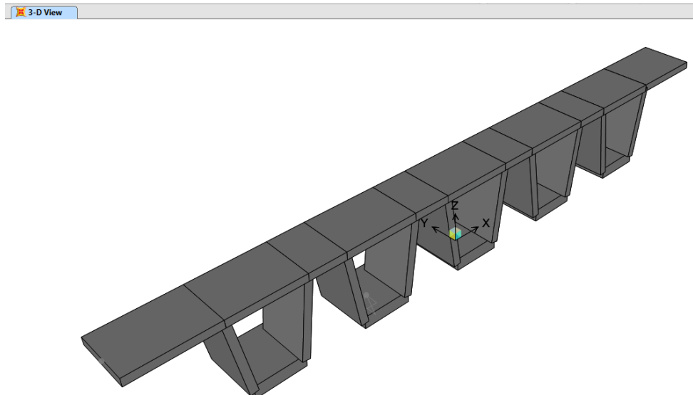
Figura 21 – Vista estrusa del modello 2D agli E.F.
