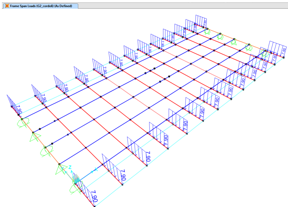
Figura 10 – Applicazione al modello agli EF dei carichi permanenti non strutturali G2_cordoli
