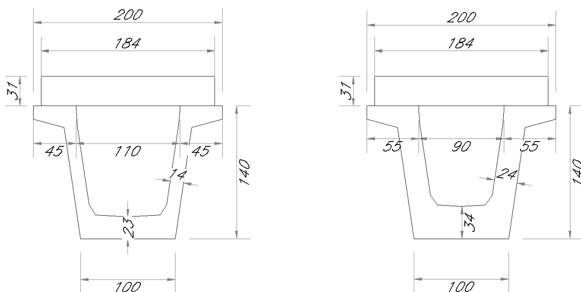
Figura 8 – Sezioni in Fase 2 (cassoncino con soletta omogeneizzata a b.t.): sezione corrente e sezione di transizione - sezione di testata
