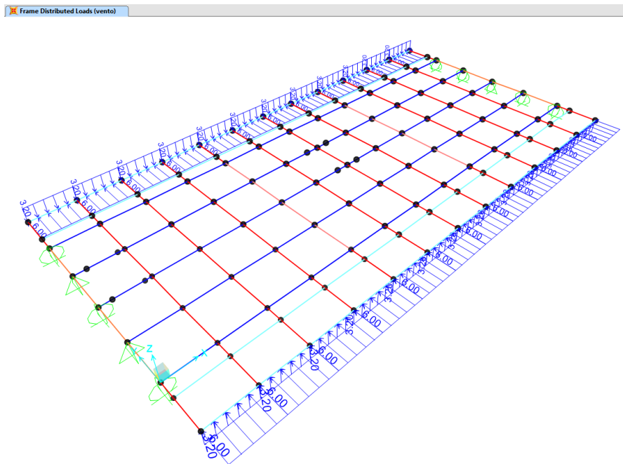
Figura 17 – Applicazione carichi del vento sul modello agli EF
