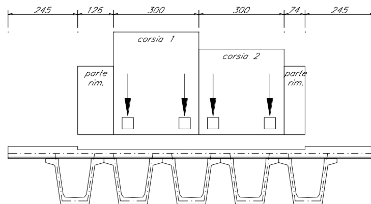
Figura 26 – Schema 1 - Disposizione 1
