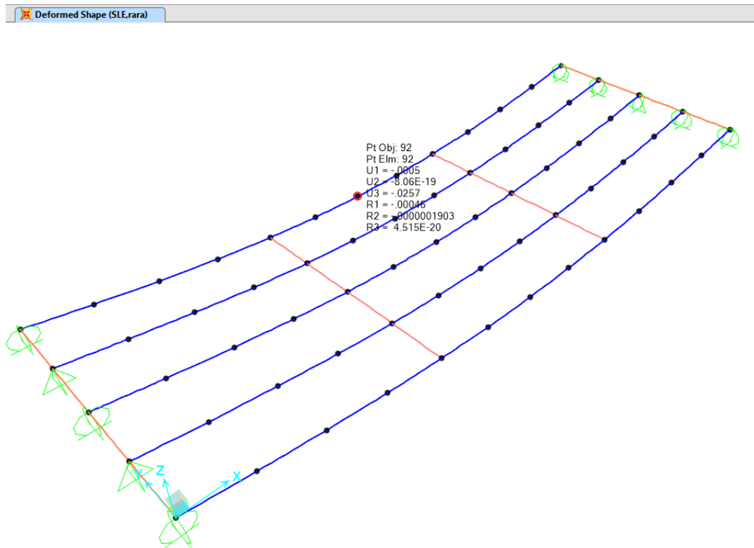
Figura 20 – Deformata dell'impalcato sotto l'effetto dei carichi accidentali (traffico e vento)
