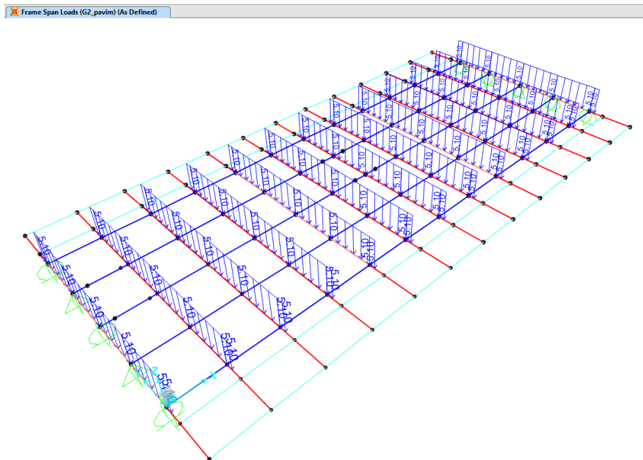
Figura 12– Applicazione al modello agli EF dei carichi permanenti non strutturali G2_pavimentazione
