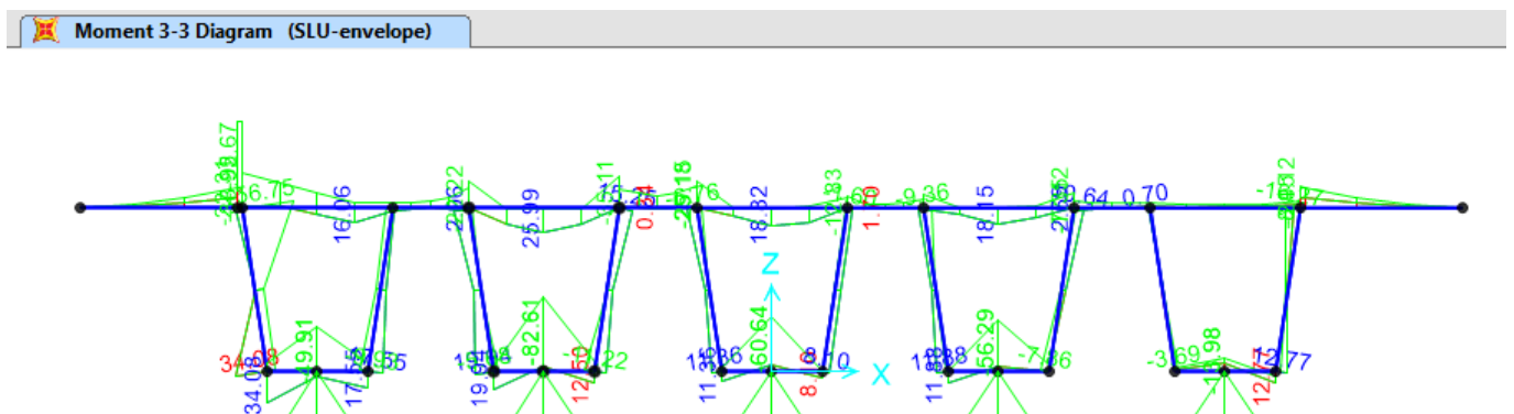
Figura 35 – Momento flettente - Combinazione di involucro SLU-STR e SLU-ECC
