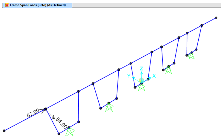
Figura 33 – Assegnazione carichi su modello agli E.F. - Urto (Q4)
