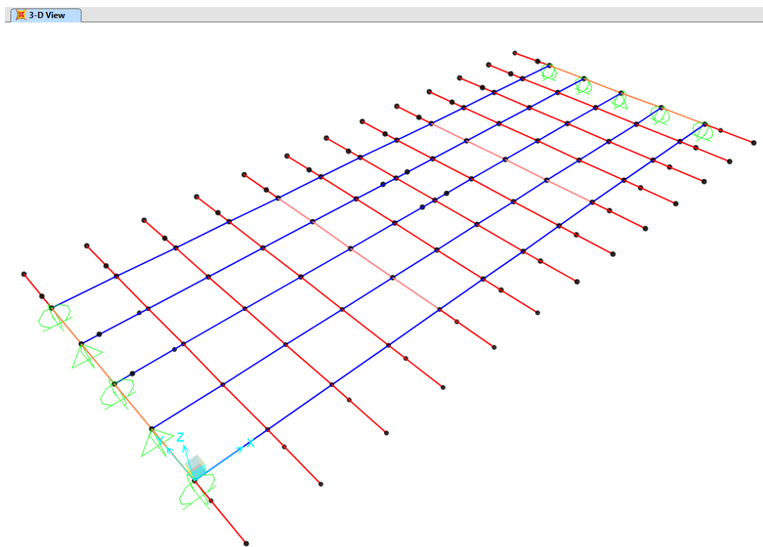
Figura 6 – Vista del modello 3D agli elementi finiti
