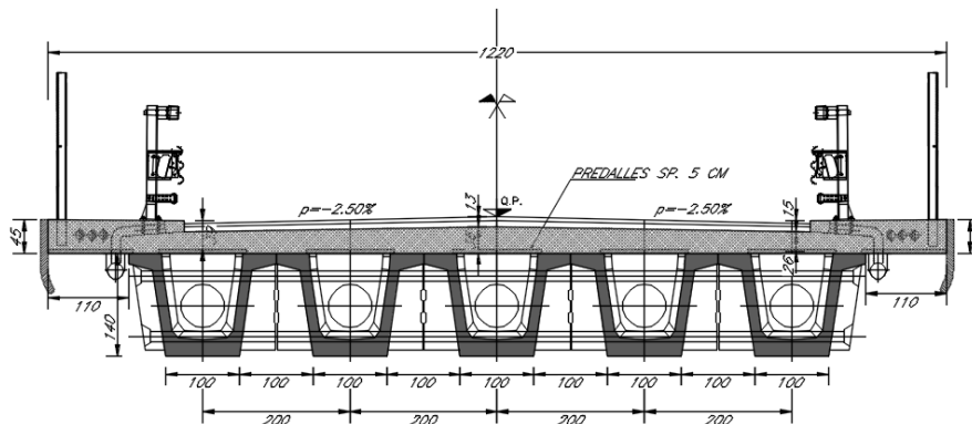
Figura 1 – Sezione tipo cavalcaferrovia campata. L=25,00 m
