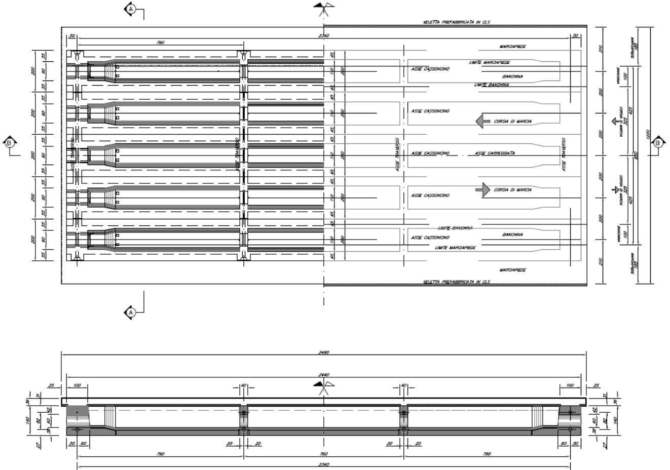
Figura 2 – Sezione, pianta e vista impalcato del Cavalcaferrovia
