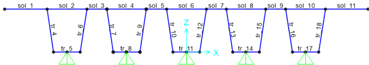
Figura 22 – Modello 2D agli E.F.
