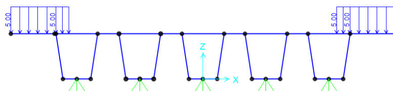
Figura 32 – Assegnazione carichi su modello agli E.F. - Schema 5 (Q3)
