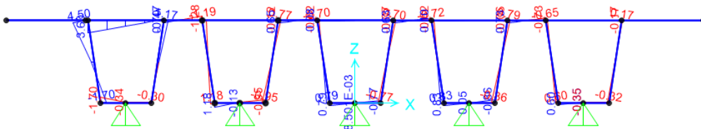
Moment 3-3 Diagram (urto)
