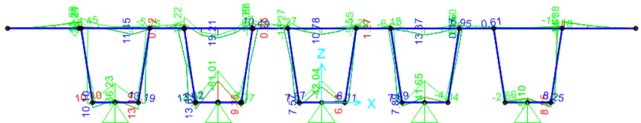
Figura 37 – Momento flettente - Combinazione di involucro SLE-Frequente e SLE-Rara
