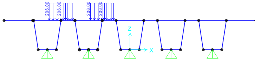
Figura 29 – Assegnazione carichi su modello agli E.F. - Schema 2 - Disposizione 1 (Q2-1)
