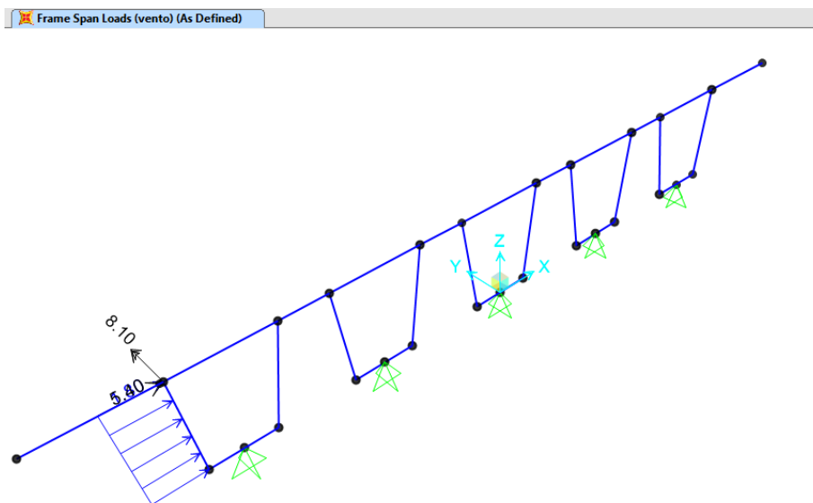
Figura 34 – Assegnazione carichi su modello agli E.F. - Vento (Q5)
