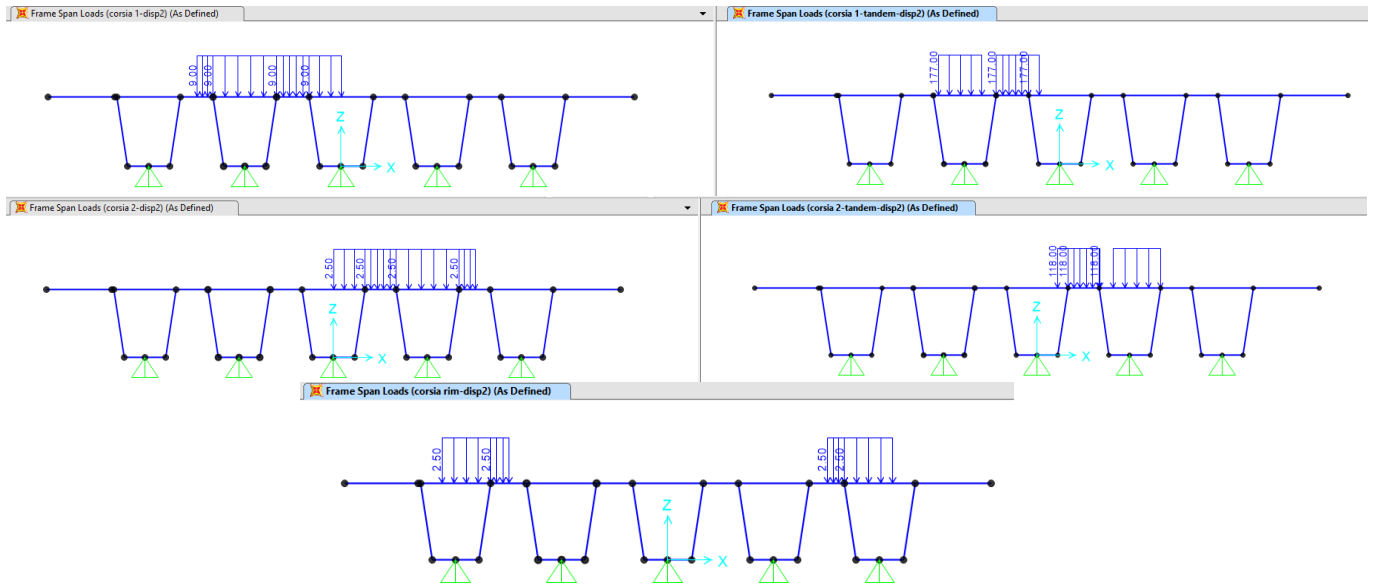
Figura 27 – Assegnazione carichi su modello agli E.F. - Schema 1 - Disposizione 2 - Tandem (Q1-2-1)
