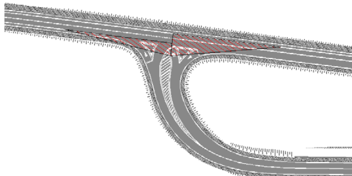
Figura 12- Triangoli visibilità segnale stop
