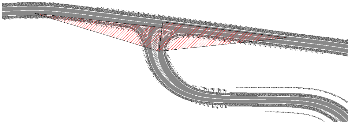
Figura 13- Triangoli visibilità segnale dare precedenza
