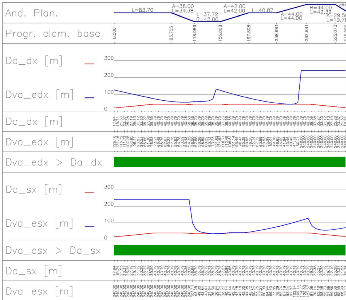
Figura 11 – Diagramma di visibilità post allargamenti
