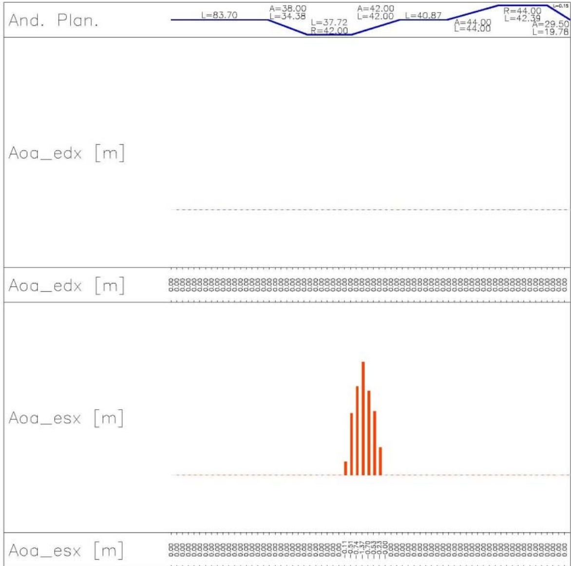
Figura 10 – Diagramma di arretramento ostacoli ante allargamenti
