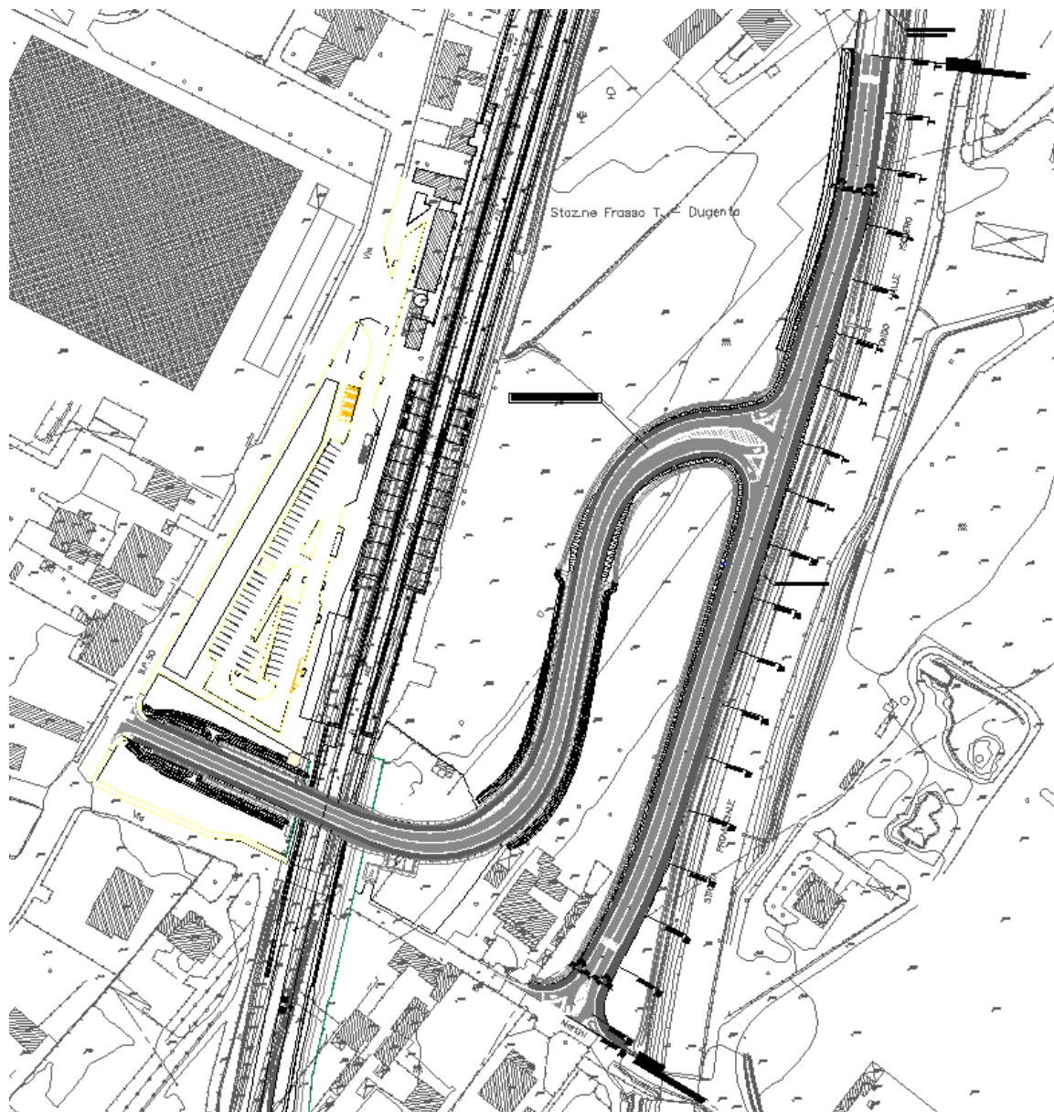
Figura 2 - Stato di progetto
