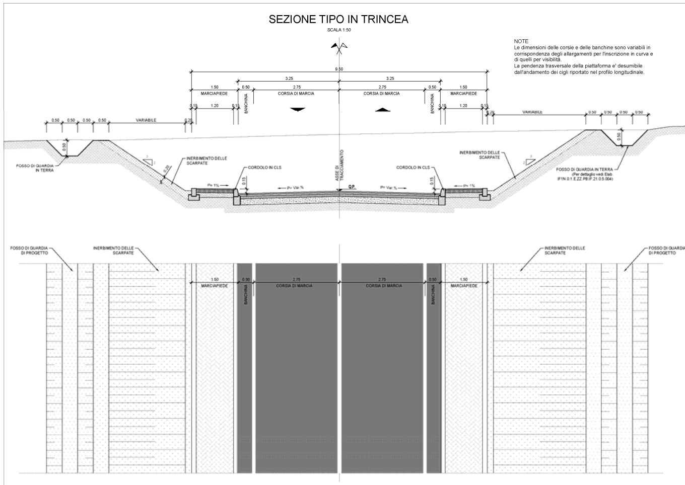
Figura 4 – Sezione e pianta tipo in trincea
