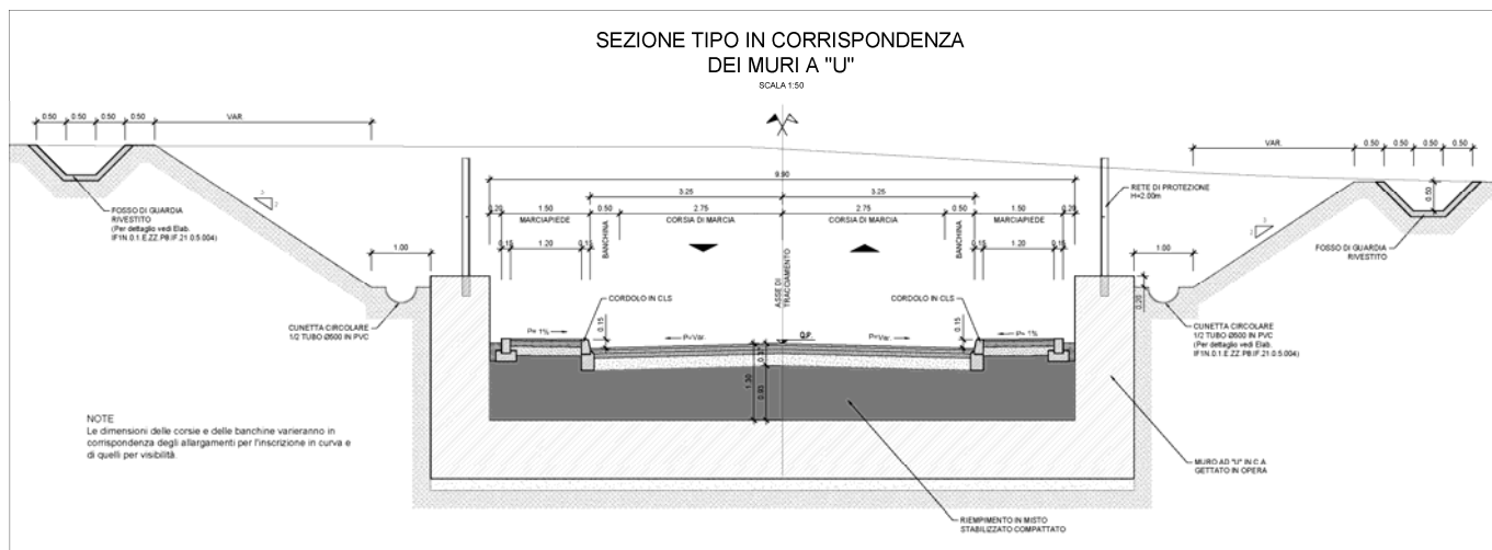
Figura 6 – Sezione e pianta tipo in corrispondenza muri a U
