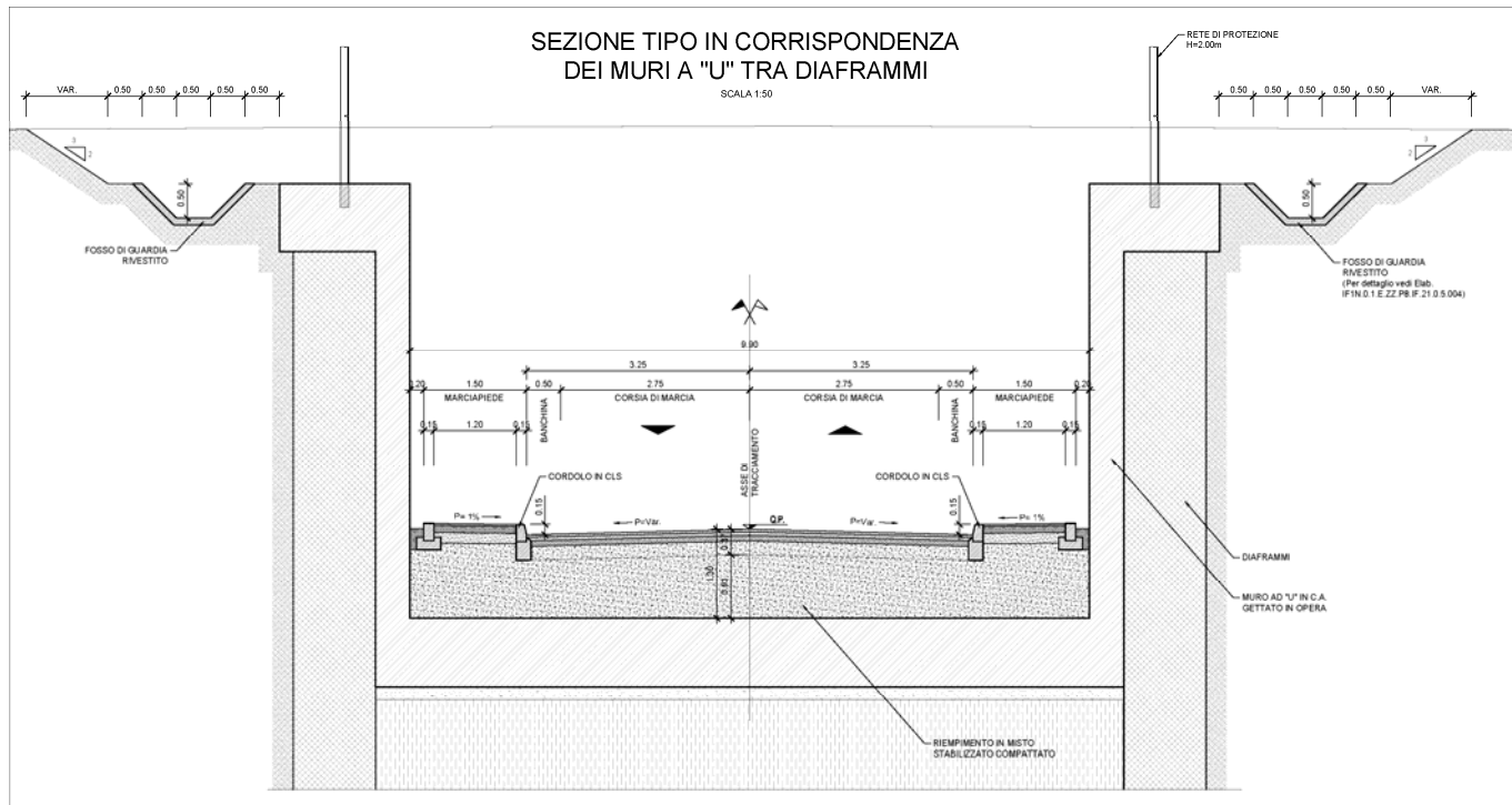
Figura 5 – Sezione e pianta tipo in corrispondenza diaframmi
