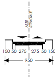
Figura 3 – Sezione stradale tipo F (ambito urbano)
