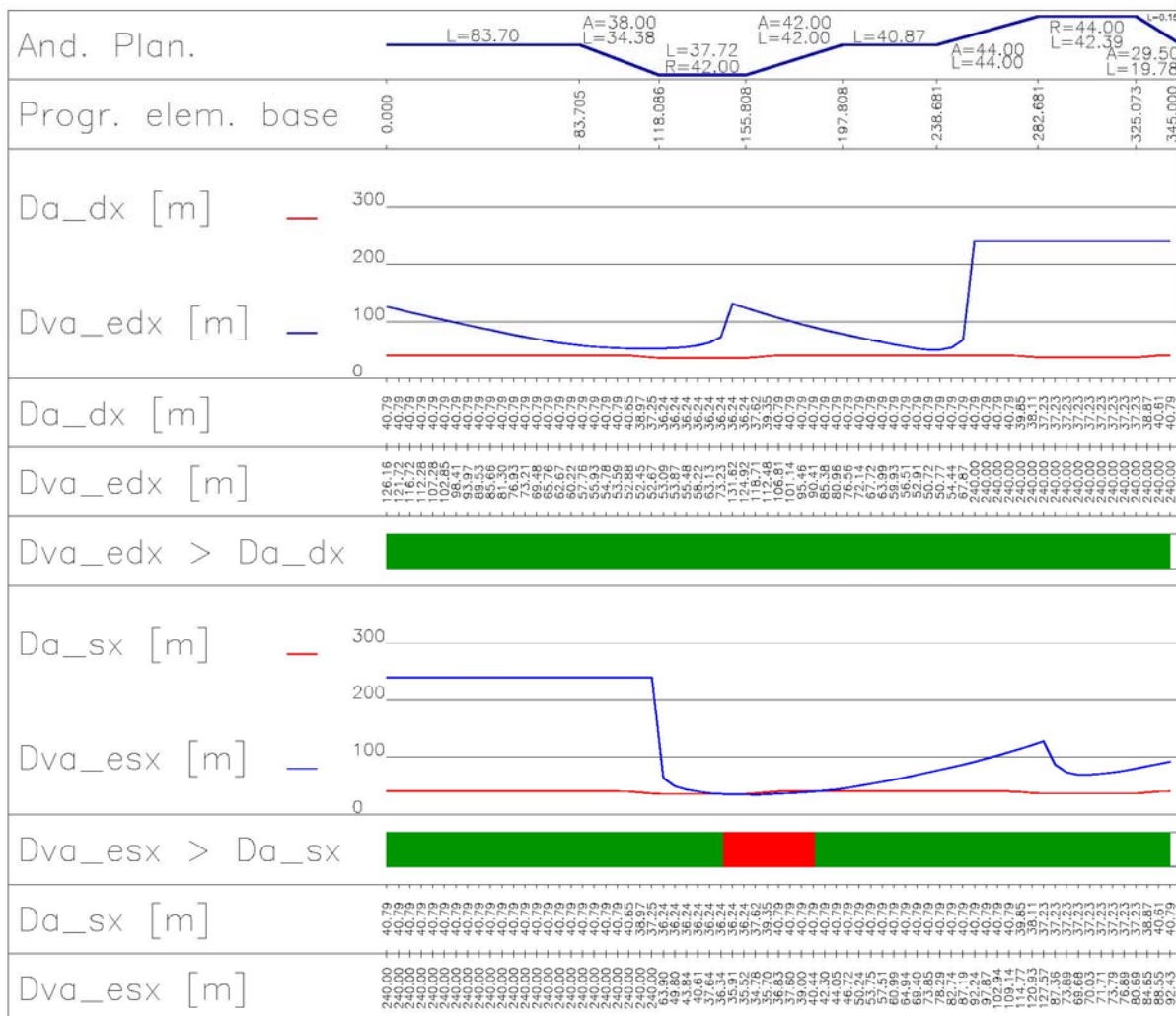
Figura 9 – Diagramma di visibilità ante allargamenti
