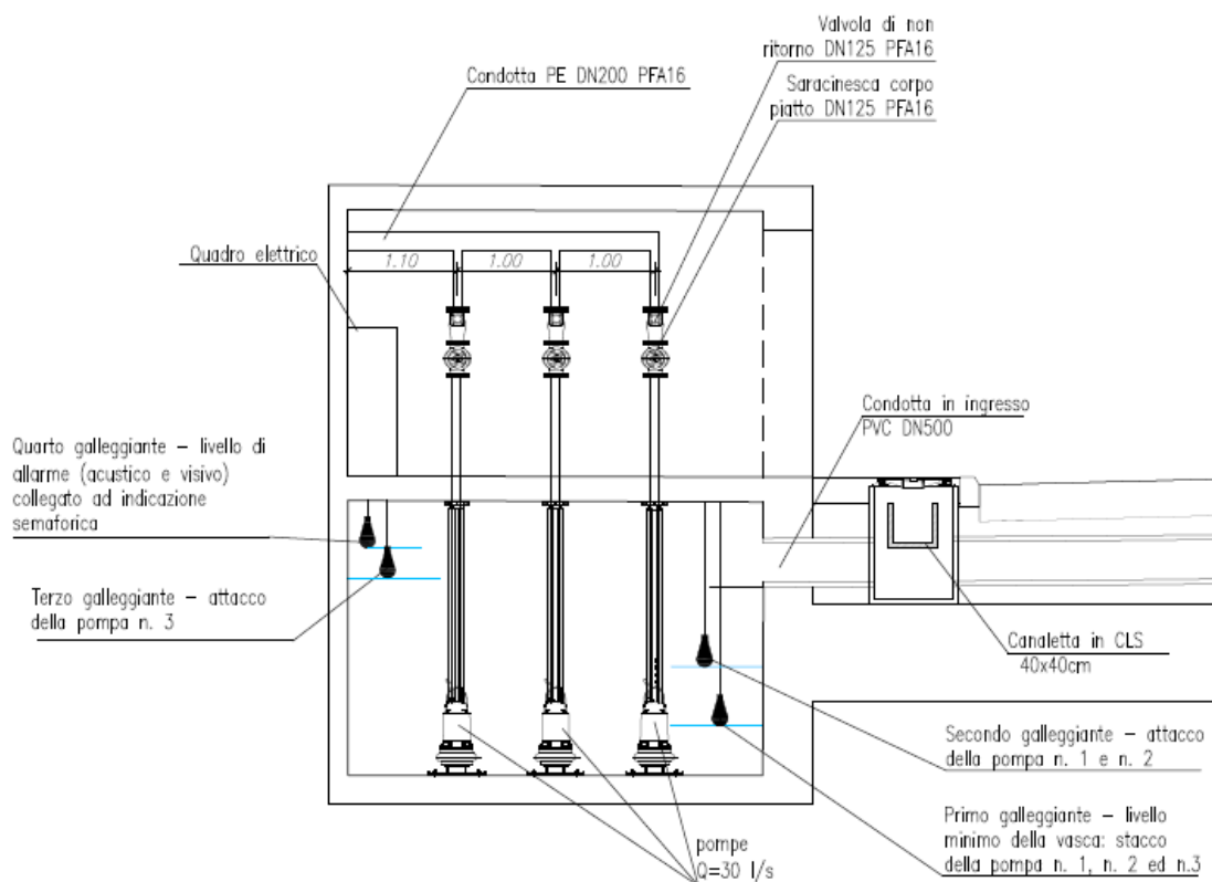
Figura 4.1: Vasca di sollevamento del Sottovia di Dugenta
