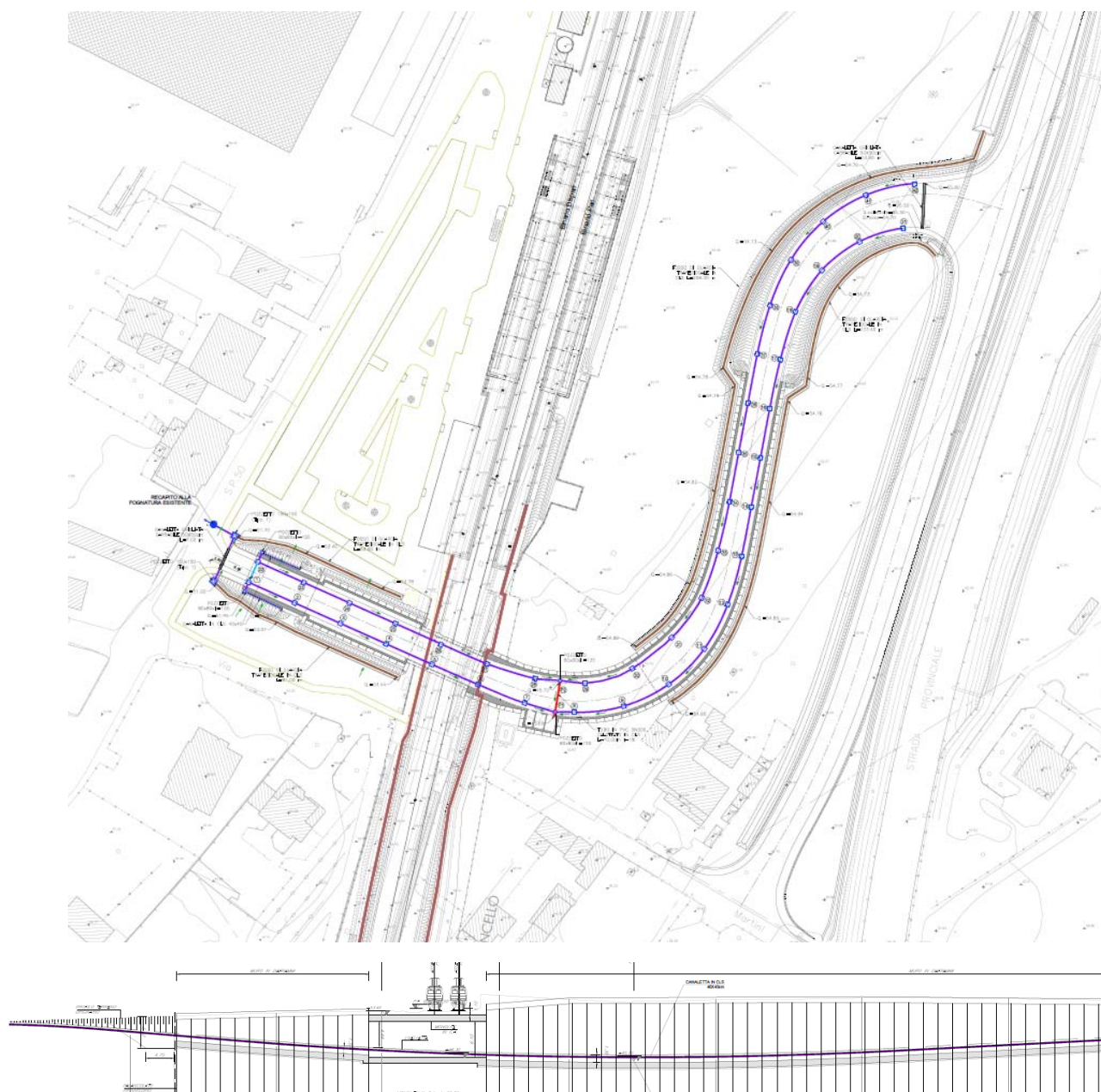
Figura 4.2: Planimetria e profilo del sottovia della Stazione di Dugenta.
