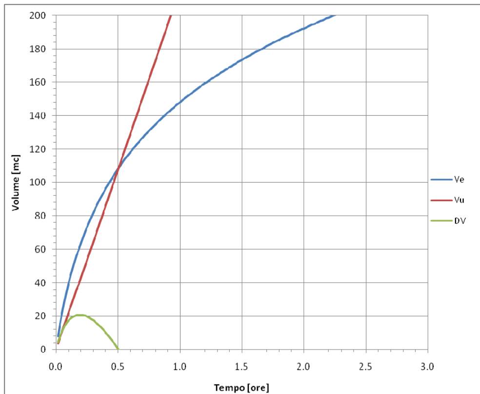
Figura 4.3: Andamento del volume teorico accumulato nella vasca di laminazione al variare del tempo di pioggia per un tempo di ritorno di 25 anni.
