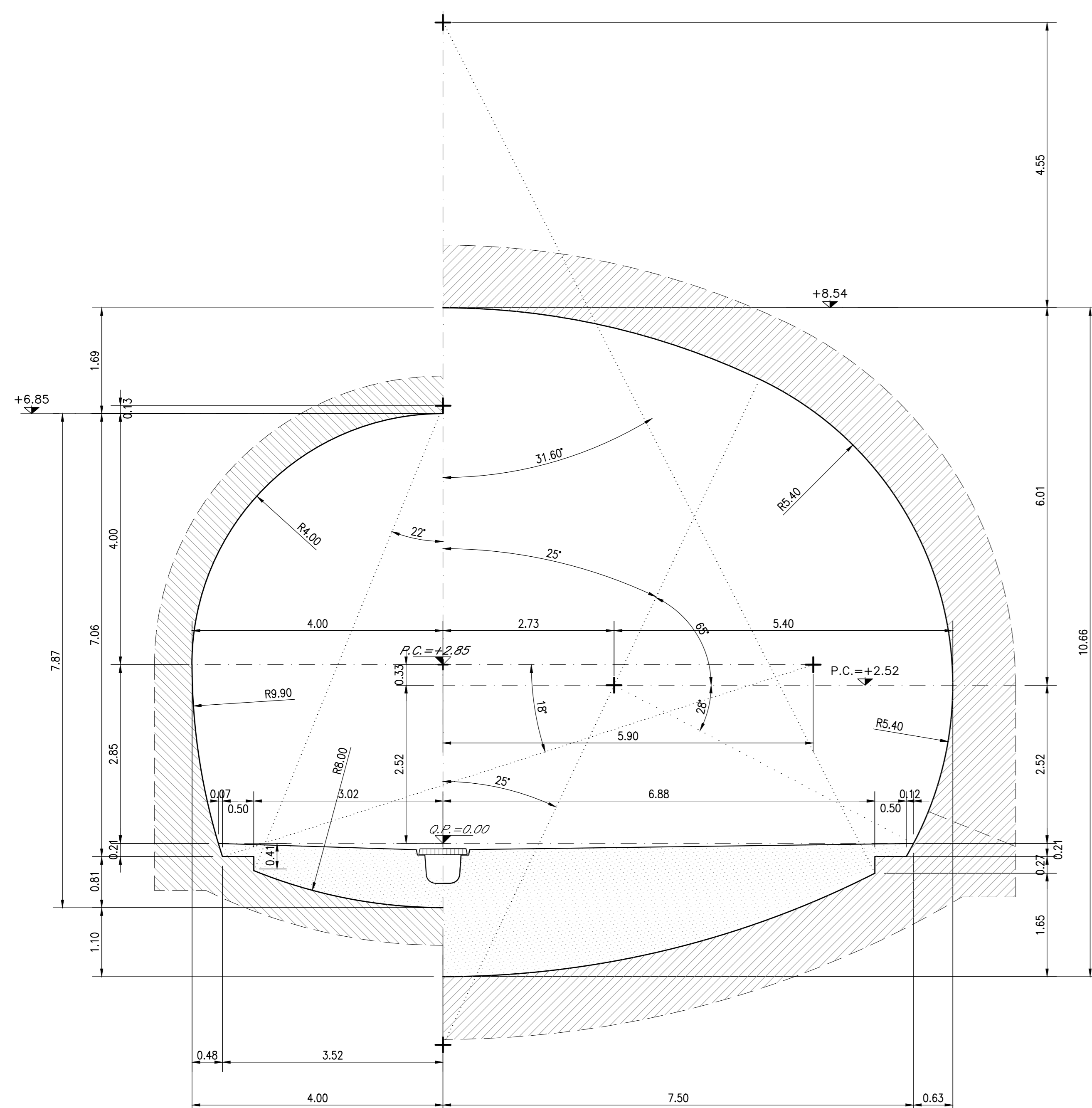
SEZIONE DI TRANSIZIONE 1/2 SEZIONE Scala 1:50 (sezione minima)
