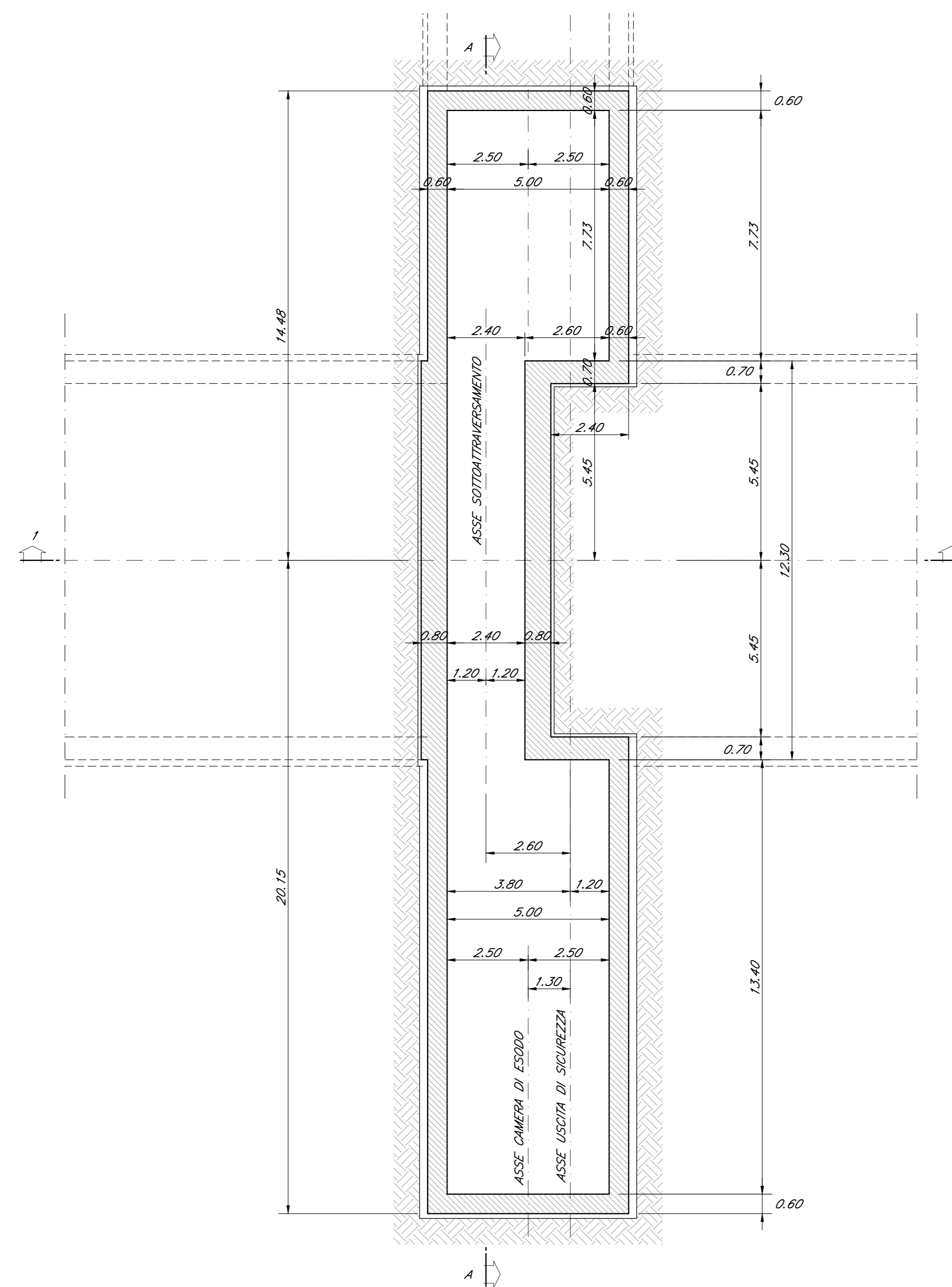
PIANTA FONDAZIONI scala 1:100
