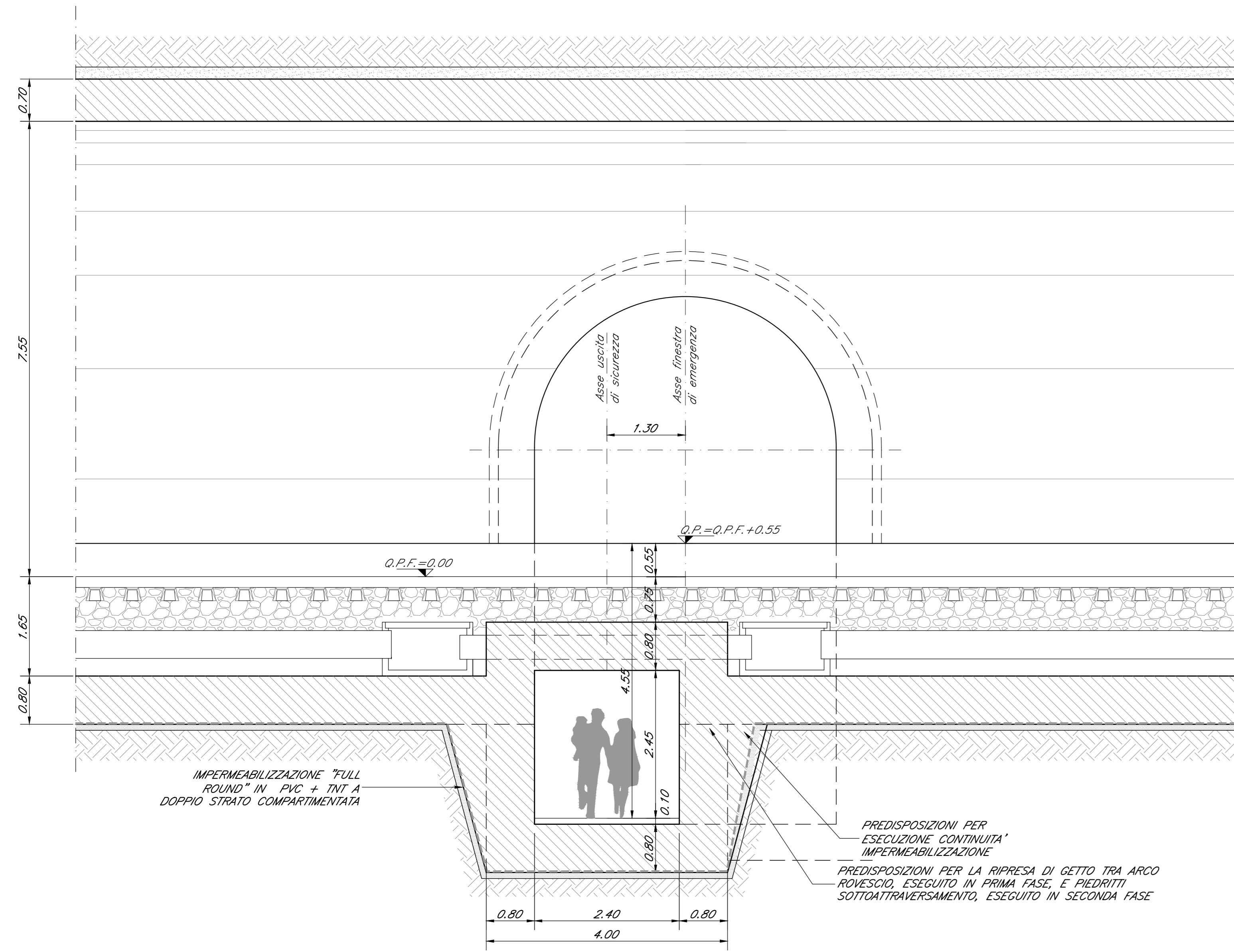
SEZIONE 1-1 scala 1:50
