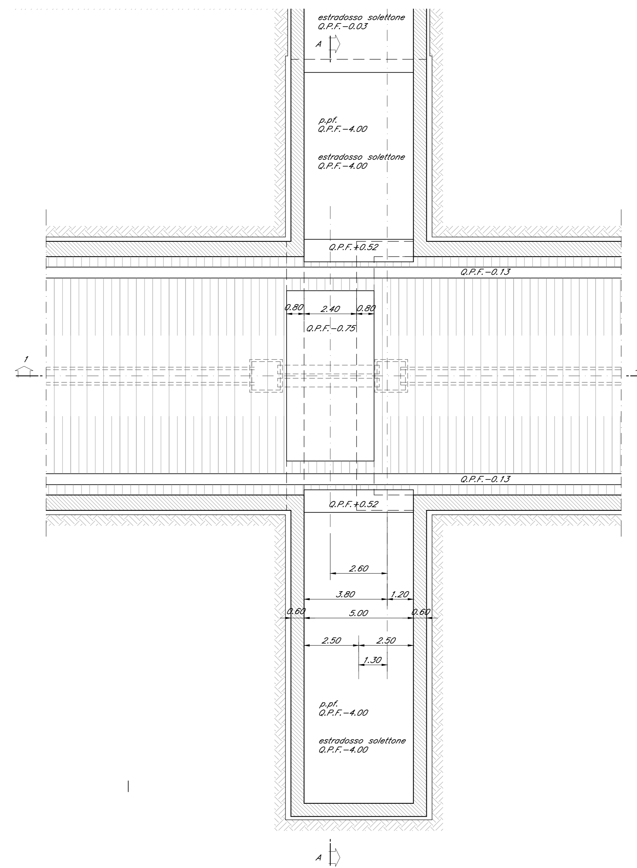
PIANTA ARCO ROVESCIO scala 1:100
