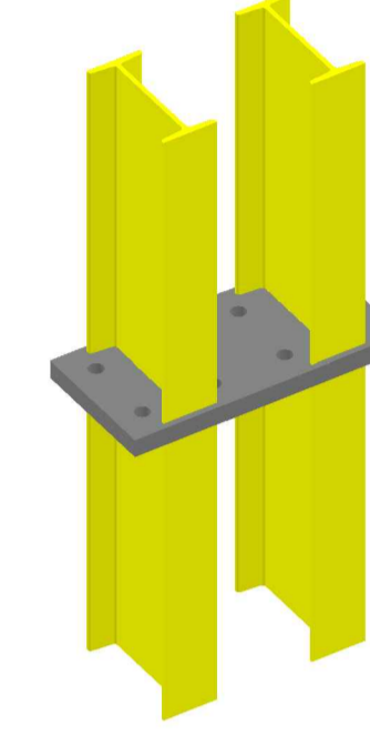
VISTA ASSONOMETRICA PARTICOLARE "02"
