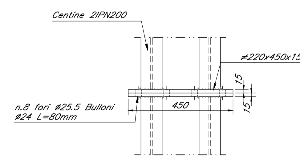
PARTICOLARE "02" scala 1:10
