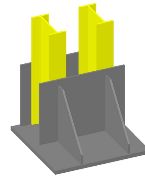
VISTA ASSONOMETRICA PARTICOLARE "01"
