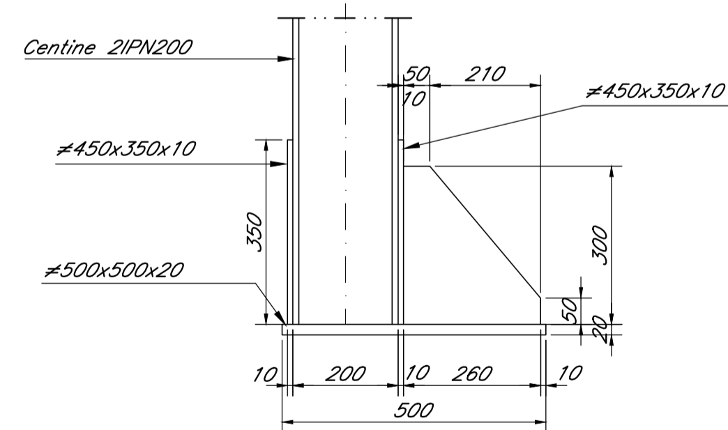
PARTICOLARE "01" scala 1:10
