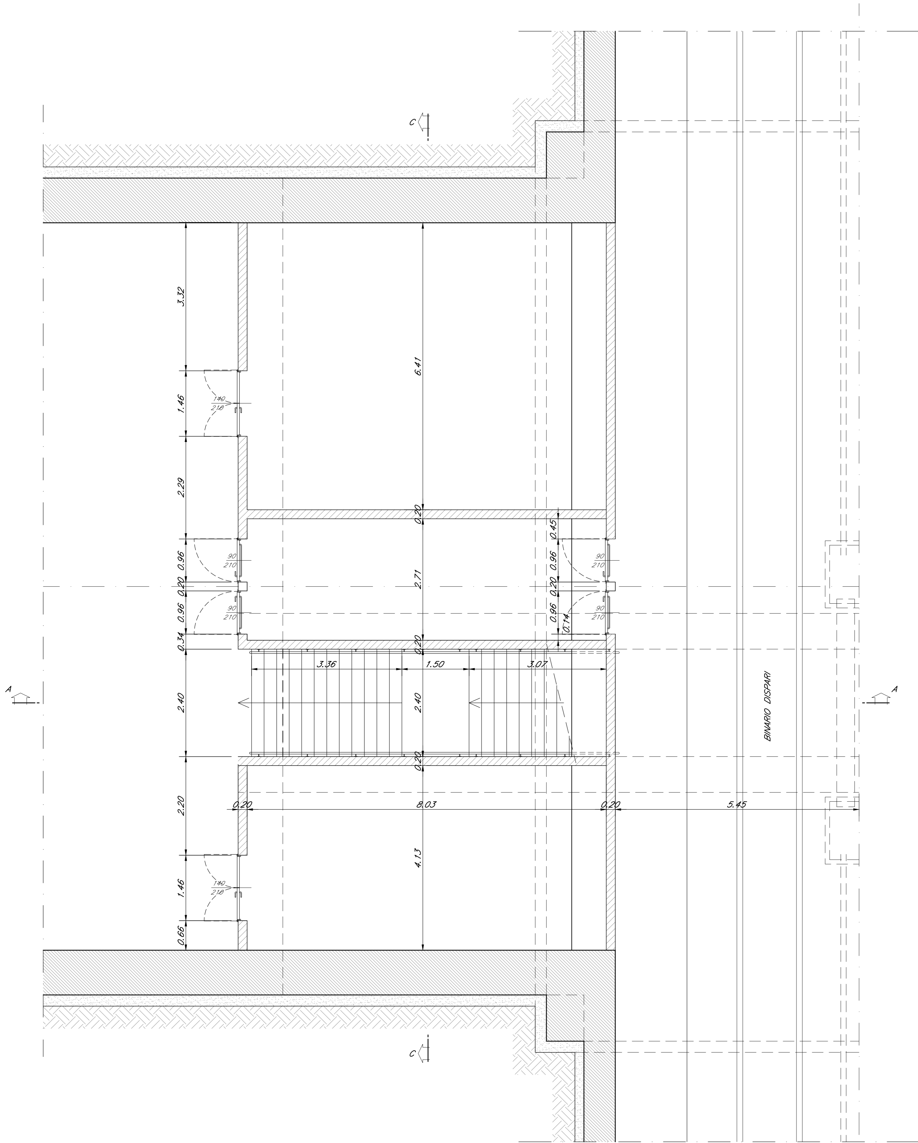
ALLESTIMENTO - SEZIONE B-B scala 1:50
