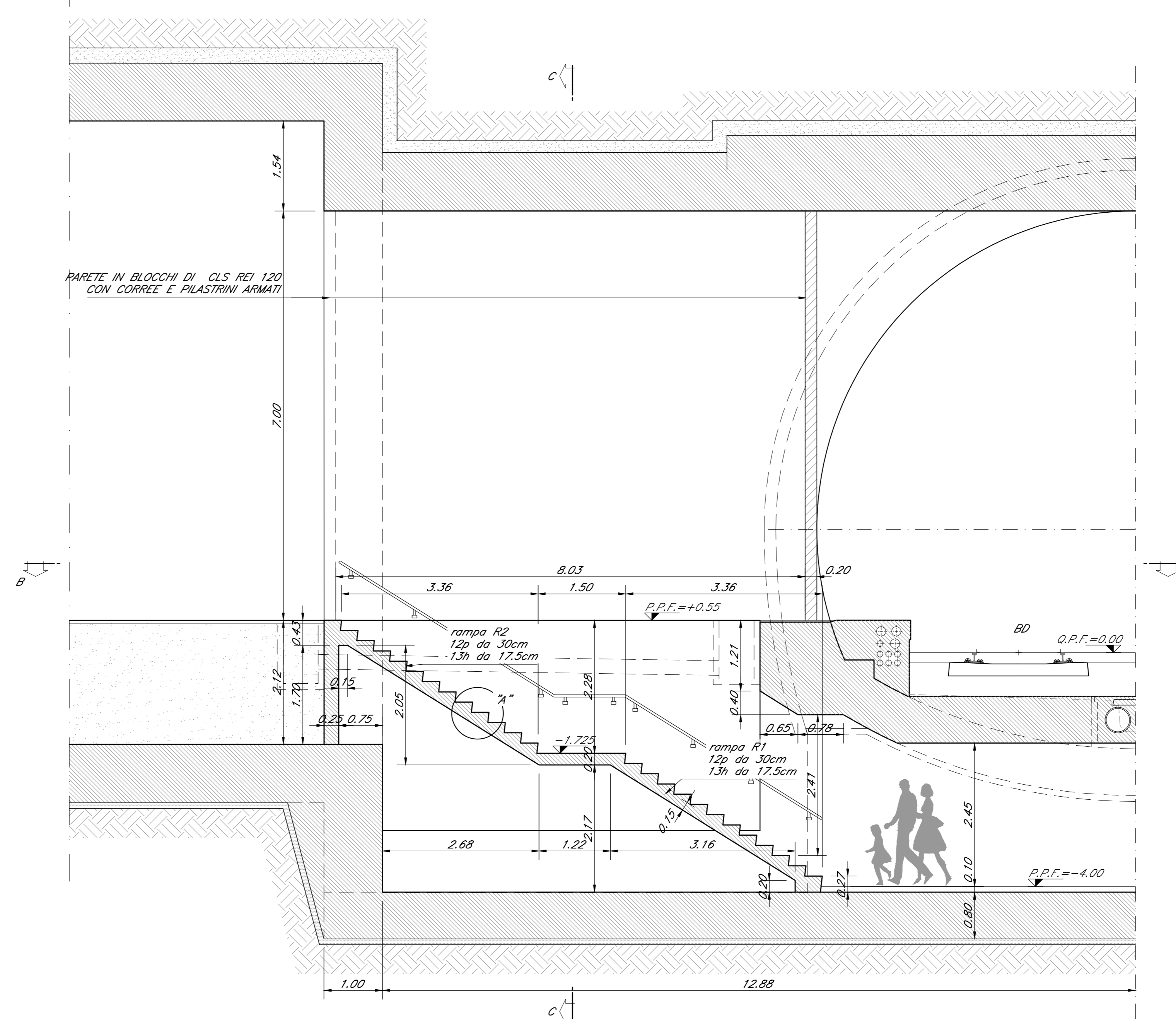
ALLESTIMENTO - SEZIONE A-A scala 1:50
