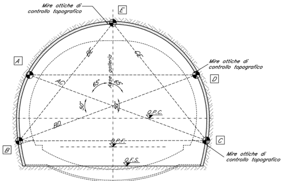
Figura 7: distribuzione delle mire ottiche sulla sezione di scavo del camerone di segnalamento
