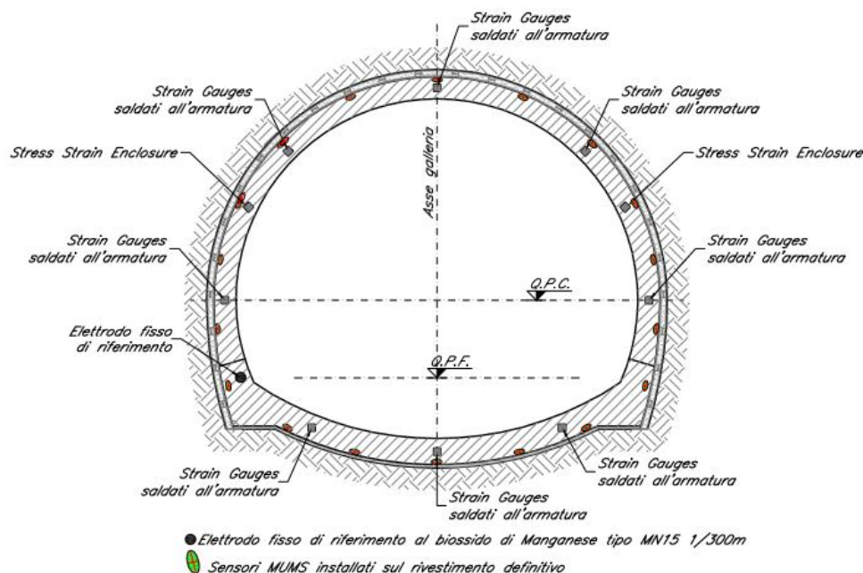
Figura 10: strumentazione per il monitoraggio del rivestimento definitivo
