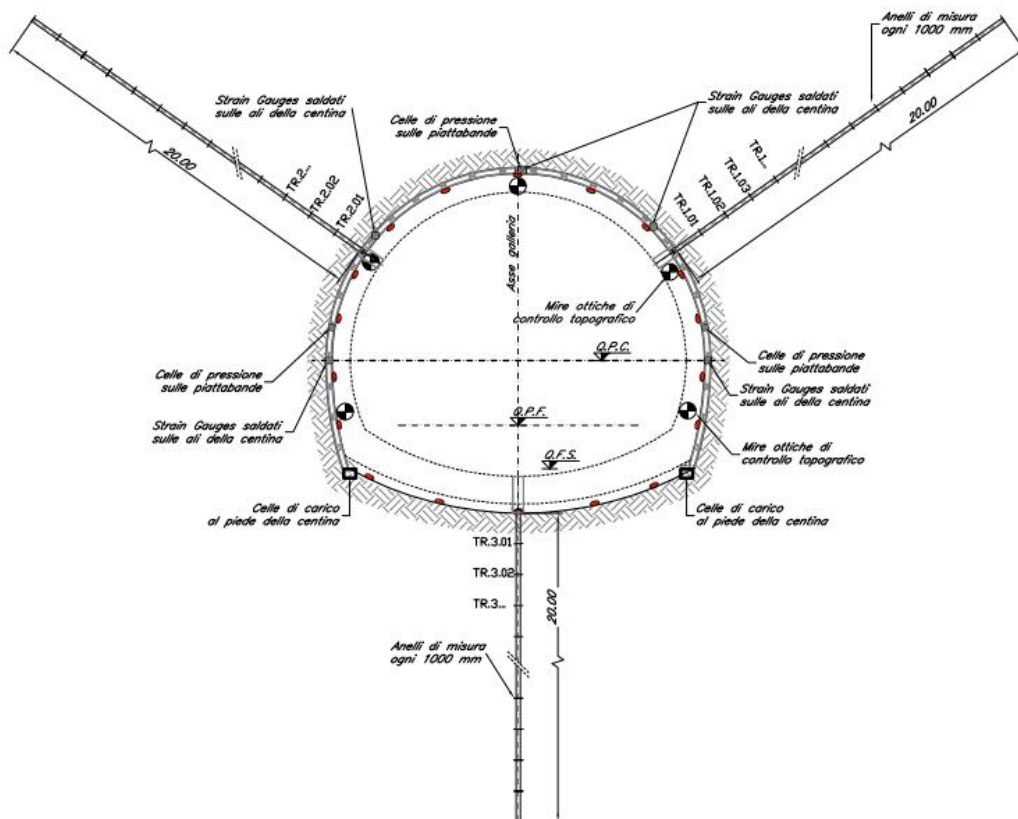
Figura 9: sezione tipologica 2 di monitoraggio del sostegno di prima fase
