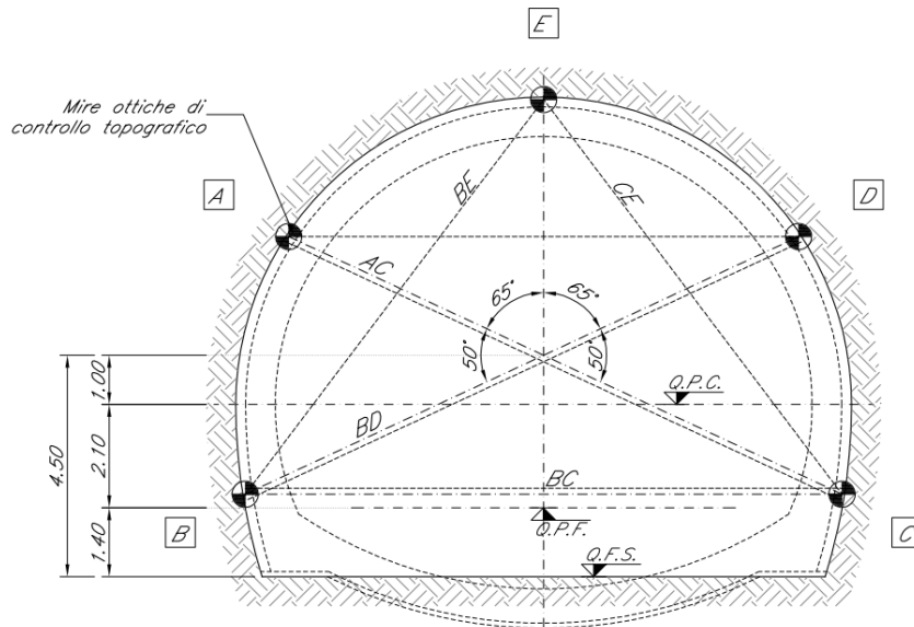
Figura 6: distribuzione delle mire ottiche sulla sezione di scavo
