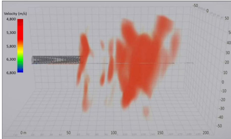
Figura 5: risultati di una indagine TSP condotta in avanzamento
