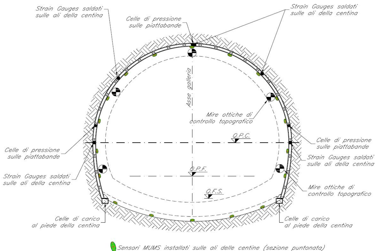
Figura 8: sezione tipologica 1 di monitoraggio del sostegno di prima fase
