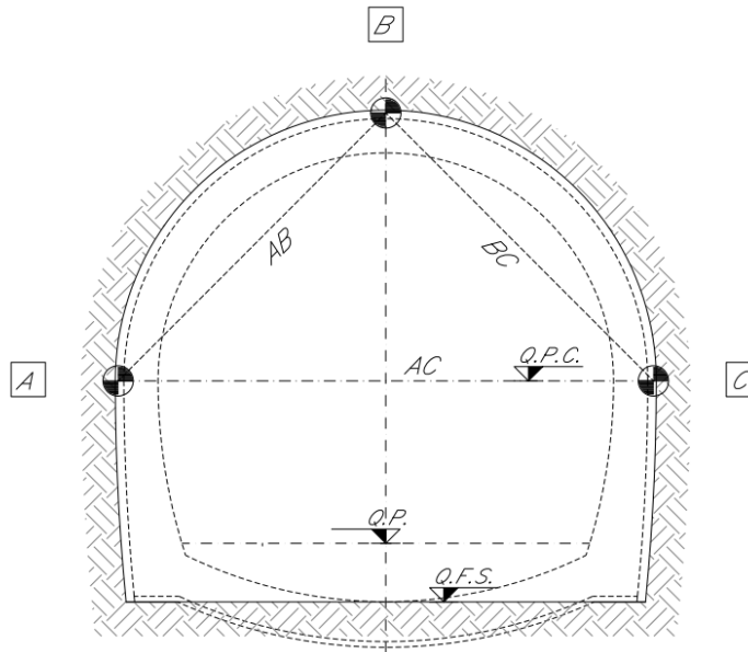
Figura 4: distribuzione delle mire ottiche sulla sezione di scavo
