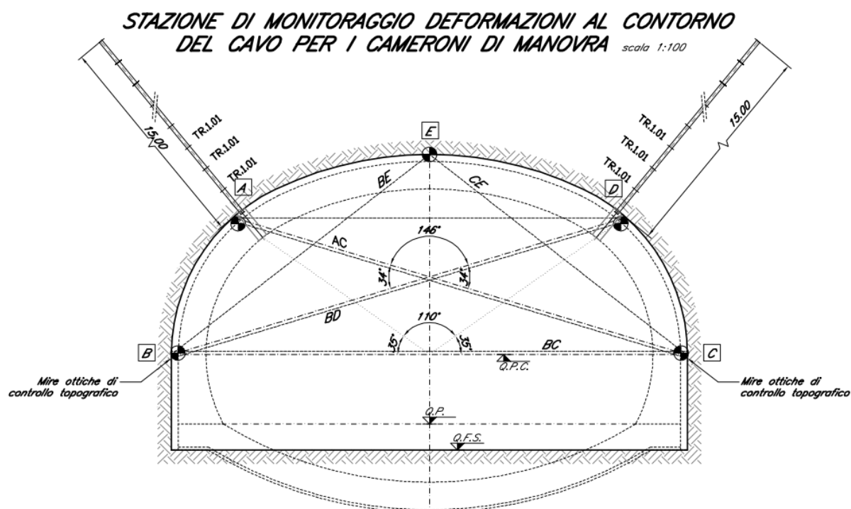
Figura 5: strumentazione per il monitoraggio del sostegno di prima fase nei cameroni di manovra
