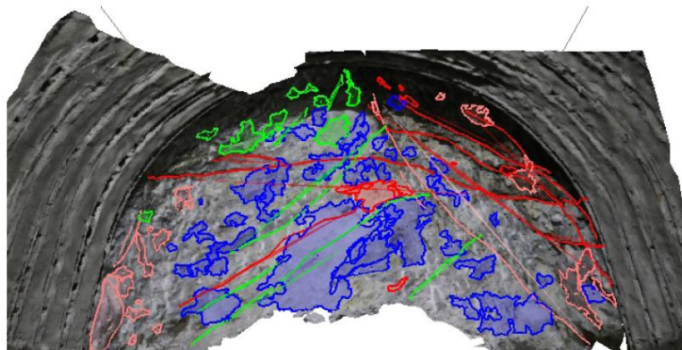
Figura 2: Esempio di un rilievo geomeccanico del fronte di scavo mediante Shapematrix 3D
