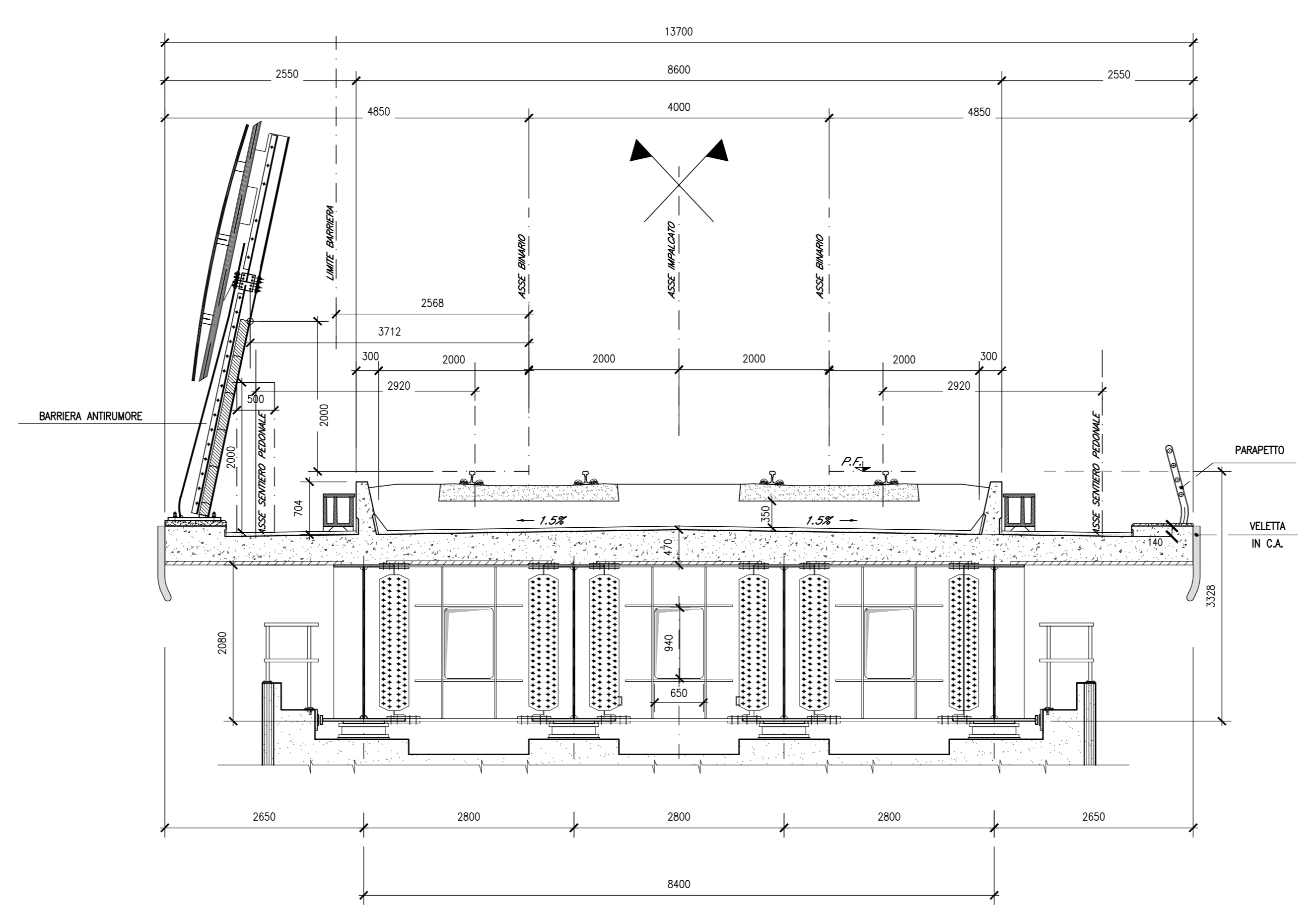
SEZIONE DI TESTATA (Scale 1:50)
