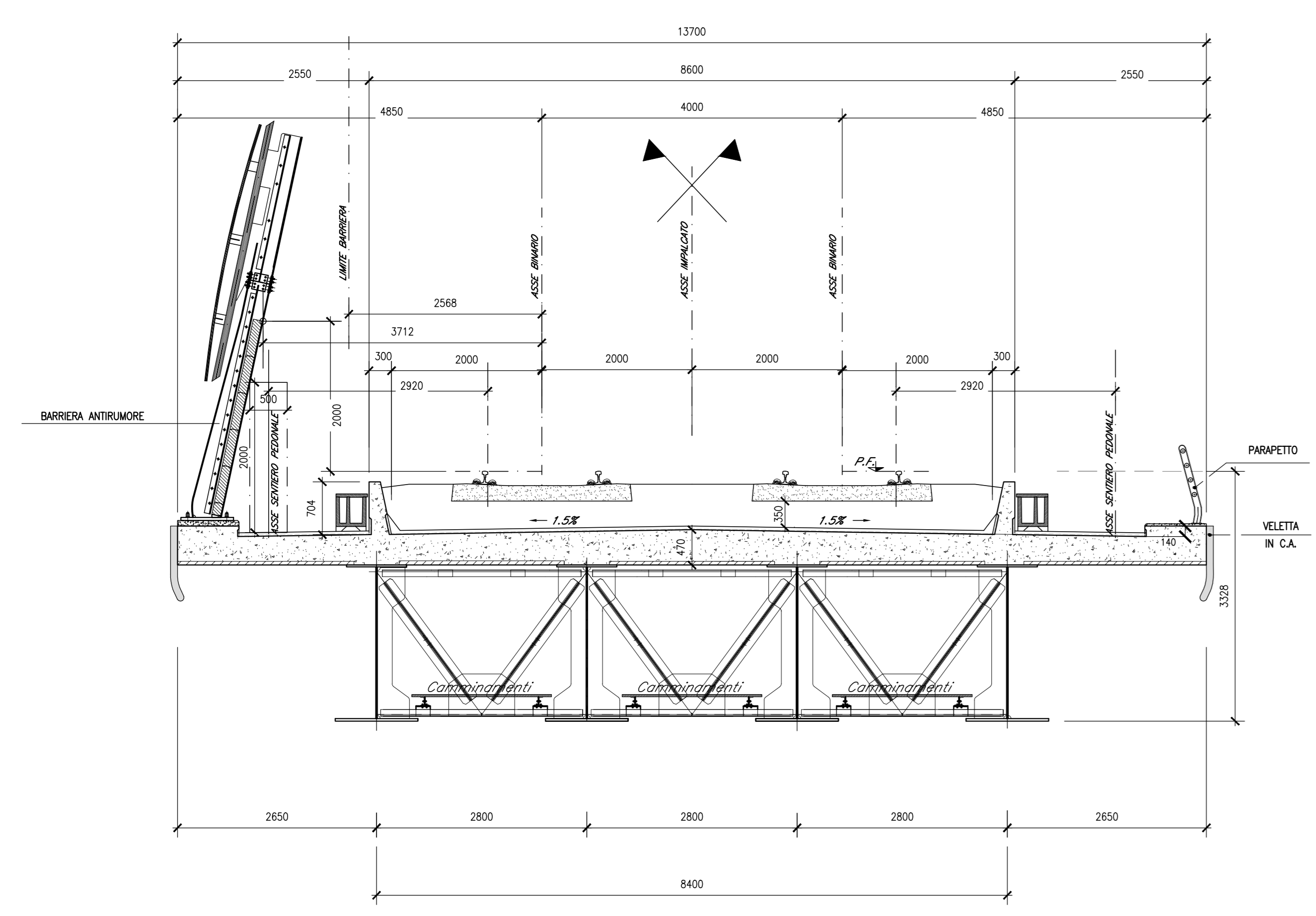
SEZIONE DIAFRAMMA (Scale 1:50)
