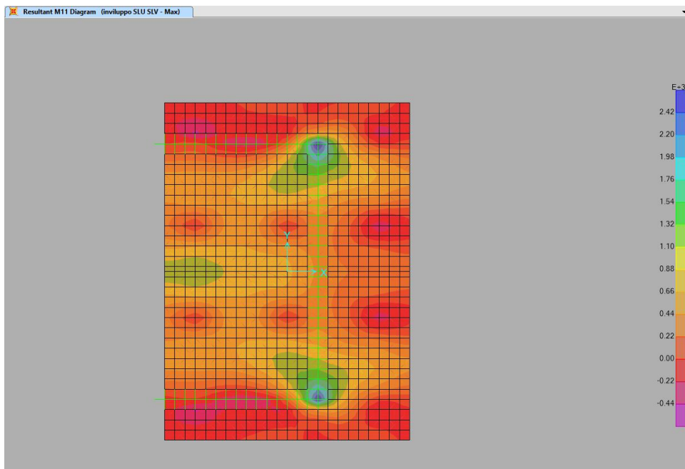
Figura 9: involucro SLU e SLV sollecitazioni M11
