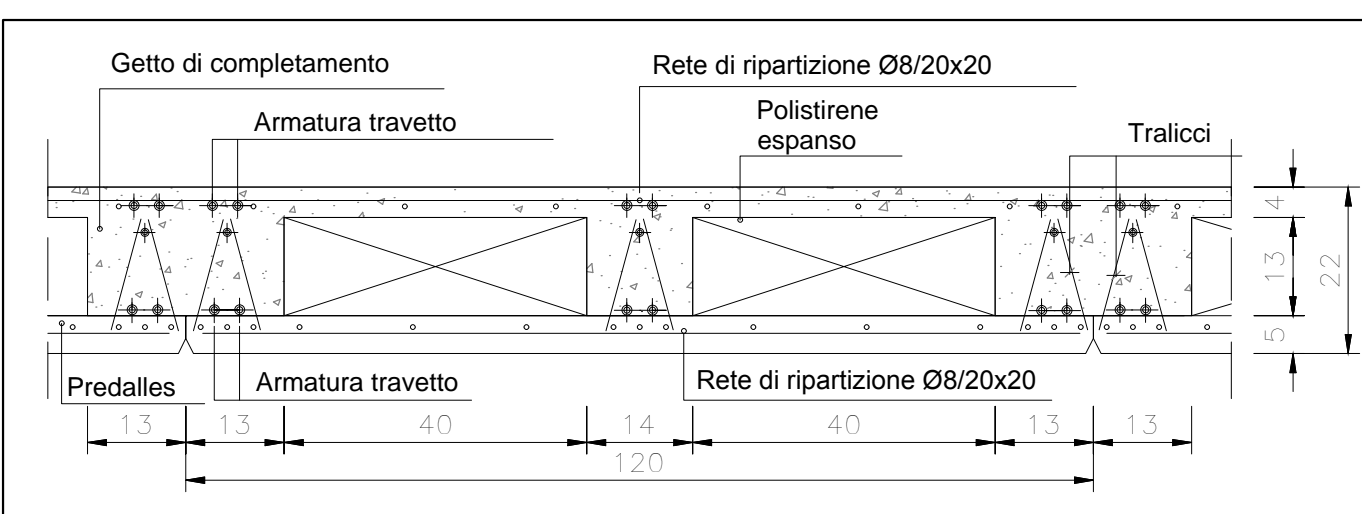
Particolare Solaio Copertura 1:10
