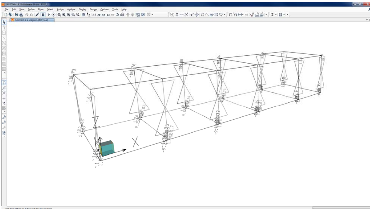
Figura 7-6 Modello di calcolo – Diagramma M22 – Combinazione “COMB_INV_SLV”.
