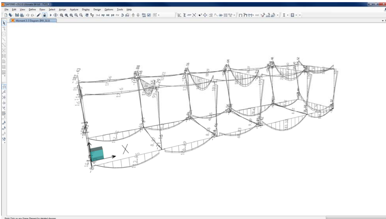
Figura 7-3 Modello di calcolo – Diagramma M33 – Combinazione “COMB_INV_SLU”.
