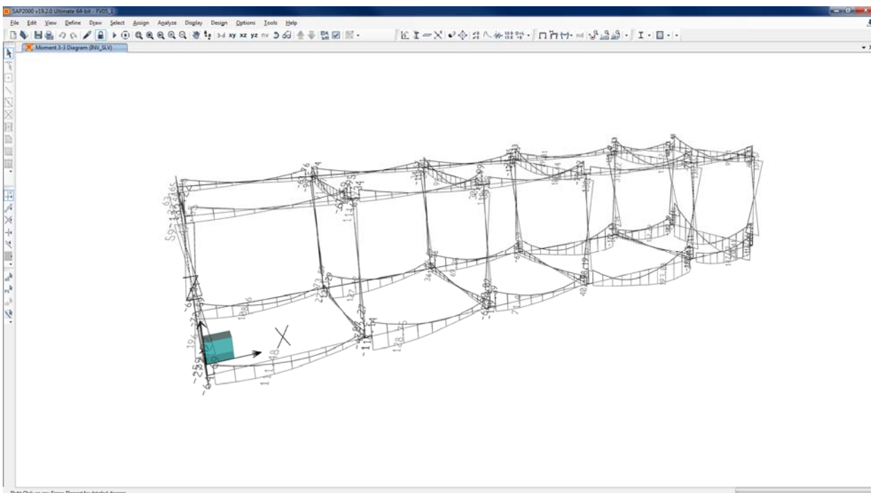
Figura 7-4 Modello di calcolo – Diagramma M33 – Combinazione “COMB_INV_SLV”.
