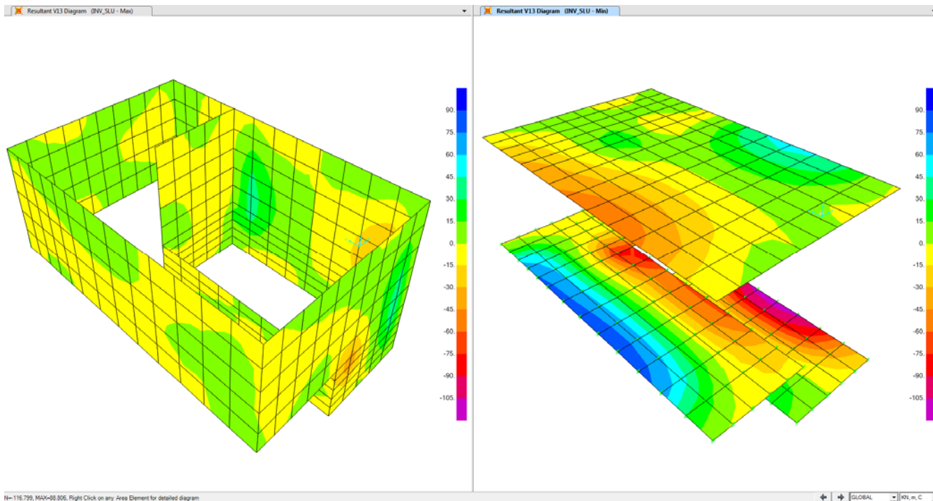
Figura 7-16 Modello di calcolo – Diagramma V13 – Combinazione “COMB_INV_SLU”.
