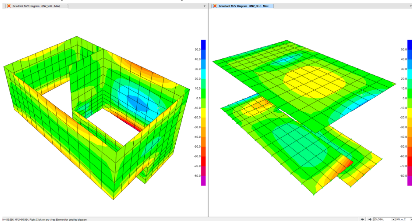
Figura 7-15 Modello di calcolo – Diagramma M22 – Combinazione “COMB_INV_SLU”.
