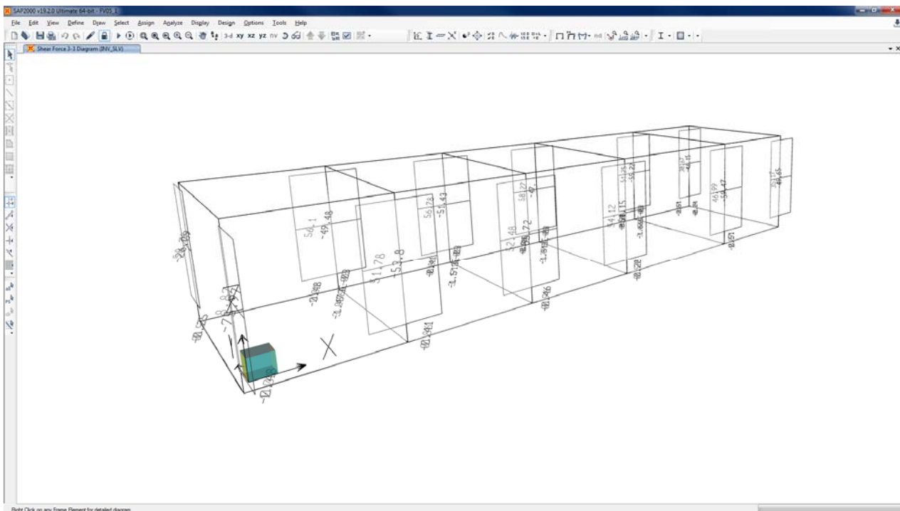
Figura 7-10 Modello di calcolo – Diagramma V33 – Combinazione “COMB_INV_SLV”.
