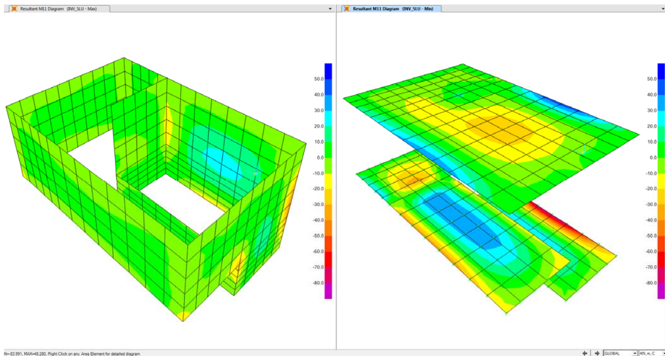
Figura 7-14 Modello di calcolo – Diagramma M11 – Combinazione “COMB_INV_SLU”.
