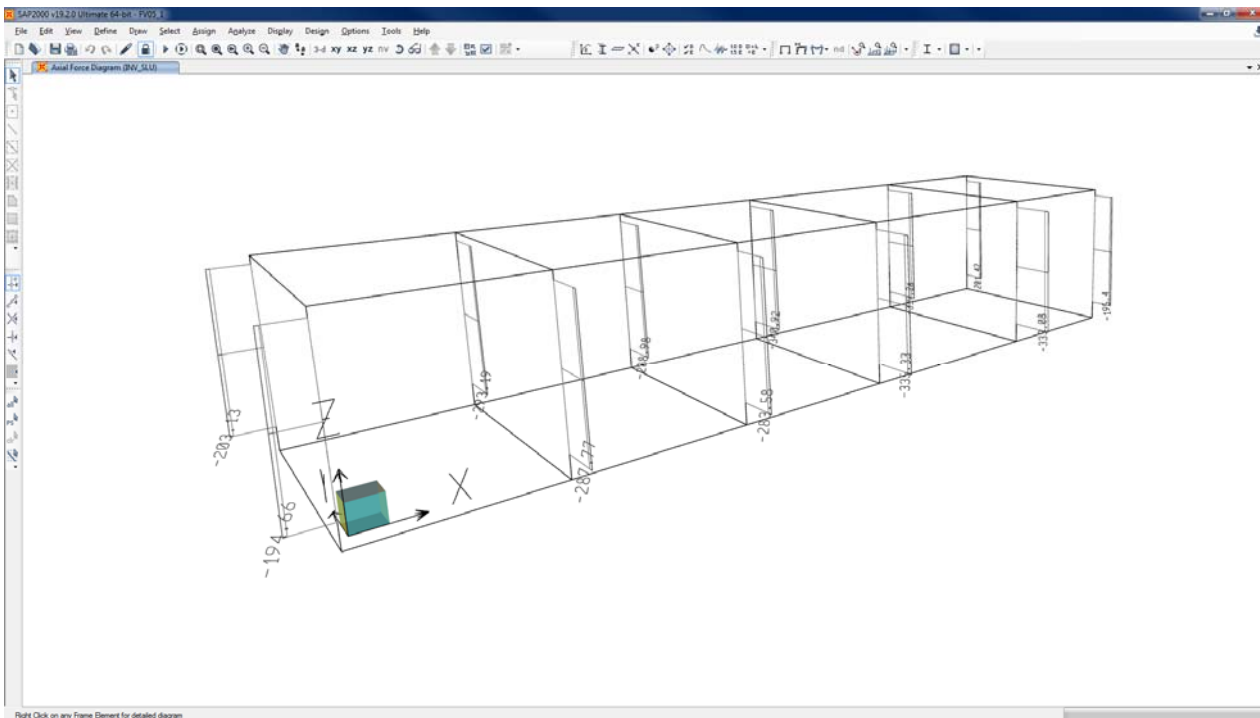
Figura 7-11 Modello di calcolo – Diagramma N – Combinazione “COMB_INV_SLU”.
