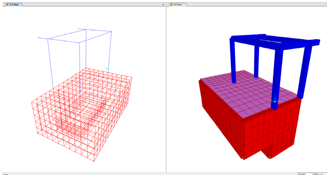
Figura 7-13 Modello di calcolo stazione di pompaggio – Vista fil di ferro ed estrusa del modello.
