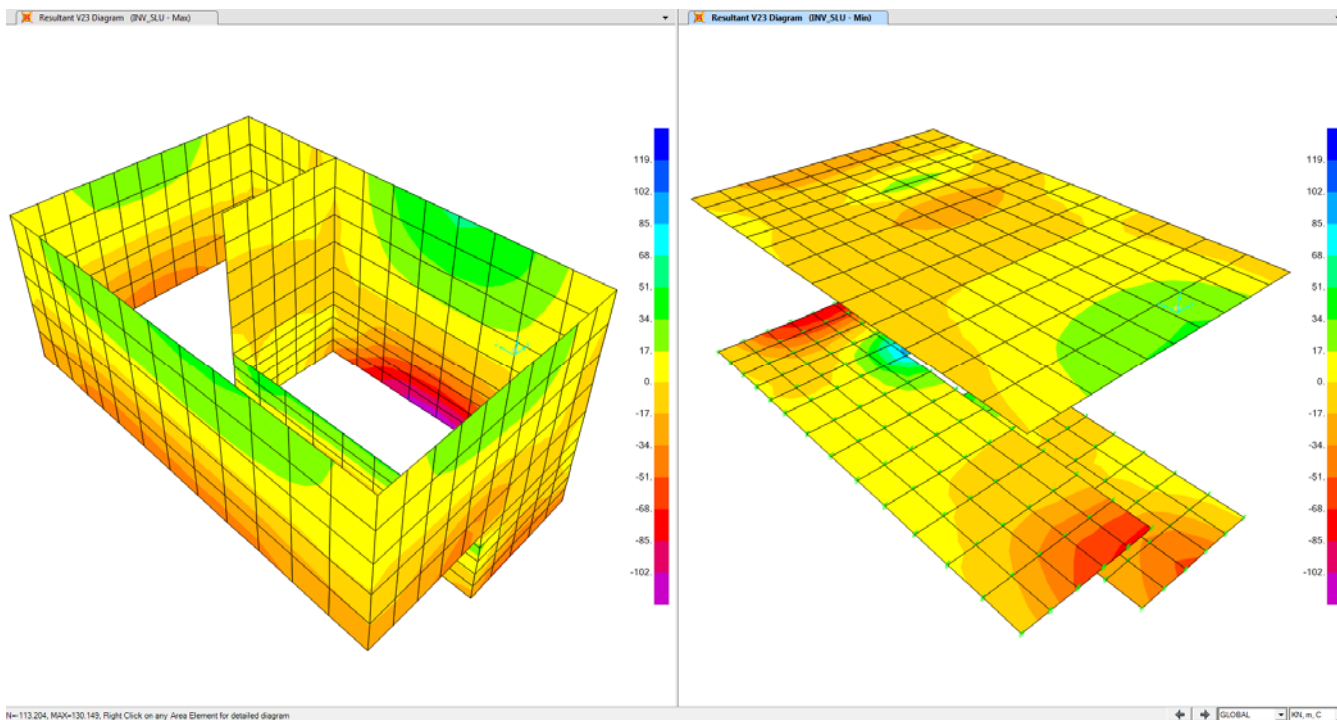
Figura 7-17 Modello di calcolo – Diagramma V23 – Combinazione “COMB_INV_SLU”.
