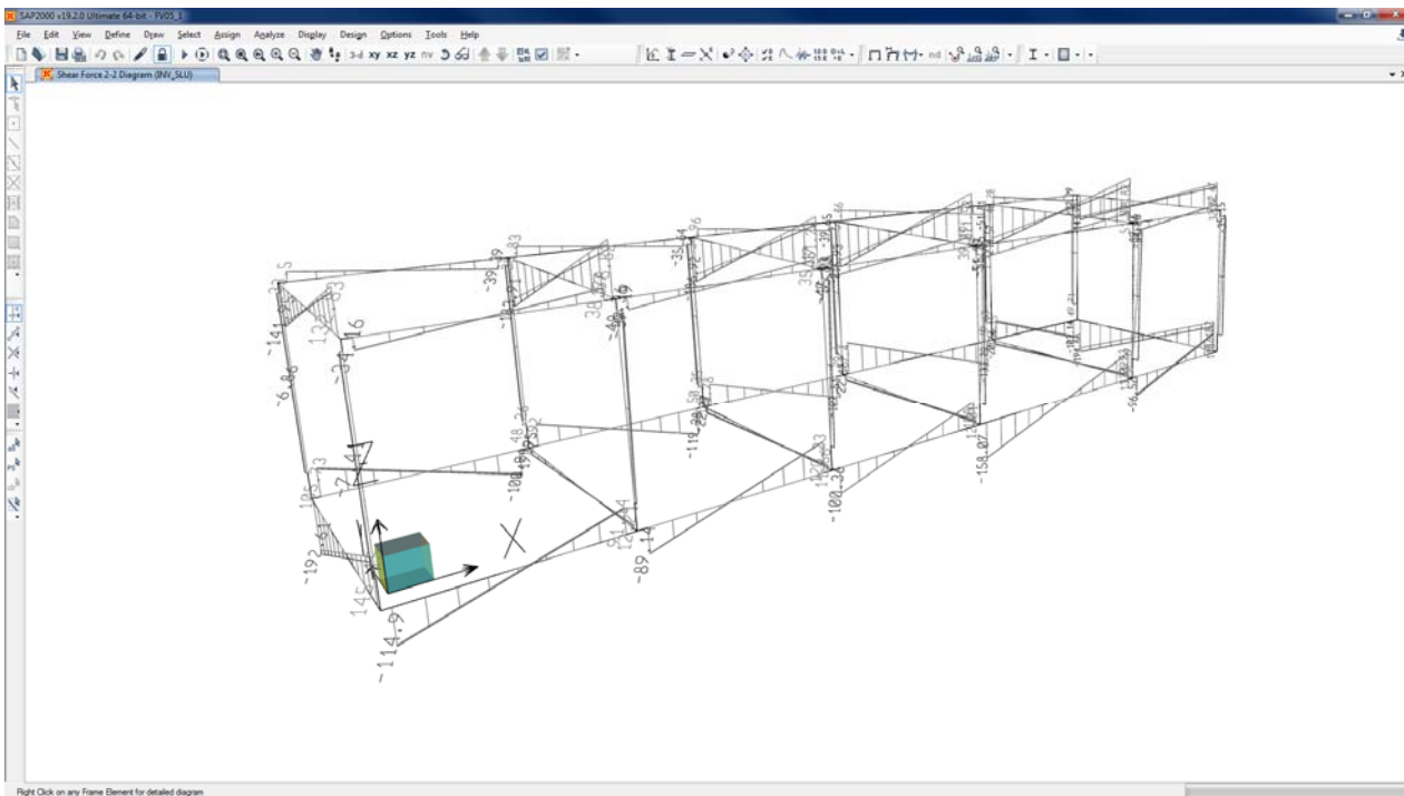
Figura 7-7 Modello di calcolo – Diagramma V22 – Combinazione “COMB_INV_SLU”.
