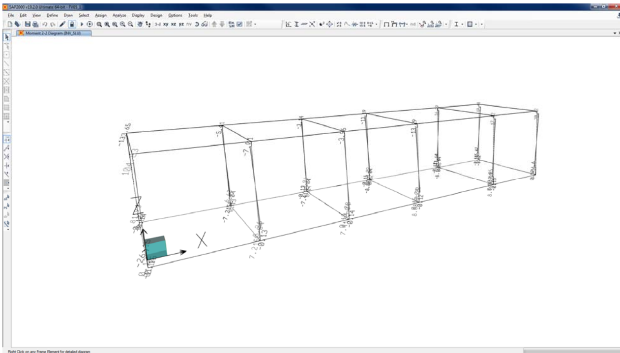
Figura 7-5 Modello di calcolo – Diagramma M22 – Combinazione “COMB_INV_SLU”.
