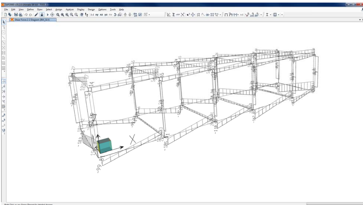
Figura 7-8 Modello di calcolo – Diagramma V22 – Combinazione “COMB_INV_SLV”.
