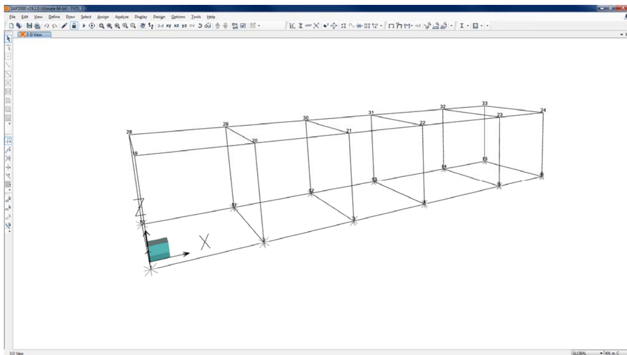
Figura 7-2 Modello di calcolo – numerazione frames e nodi.
