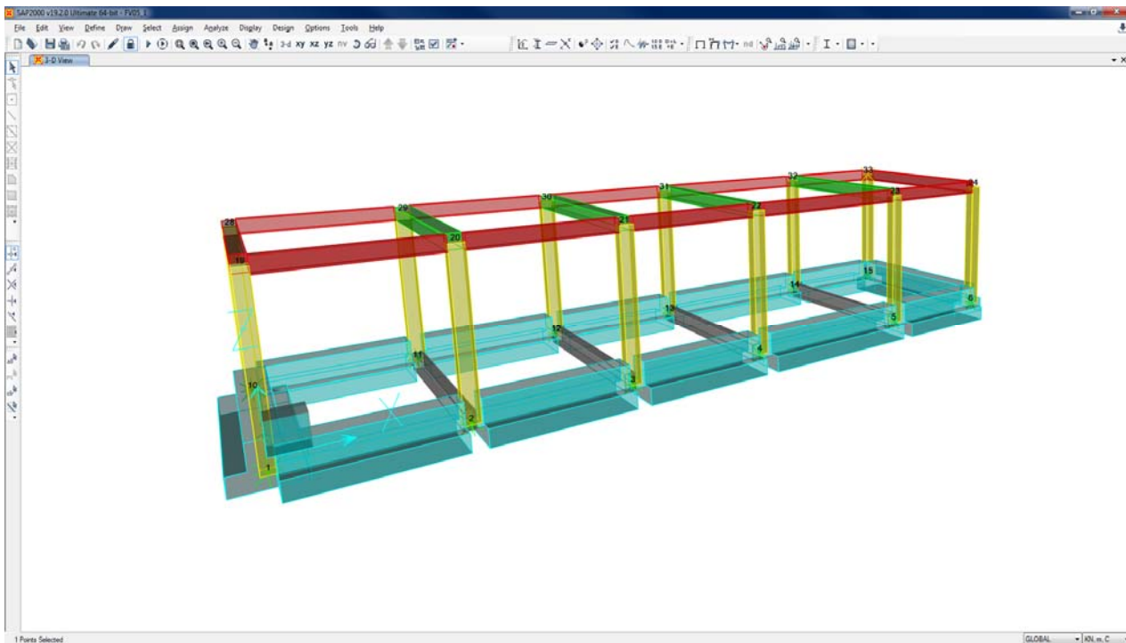
Figura 7-1 Modello di calcolo – Vista estrusa del modello.
