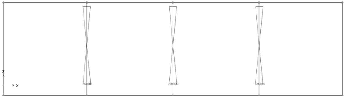
Figura 7-7 Diagramma dei momenti M2 - COMB_INV_SLU
