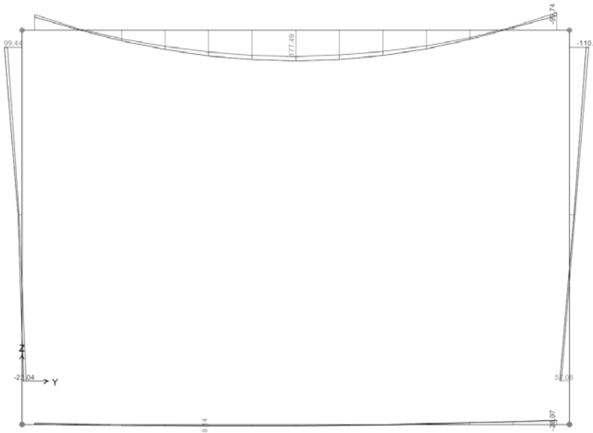
Figura 7-10 Diagramma dei momenti M3 – COMB_INV_SLU – allineamento 2.
