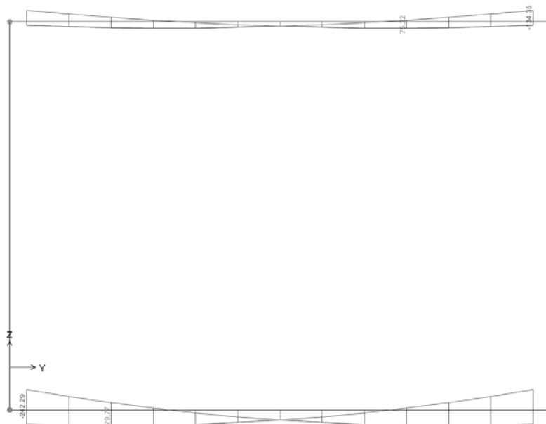
Figura 7-9 Diagramma dei momenti M3 – COMB_INV_SLV – allineamento 1.
