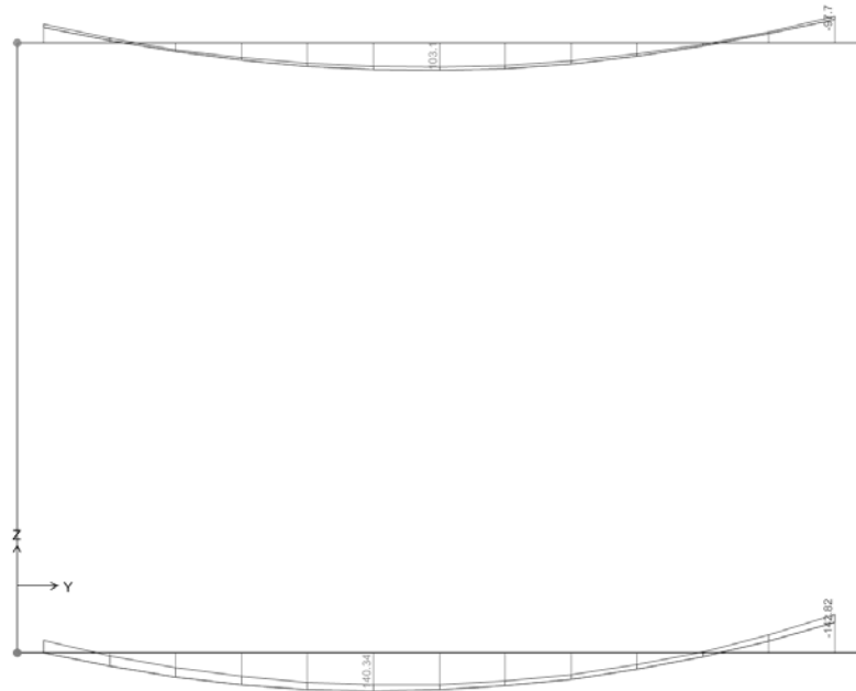
Figura 7-8 Diagramma dei momenti M3 – COMB_INV_SLU – allineamento 1.
