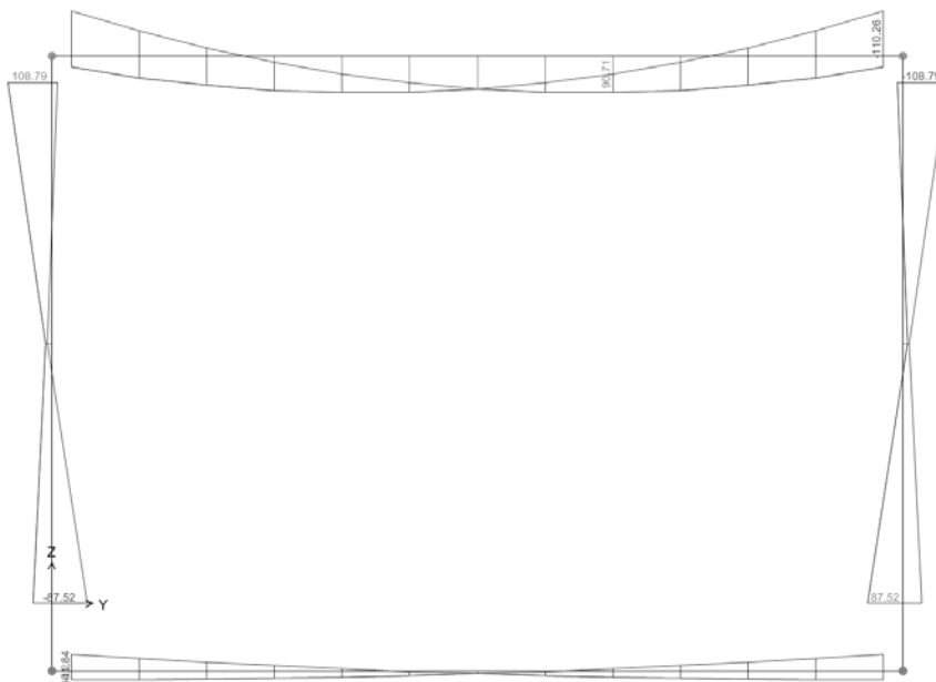
Figura 7-11 Diagramma dei momenti M3 – COMB_INV_SLV – allineamento 2.
