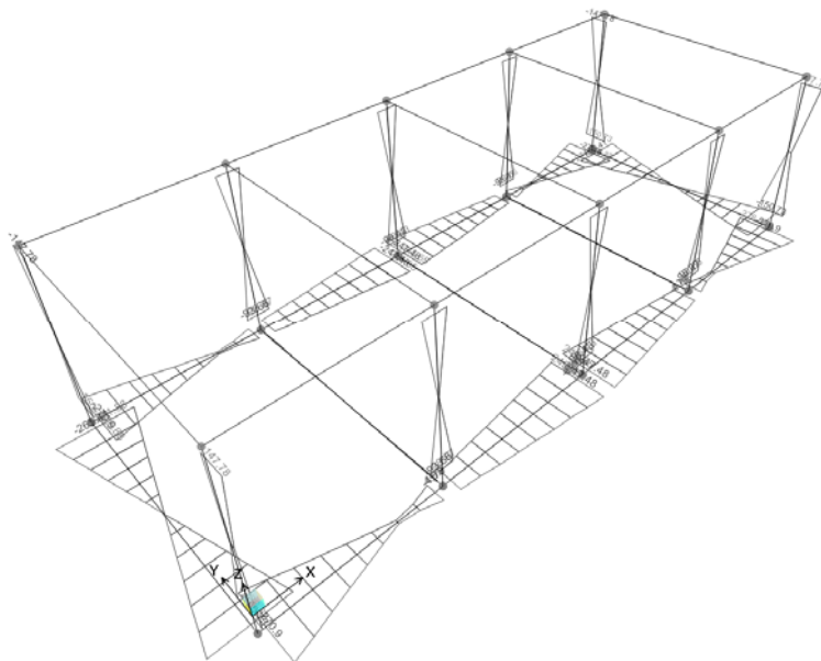
Figura 7-12 Diagramma dei momenti M2 – COMB_INV_SLU.
