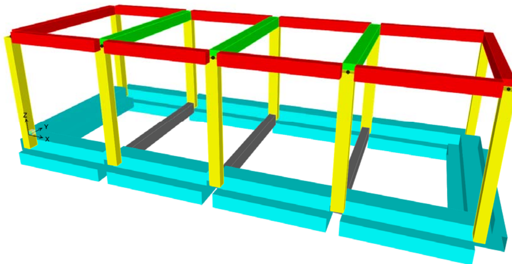
Figura 7-1 - Vista estrusa del modello.
