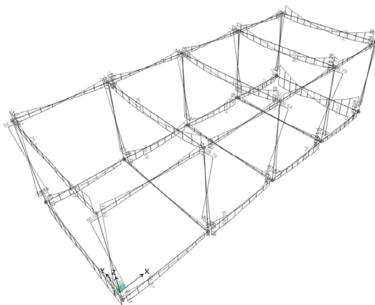
Figura 7-13 Diagramma dei momenti M3 – COMB_INV_SLV.
