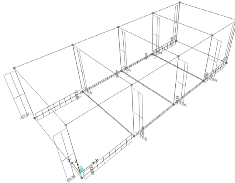
Figura 7-16 Diagramma dello sforzo assiale P – COMB_INV_SLU.
