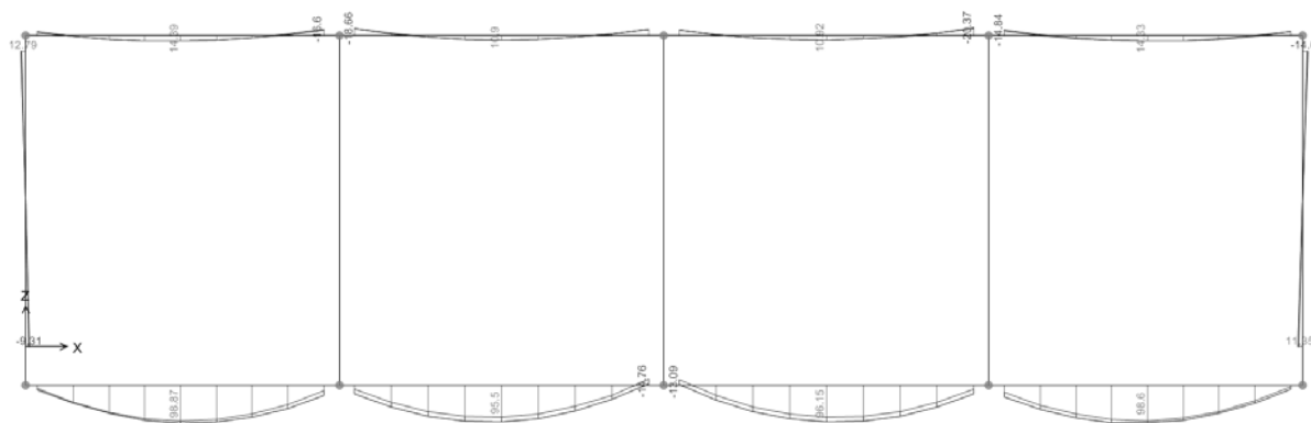
Figura 7-5 Diagramma dei momenti M3 - COMB_INV_SLV – allineamento B.
