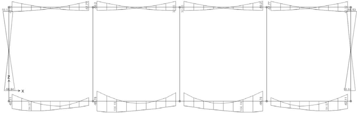
Figura 7-6 Diagramma dei momenti M3 - COMB_INV_SLU
