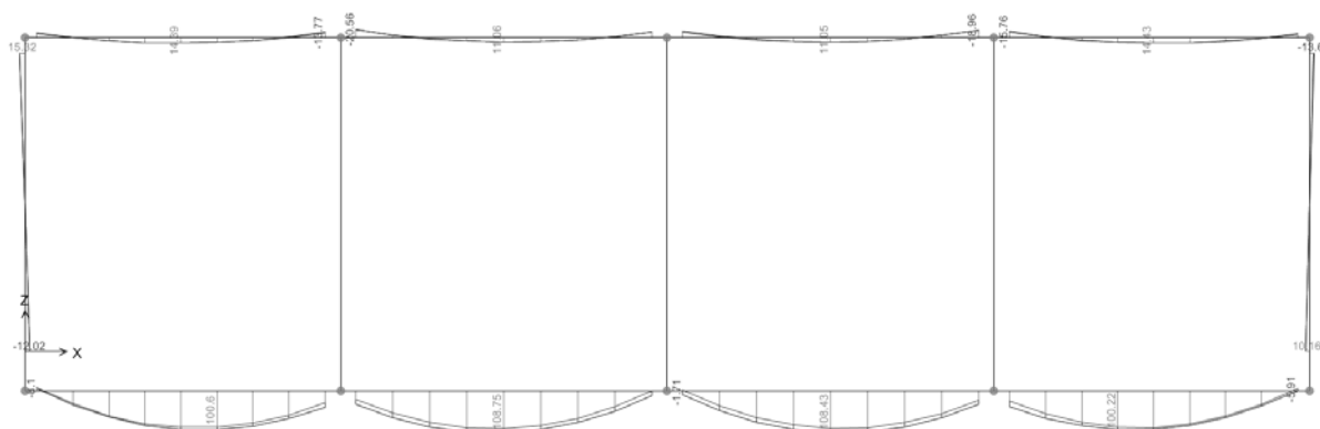
Figura 7-4 Diagramma dei momenti M3 – COMB_INV_SLU – allineamento A.
