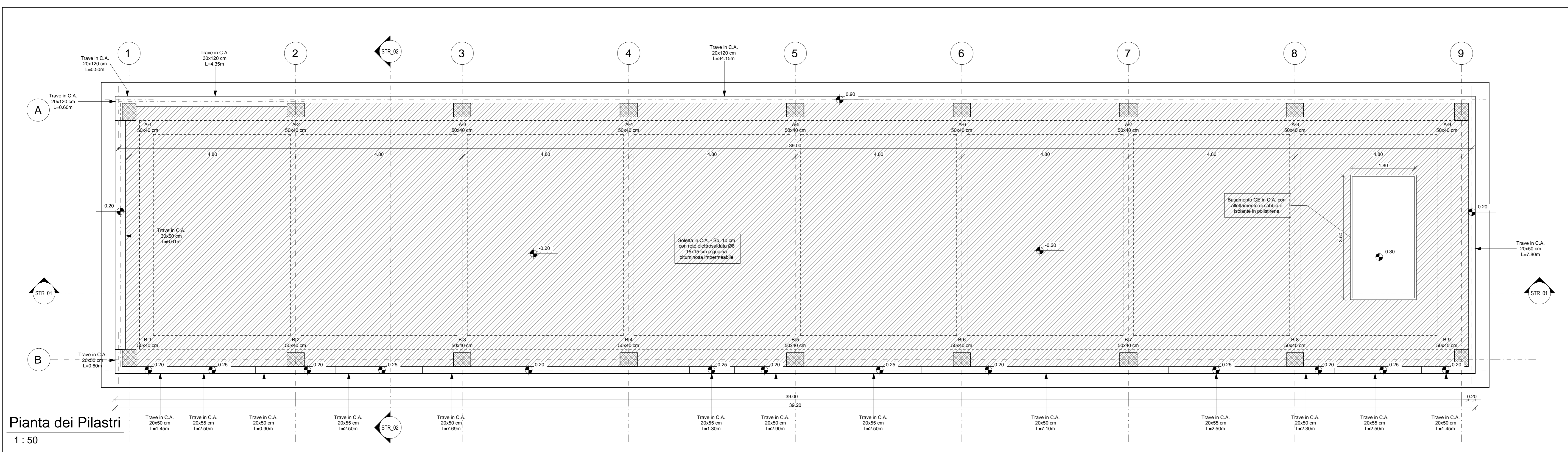
Pianta Fondazioni 1 : 50
