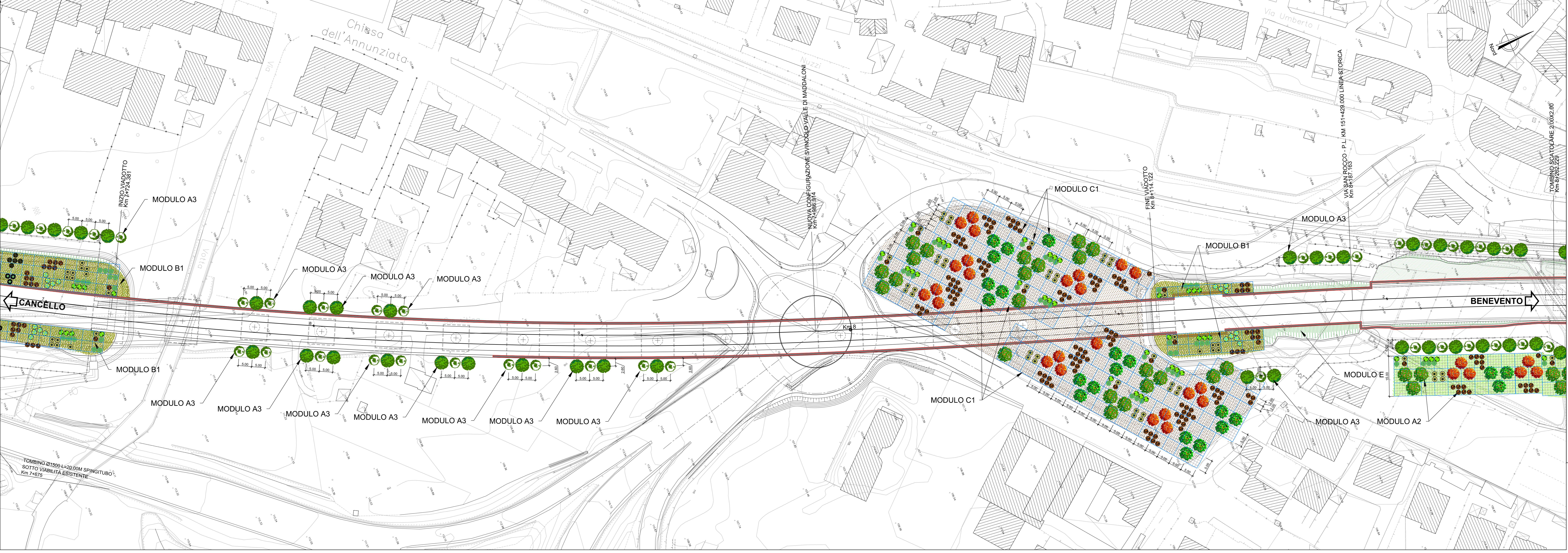
PLANIMETRIA DI DETTAGLIO OPERE A VERDE AREA VIADOTTO KM 8+639 - SCALA 1:500
