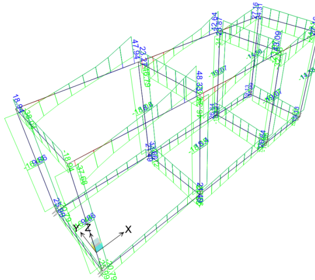
Figura 6-28 Diagramma del taglio V2 – COMB_INV_SLU.
