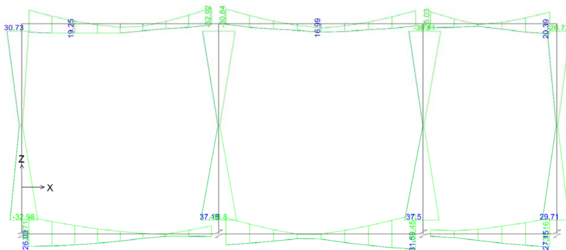
Figura 6-20 Diagramma dei momenti M3 – COMB_INV_SLU – allineamento A.
