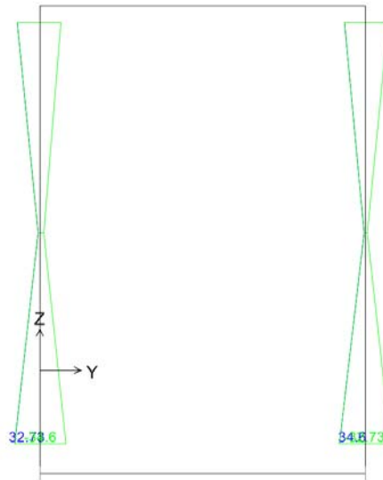
Figura 6-24 Diagramma dei momenti M3 – COMB_INV_SLU – allineamento 3.
