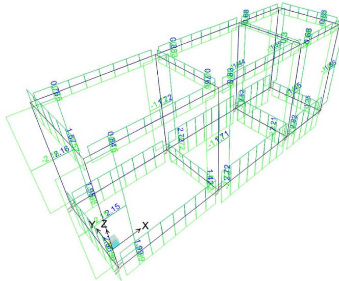
Figura 6-31 Diagramma della torsione T– COMB_INV_SLU.
