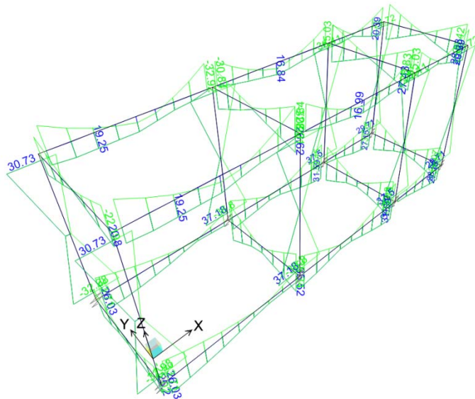
Figura 6-27 Diagramma dei momenti M3 – COMB_INV_SLU.
