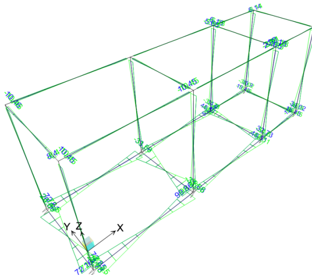
Figura 6-26 Diagramma dei momenti M2 – COMB_INV_SLU.
