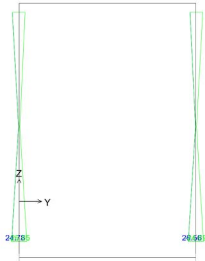
Figura 6-22 Diagramma dei momenti M3 – COMB_INV_SLU – allineamento 1.
