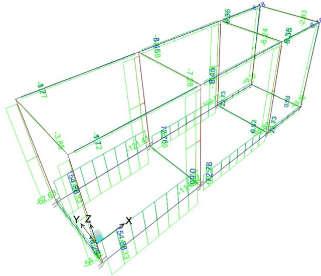
Figura 6-30 Diagramma dello sforzo assiale P – COMB_INV_SLU.
