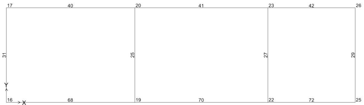
Figura 6-18 Numerazione frames e nodi piano copertura.
