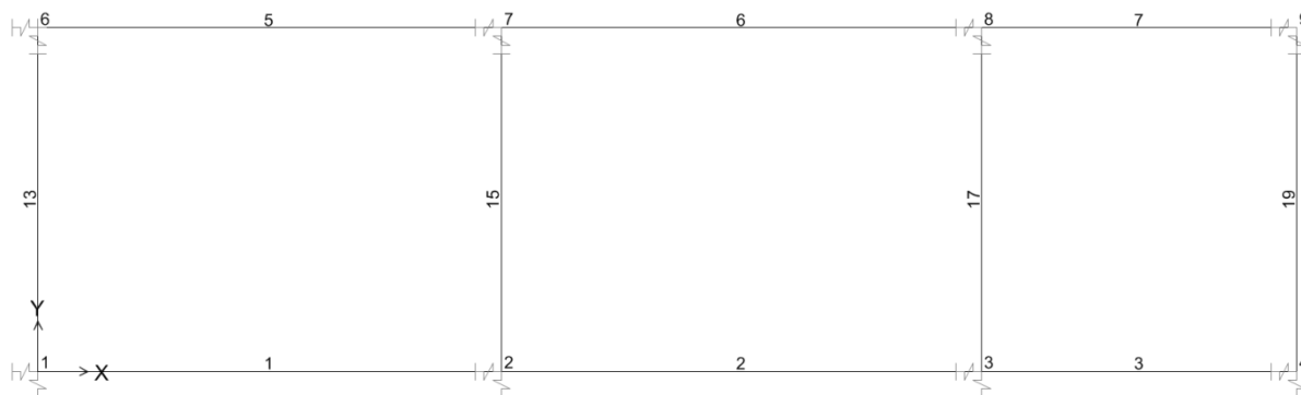
Figura 6-19 Modello di calcolo – numerazione frames e nodi piano fondazioni.
