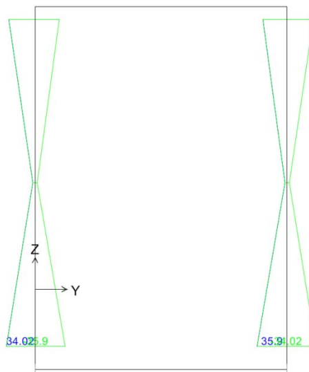
Figura 6-25 Diagramma dei momenti M3 – COMB_INV_SLU – allineamento 4.
